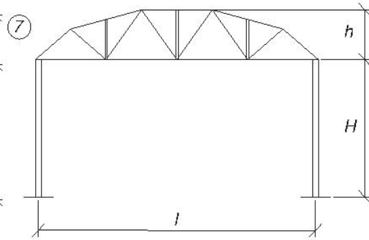
Ригель – багатокутна ферма; Стояк – дощатоклеєний
