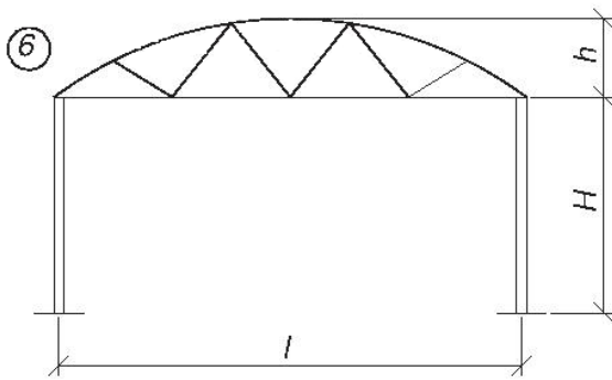
Ригель – ферма сегментна; стояк – клеєний, армований
