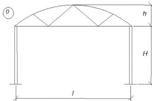
Ригель – ферма сегментна; стояк – дощатоклеєний
