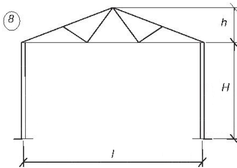
Ригель – трикутна ферма; стояк – дощатоклеєний
