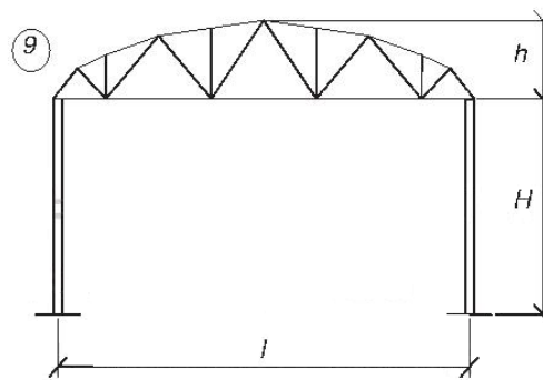
Ригель – багатокутна ферма; стояк – клеєний, армований
