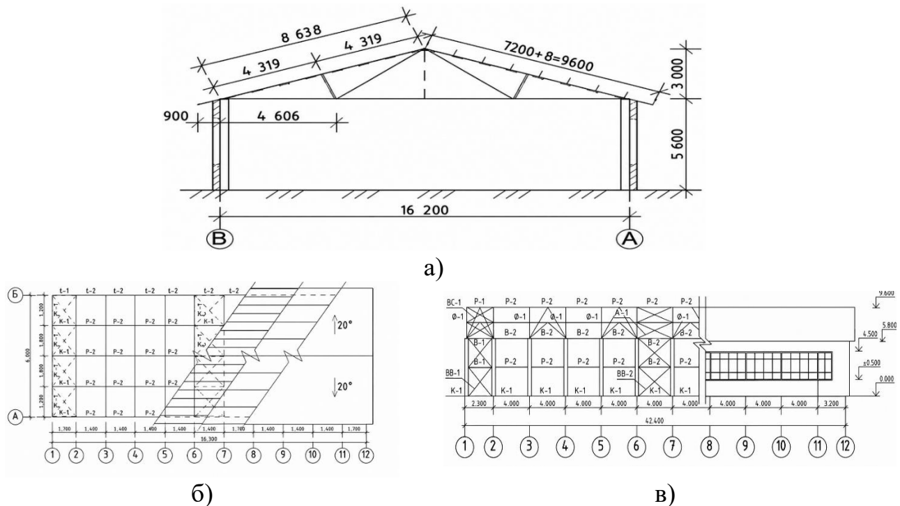
Рис. 2. Конструктивна схема будівлі: а) – поперечний розріз;
