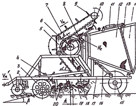
Рис. 1. Принципова схема трирядкової бункерної коренезбиральної машини
