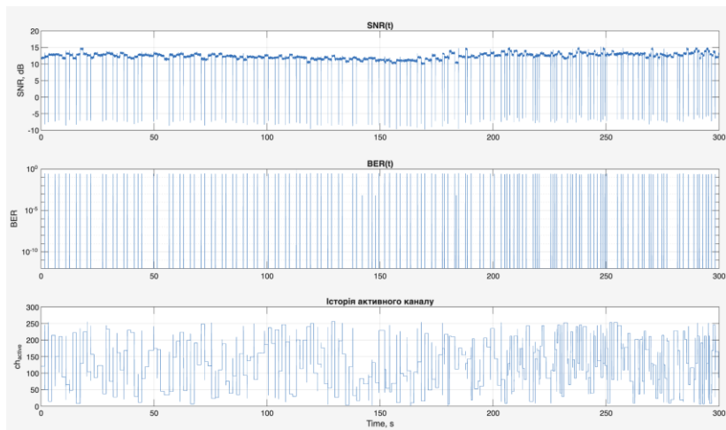
Рис. 2. Моделювання в середовищі MATLAB роботи захищеної системи передавання інформації
