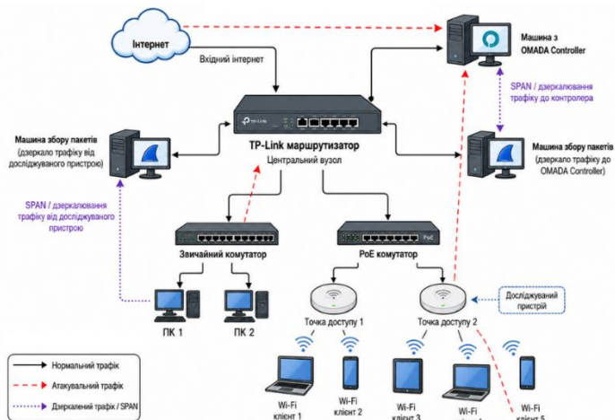
Рис.1. Схема дослідження трафіку та збору пакетів
