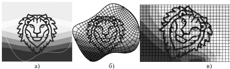
Рис. 1. Початкове зображення (а), сіткі фізичної області (б) та області комплексного потенціалу (в)
