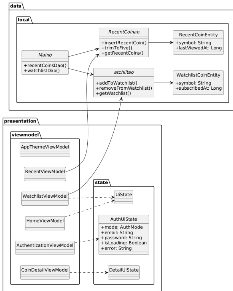
Рисунок 2.4 — Діаграма класів: локальне сховище та презентаційний шар
