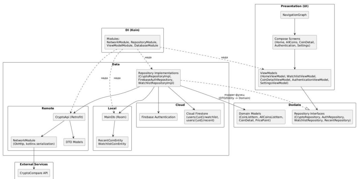
Рисунок 2.1 – Загальна архітектура програмної системи The Futures
