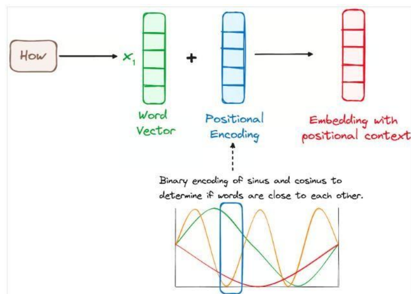
Рисунок 2.4 – Схематичне зображення позиційного кодування [27]
