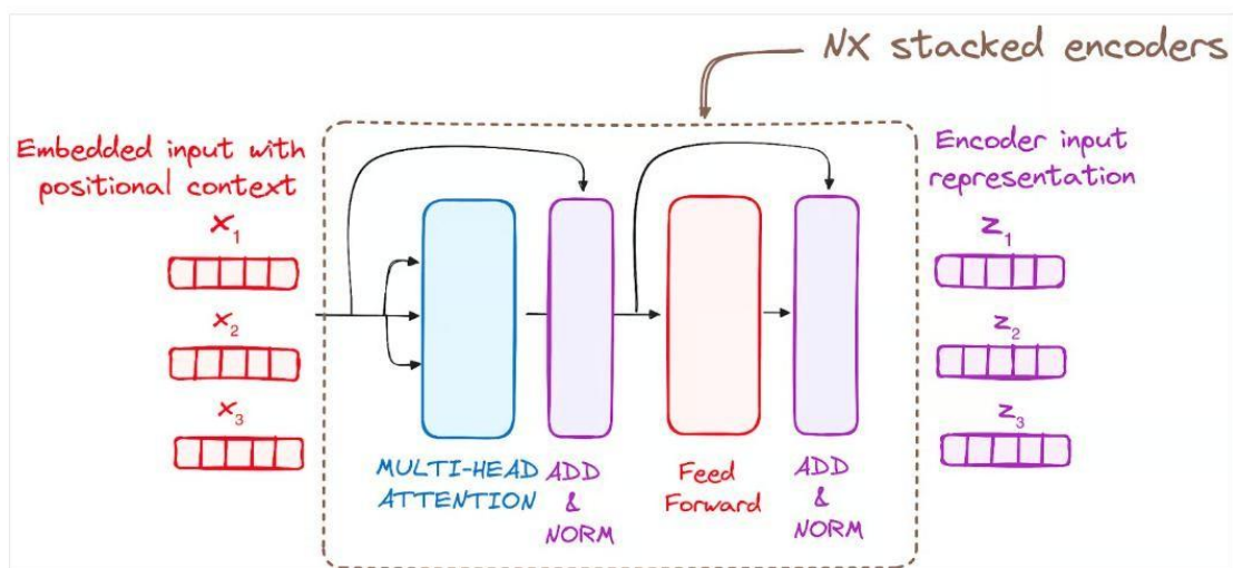
Рисунок 2.5 – Набір шарів енкодера [27]
