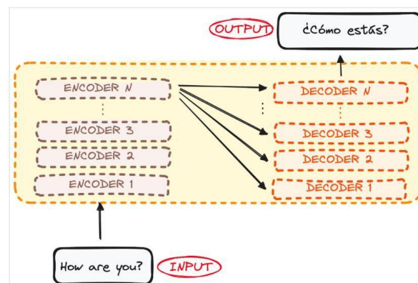
Рисунок 2.1 – Загальна структура архітектури Transformer “кодер–декодер” з N-шарами
