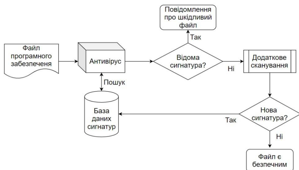
Рисунок 1.6 – Алгоритм роботи сигнатурного методу [22]
