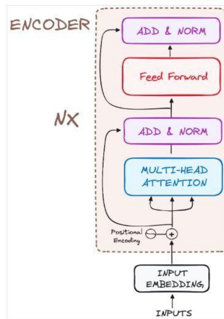
Рисунок 2.2 – Структура кодера [27]
