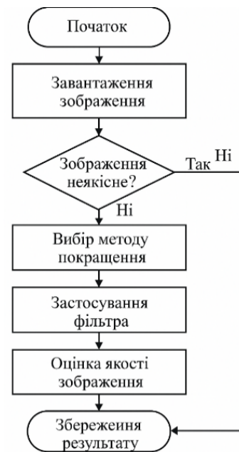
Рис. 1. Алгоритм побудови фільтраційної послідовності в системі компенсації завад
