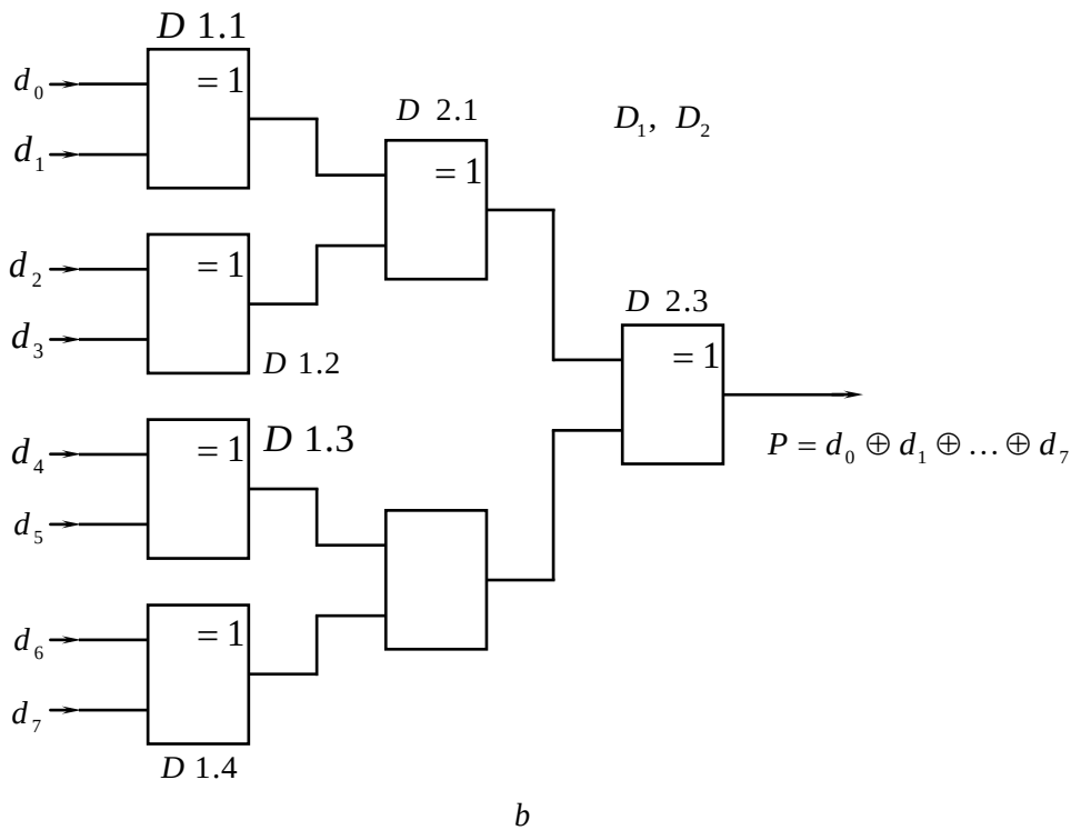
Рис. 3.1. Захист даних при передачі з допомогою перевірки на парність
