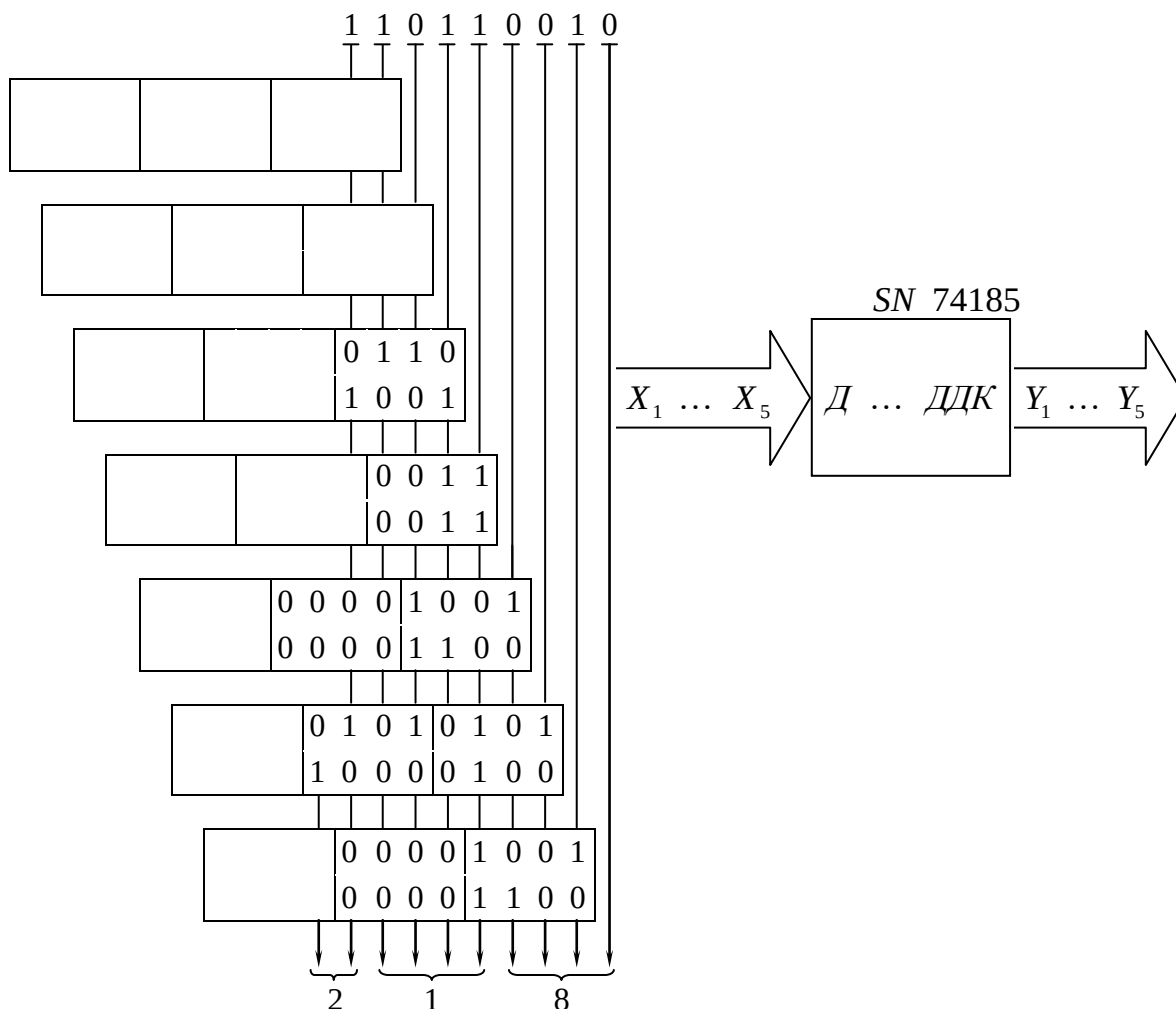
Рис. 2.3. Комбінаційні схеми перетворення коду.
