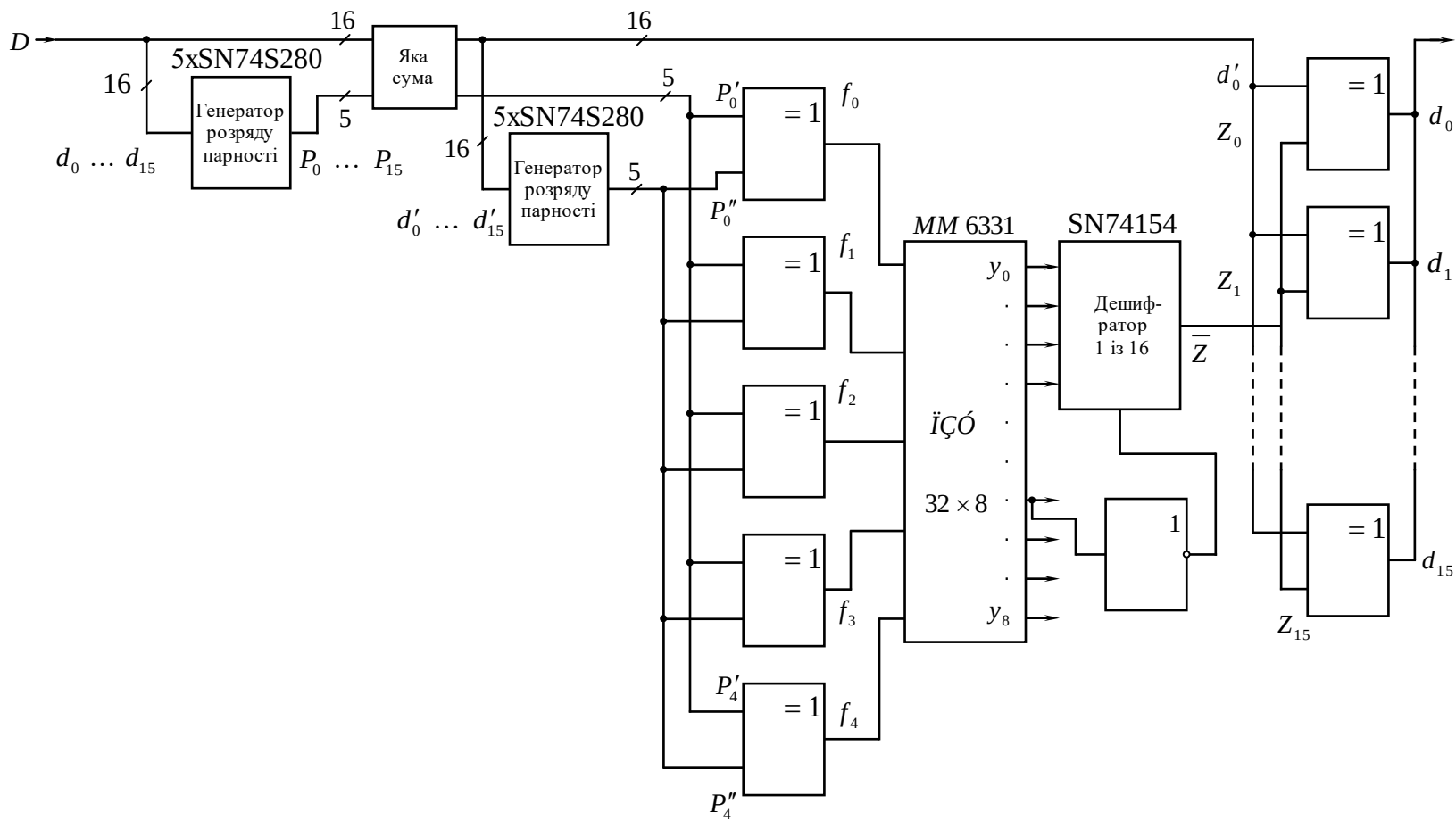
Рис. 6. Передача даних з корегуванням одиничної помилки.
