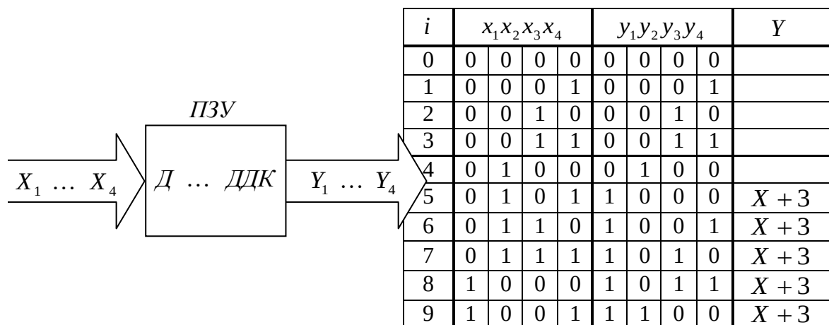
Рис. 2.2. Схемна реалізації перетворення кодів.
