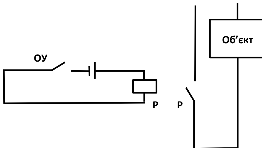
Рисунок 2 – Дистанційне управління об'єктом
