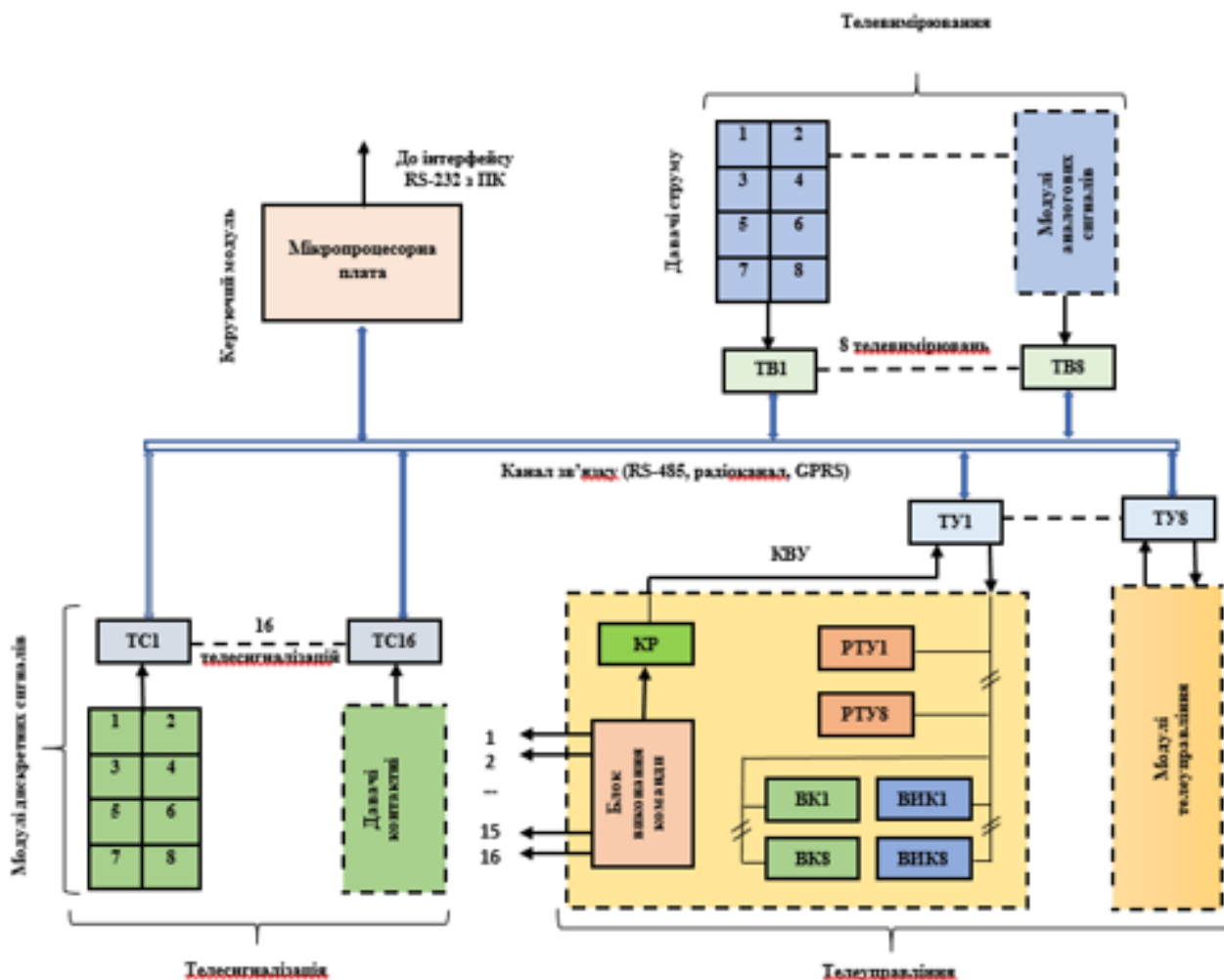
Рисунок 1. Комплекс мікропроцесорної телемеханіки (МТ):
