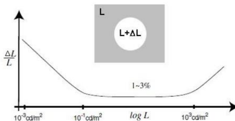
Рисунок 2.6 – Закон Вебера-Фехнера
