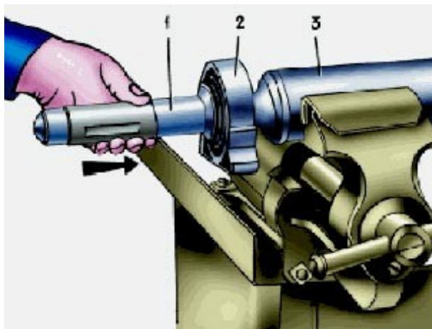
Рисунок 2.12 - Установка промежуточной опоры на передний карданный вал:
