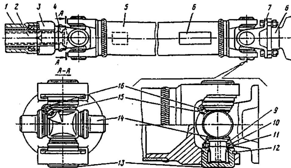
Рисунок 1.1 - Карданна передача:
