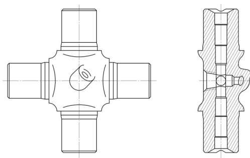
Рисунок 1.3 – Хрестовина 3102-2201030
