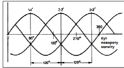
Рис. 3. Графік напруги трифазного генератора
