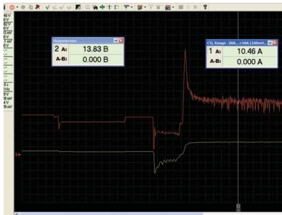
Рис.4. Осцилограма струму та напруги АКБ генератора зняті при запуску ДВЗ
