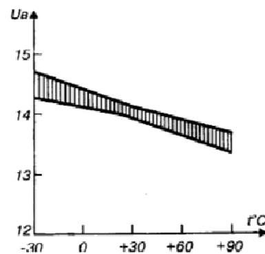
Рис.2. Температурна залежність напруги, яку підтримує регулятор при частоті обертання ротора 6000 хв -1 і силі струму 5А.
