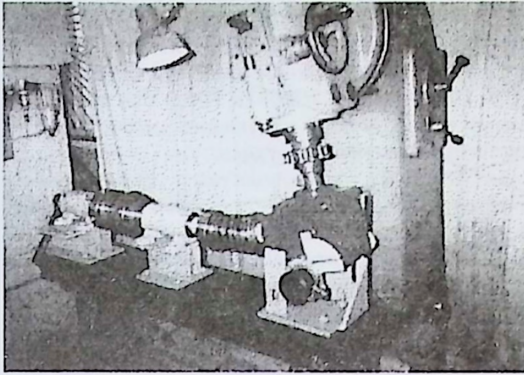
Рисунок 1 – Загальний вигляд стенда для дослідження запобіжно-компенсуючих муфт.
