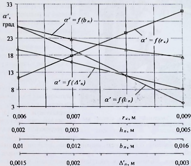
Рисунок 2 – Залежність зміни кута \alpha' зміщення півмуфт від конструктивних параметрів радіальної пари контакту пружина-кулька-паз.
