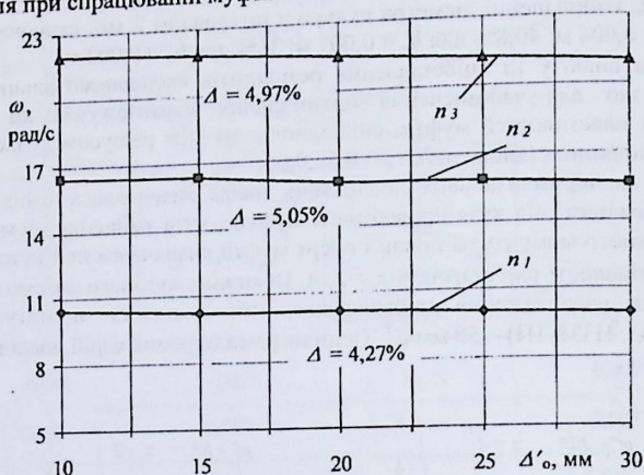
Рисунок 5 – Залежності впливу амортизуючої пружини на кутову швидкість муфти при наявності осьового зміщення: n_1 \approx 100 об/хв.; n_2 \approx 158 об/хв.; n_3 \approx 212 об/хв.
