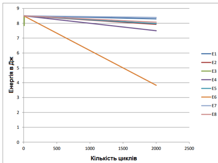
Рис. 3.8.Зміна енергії за 2000 циклів для восьми датчиків
