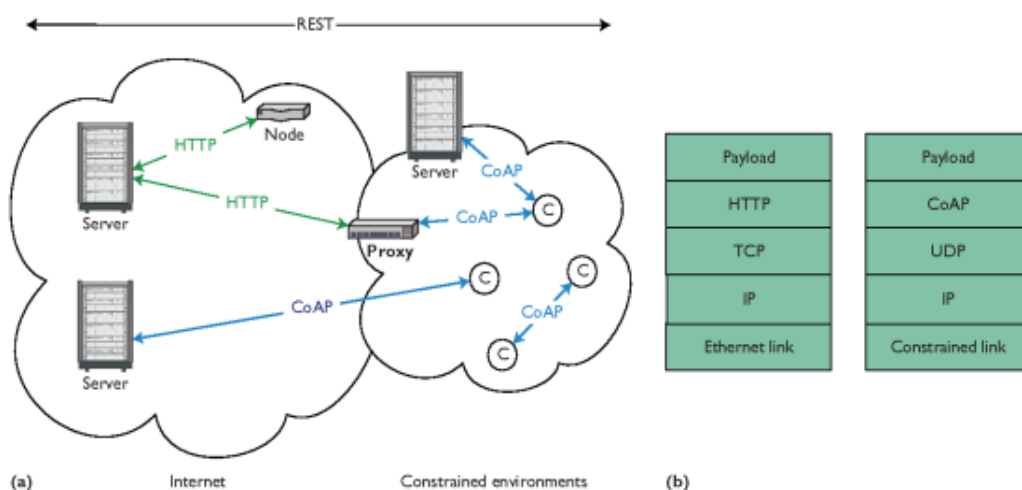
Рис. 2.3. Протокол CoAP
