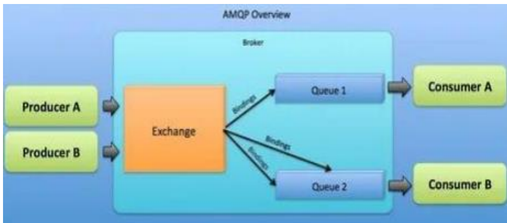
Рис. 2.5. Протокол AMQP
