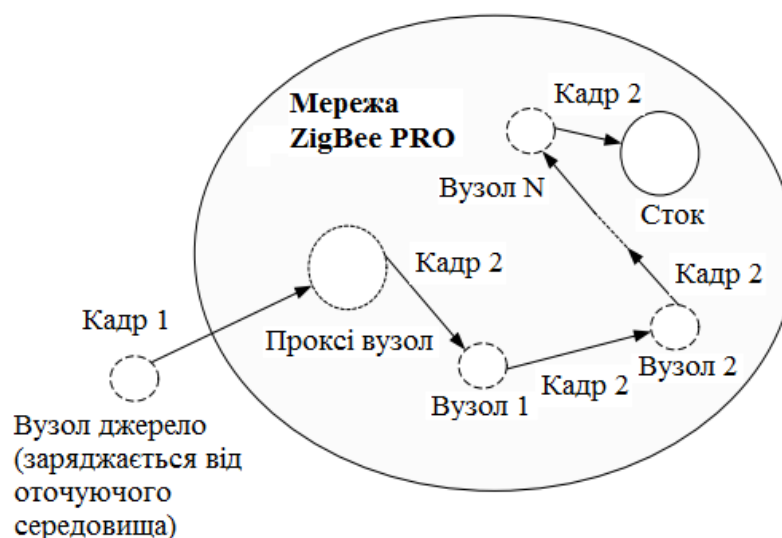
Рис. 1.3. Базовий механізм ZigBee GP
