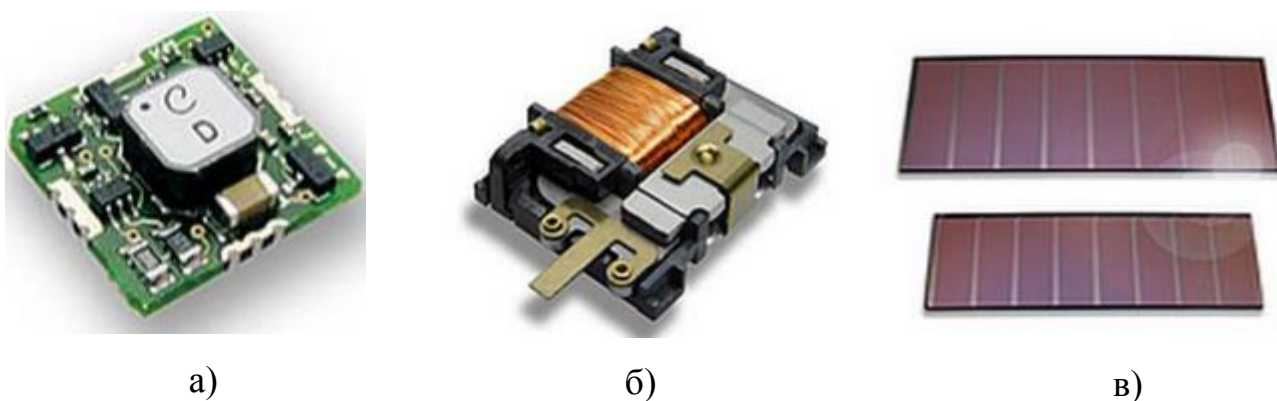
Рис. 1.2. Спеціалізовані модулі, котрі беруть енергію із навколишнього середовища (а - ECO 200 - Motion Energy Harvesting, б - ECT 310 Perpetuum - Thermo Energy Harvesting, в - ECS 300/ ECS 310 - Solar cells)
