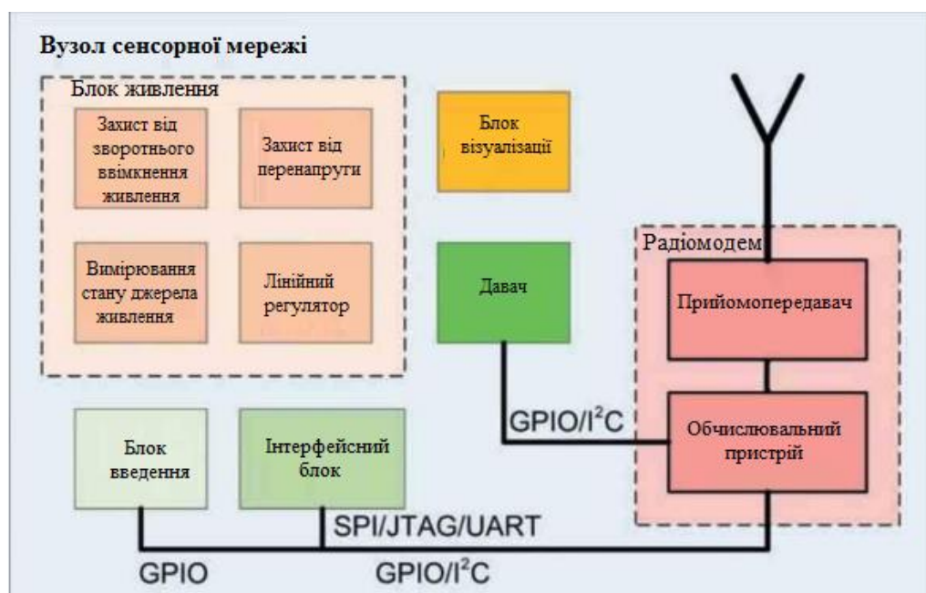
Рис. 2.1. Вузол БСМ
