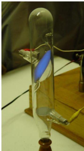
Фосфоресцентна лампа, конструкції Івана Пулюя
