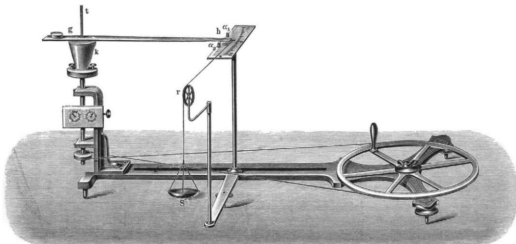
Прилад конструкції Івана Пулюя для вимірювання значення механічного еквіваленту теплоти
