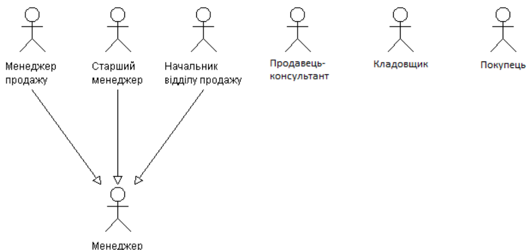
Рисунок 3 - Актори системи
