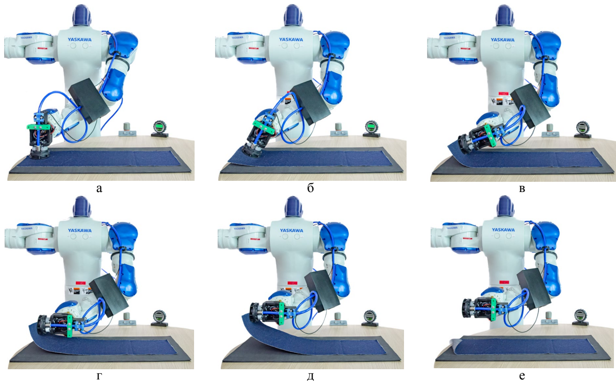
Рис. 2. Втрата контакту із гнучким об'єктом під час маніпулювання: (а) захоплення; (б) переорієнтація; (в) переорієнтація; (г) початок підняття; (д) підняття; (е) втрата контакту і падіння.
