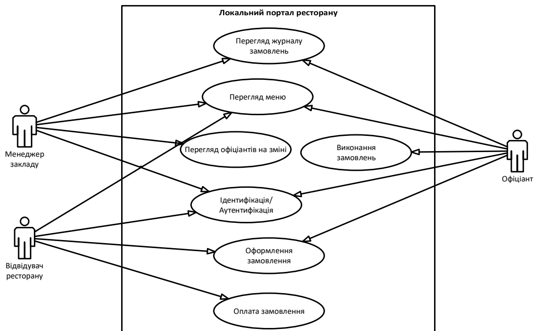
Рис. 1. Діаграма варіантів використання локального порталу розподіленої системи управління приватними ресторанами
