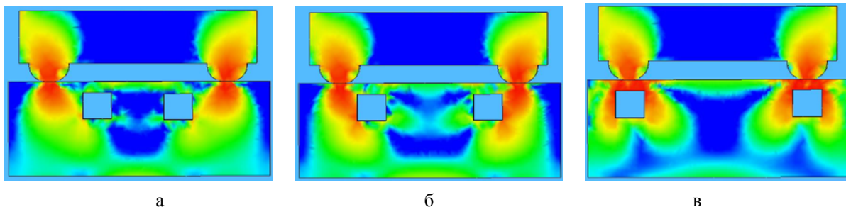
Рисунок 3 – Характерні епюри напруження в зоні контакту поверхонь зразків (деталей) при різній відстані розташування наповнювачів кубічної форми: а – \lambda_1 ; б – \lambda_2 ; в – \lambda_3 ; \lambda_1 < \lambda_2 < \lambda_3
