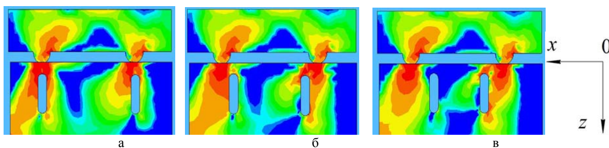
Рисунок 6 – Характерні епюри напруження в зоні контакту трибоспрязження зразків з частинками наповнювача циліндричної форми у поверхневому шарі при терті \bar{v} \neq 0 : в контактній (а) та міжконтактній (б, в) областях
