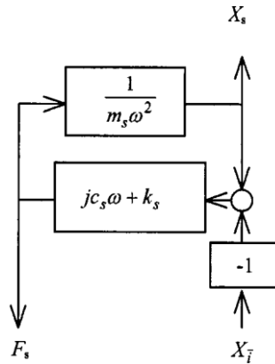
Рисунок 3. Двостороння модель графа стану вторинної системи
