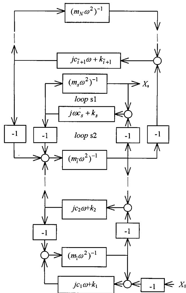
Рисунок 4. Графічний режим роботи обладнання та первинної структури
