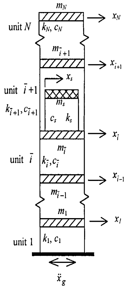
Рисунок 1. Принципова схема обладнання, приєднаного до багатопверхового будинку
