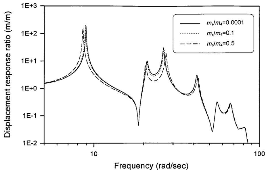
Рисунок 6. Коефіцієнт відгуку обладнання на 4 поверсі, \Omega_s/\Omega_4 = 0,5 , \xi_s = 0,012
