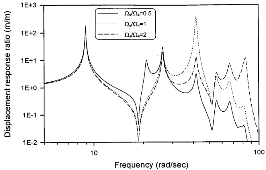
Рисунок 5. Коефіцієнт відгуку обладнання на поверхсі 4, m_s/m_4 = 0,01 , \zeta_s = 0,012
