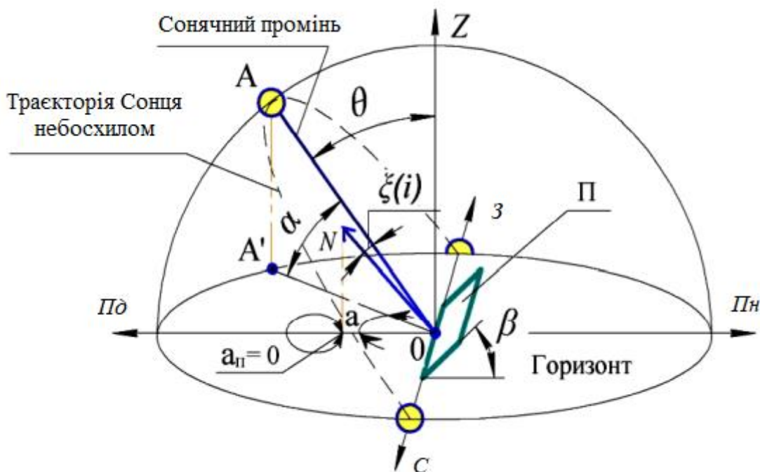
Рисунок 1.5 – Просторова орієнтація наземних сонячних установок відносно Сонця: Пд, Пн, С, З – сторони світу; А - положення Сонця на небосхилі; а - азимут Сонця; \theta – кут зеніту, \alpha – кут висоти Сонця; П – поверхня сонячної установки; N – нормаль до поверхні; a_n - азимут поверхні; \xi(i) – кут між нормаллю та напрямом на Сонце; \beta – кут нахилу
