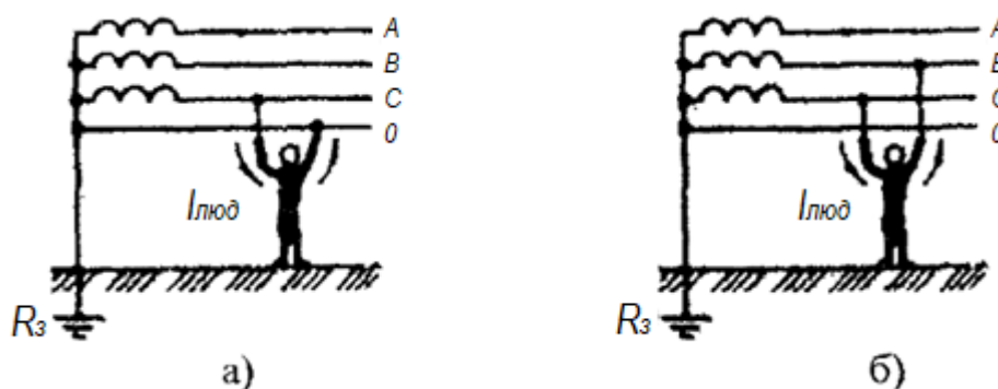
Рисунок 4.2 - Двополіусний дотик до мережі з глухозаземленою нейтраллю
