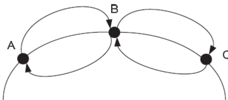
Рисунок 3.6 – Траєкторія руху робочої точки на вольт-ватній характеристиці сонячних панелей в околі точки максимуму
