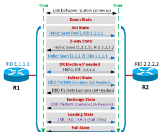
Рис 1.3. Процес встановлення сусідства за OSPF
