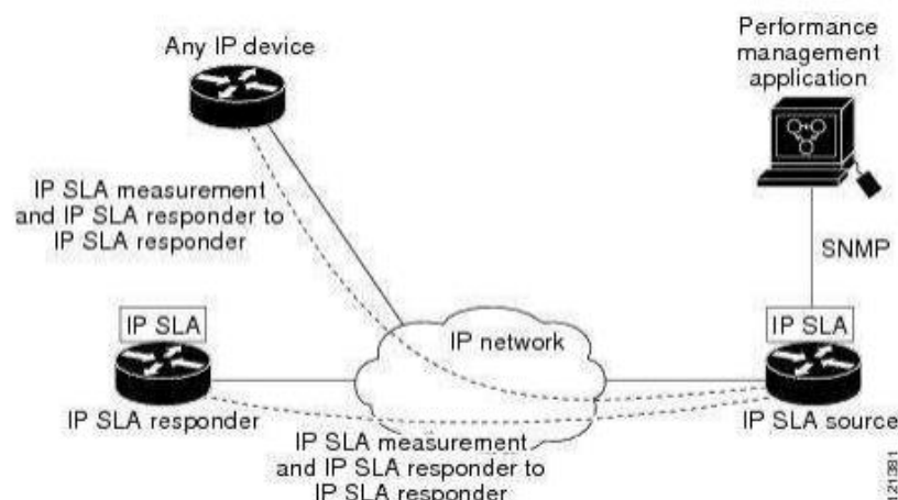
Рис. 1.4. Операції IP SLA
