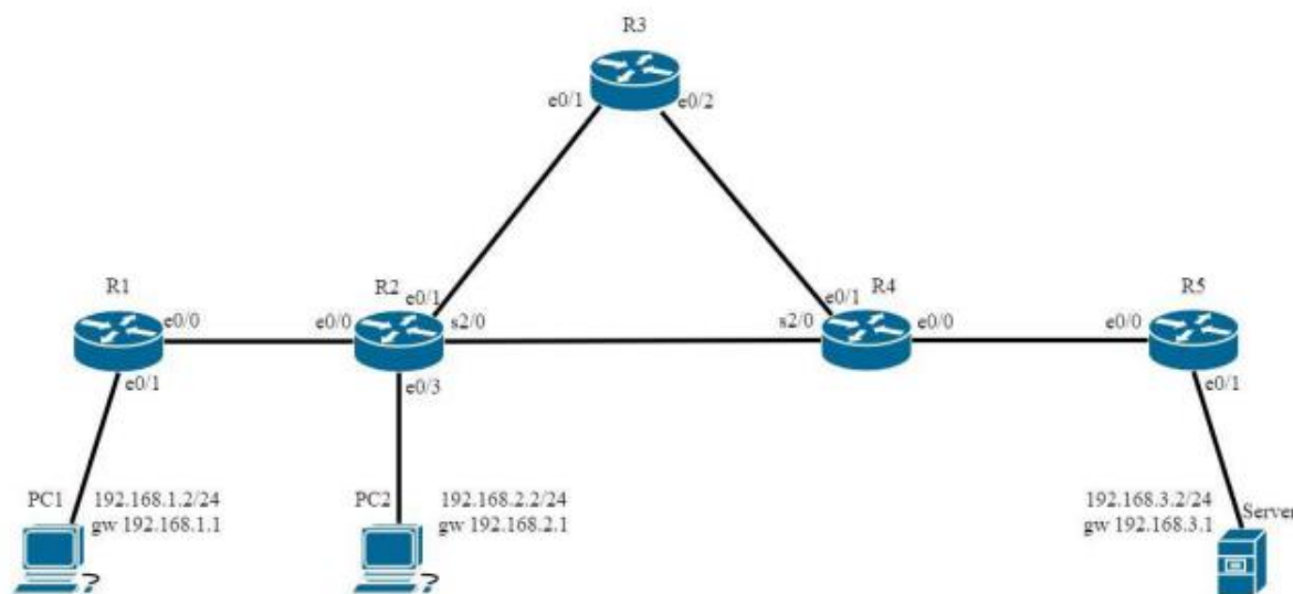
Рис. 3.1. Лабораторний стенд
