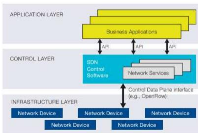
Рис. 1.6. Архітектура SDN
