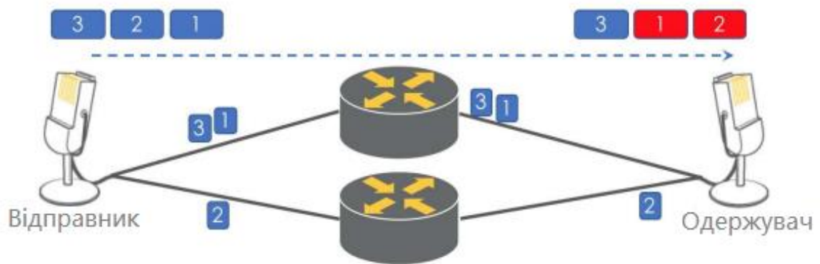
Рис. 2.6. Невпорядкована доставка пакетів
