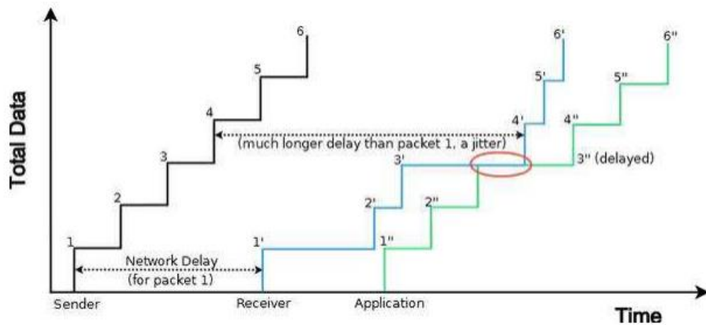
Рис. 2.5. Ілюстрація джитера при відправці пакетів
