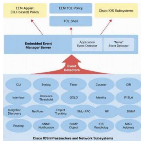
Рис. 1.5. Архітектура ЕЕМ
