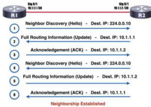
Рис. 1.2. Встановлення сусідства по протоколу EIGRP
