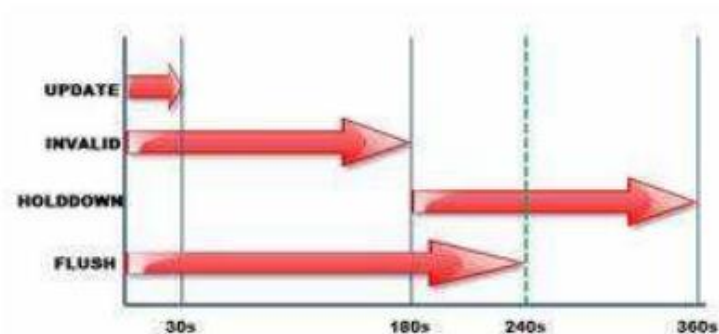
Рис. 1.1. Таймери протоколу RIP
