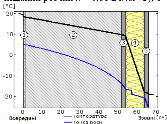
Рисунок 1. Розподіл температури в стіні за наявності утеплювача
