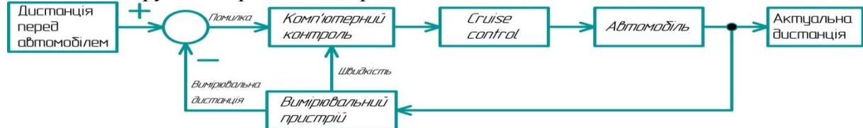
Рисунок 1. Структурна схема підсистеми керування мехатронною системою
