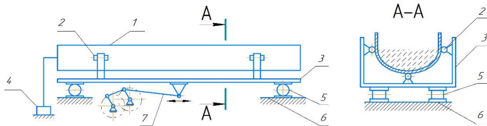
Рисунок 1. Інерційний конвеєр
