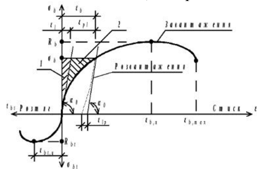
Рисунок 1. Залежність між напруженнями та деформаціями в бетоні:
