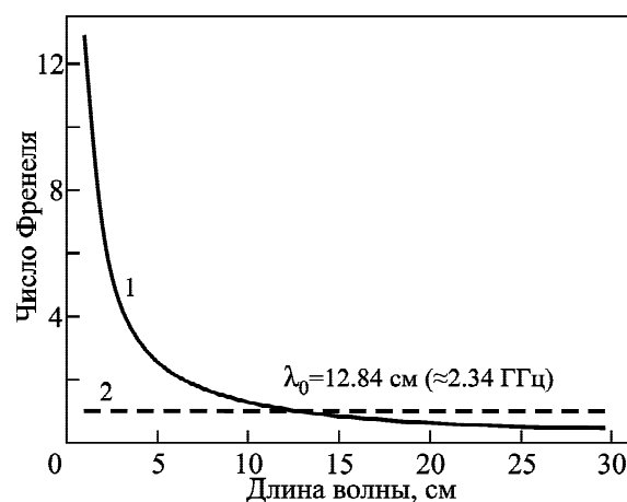
Рис. 5. Зависимость числа Френеля от длины волны для антенной системы MARK-4B (линия 1). Линией 2 показан уровень, где число Френеля равно 1.0. Значение \lambda_0 на графике показывает при какой длине волны (частоте) число Френеля для антенной системы MARK-4B равно 1.0
