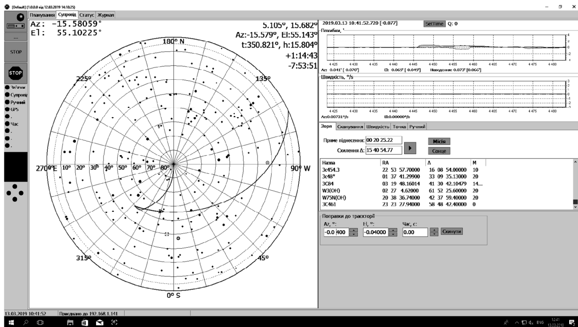
Рис. 17. Эфемериды радиостанции ЗС9 (ЗС26 FK5). В правом верхнем углу изображены эпюры распределения скоростей движения зеркала радиотелескопа РТ-32 по азимуту и углу места
