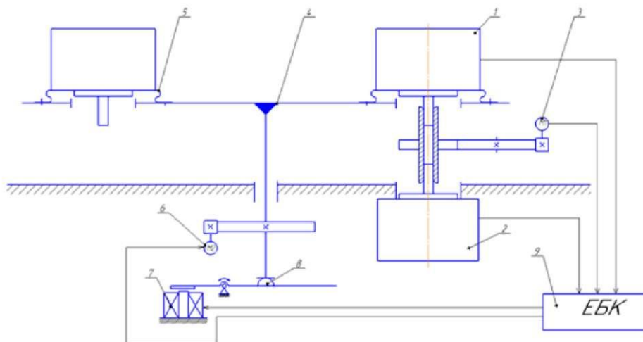
Рис. 1. Функціональна схема стану для перевірки еncoderів
