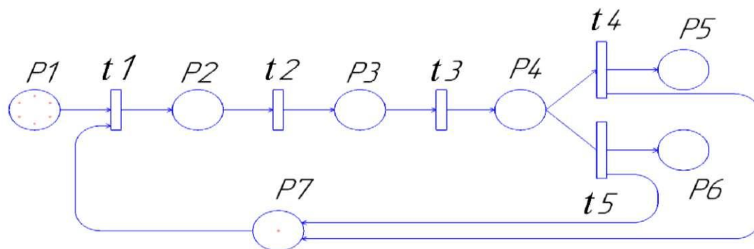
Рис. 2. Стохастична мережа Петрі для імітації роботи стану для перевірки енкодерів
