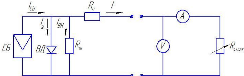
Рис. 1. Еквівалентна схема сонячного модуля
