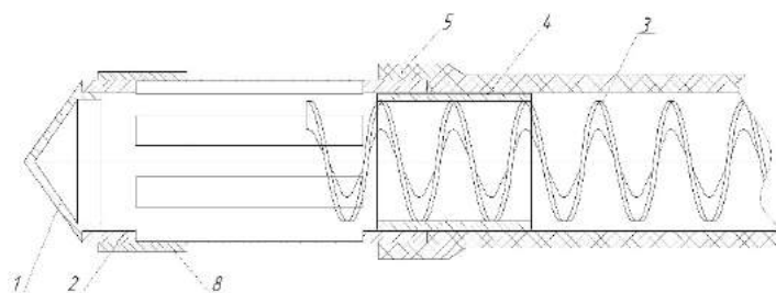
Рис. 8 - Завантажувально-захисна насадка гвинтового конвєсера з регулюванням процесу завантаження
