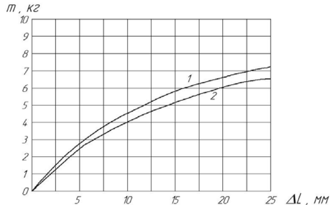
Рис. 7 - Залежність величини відносного видовження шнекової спіралі \Delta L від маси підвішеного вантажу m при зовнішньому діаметрі спіралі: 1 - D_1 = 68 мм; 2 - D_2 = 98 мм
