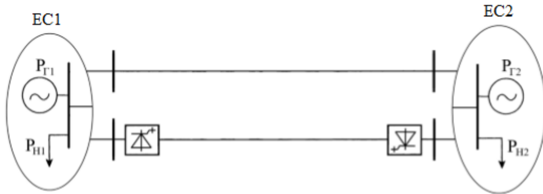
Рисунок 1. Керований перетин, що містить гнучку лінію постійного струму
