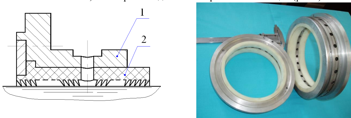
Рисунок 1 – Конструкція пластмасо-металевого лабіринтного ущільнення відцентрового нагнітача фірми «Нуово Піньоне» ГТК-25I
