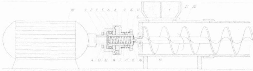
Рис. 2. Гвинтовий конвеєр обладнаний пружно-запобіжною муфтою
