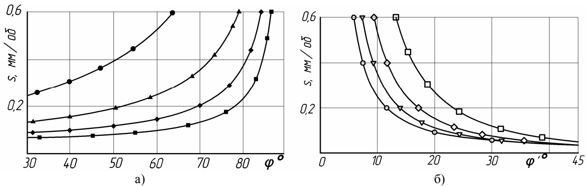
Рисунок 3. Графіки залежностей s БРГ від \varphi та \varphi' при H = \text{const} : а) s = f(\varphi) при різних значеннях \varphi' : ●—●—●— \varphi' = 10^\circ ; ▲—▲—▲— \varphi' = 15^\circ ; ◆—◆—◆— \varphi' = 20^\circ ; ■—■—■— \varphi' = 25^\circ ; б) s = \psi(\varphi') при різних значеннях \varphi : ○—○—○— \varphi = 30^\circ ; ▽—▽—▽— \varphi = 45^\circ ; ◇—◇—◇— \varphi = 60^\circ ; □—□—□— \varphi = 75^\circ
