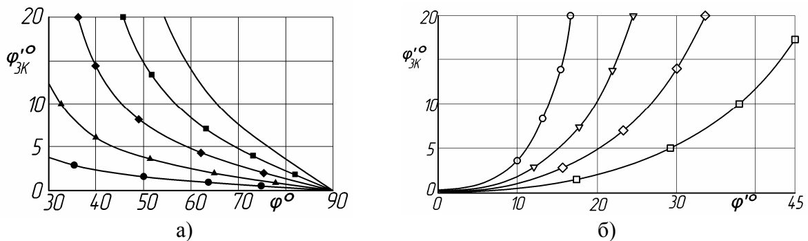
Рисунок 8. Графіки залежностей скорегованого допоміжного кута в плані ТЧР від значень головного та допоміжного кутів у плані: \varphi'_{3K} = \rho(\varphi) при різних \varphi' : \bullet — \varphi' = 10^\circ ; \blacktriangle — \varphi' = 15^\circ ; \blacklozenge — \varphi' = 20^\circ ; \blacksquare — \varphi' = 25^\circ — \text{—} — \varphi' = 30^\circ ; б) \varphi'_{3K} = \sigma(\varphi') при різних \varphi : \circ — \varphi = 30^\circ ; \nabla — \varphi = 45^\circ ; \diamond — \varphi = 60^\circ ; \square — \varphi = 75^\circ
