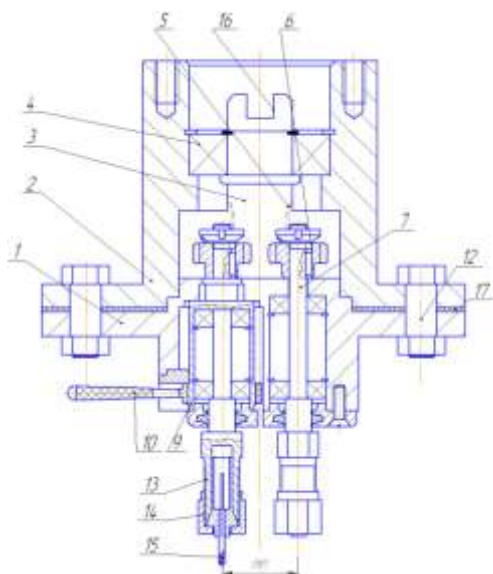
Рис. 1. Багатошпіндельна головка для обробки отворів (Патент України № 68202)
