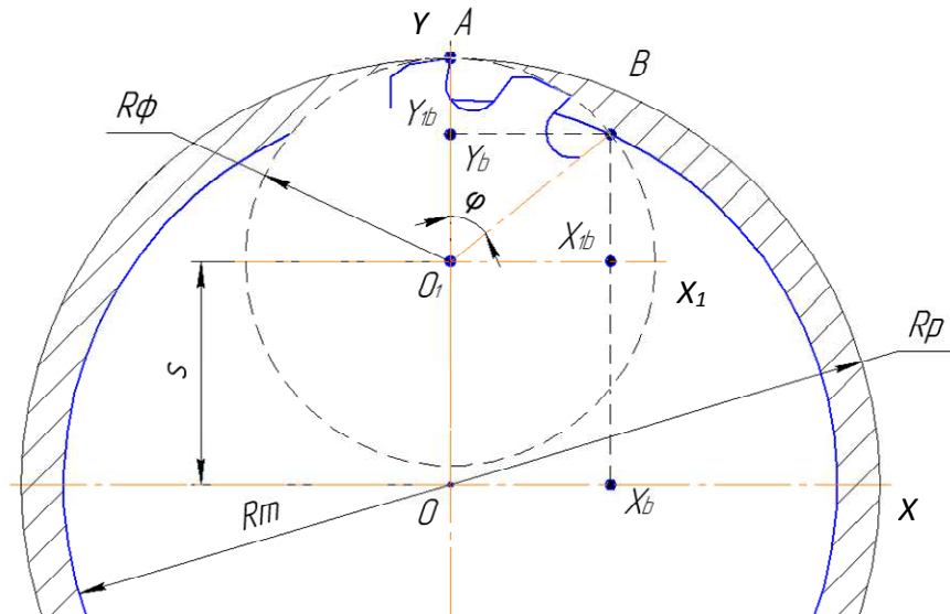
Рисунок 2. Розрахункова схема
