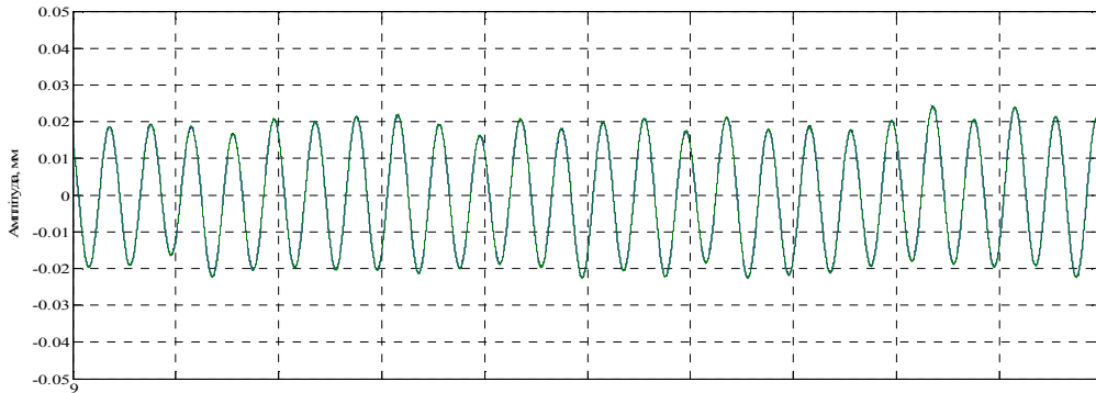
Рисунок 4. Запис коливань при напрузі живлення вібратора 140 В
