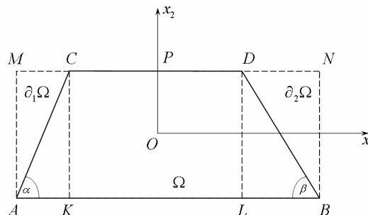
Рисунок 1. Схема трапецевидної плити
