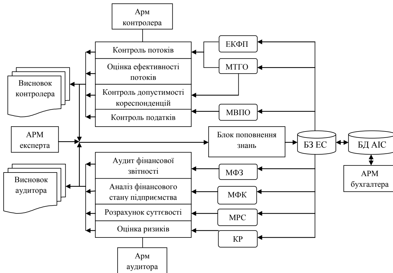
Рис. 5.2. Організація експертної системи
