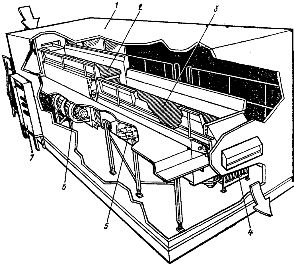
Рис. 15.6. Апарат флюїдаційний :
