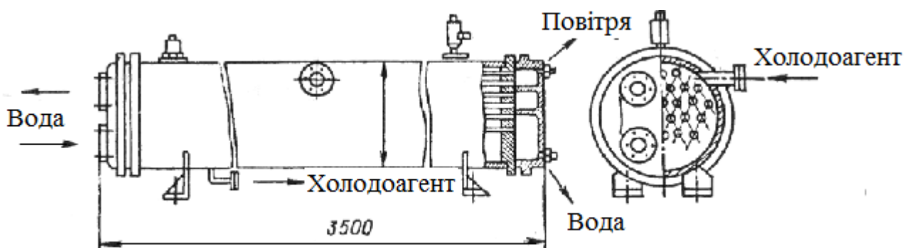
Рис. 5.2. Горизонтальний кожухотрубчастий хладоновий конденсатор
