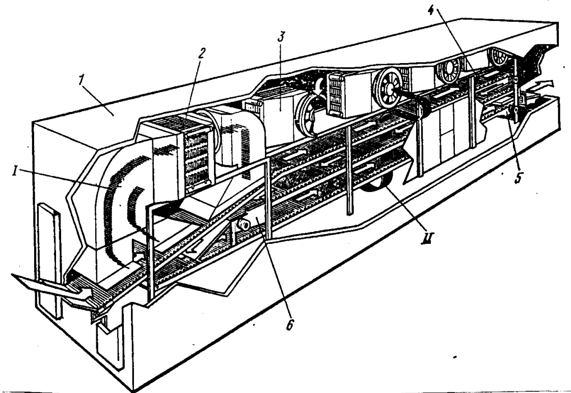
Рис. 15.3. Апарат з лінійними горизонтальними конвеєрами:
