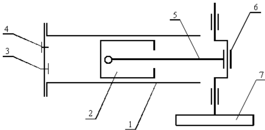
Рис. 4.2. Поршковий компресор
