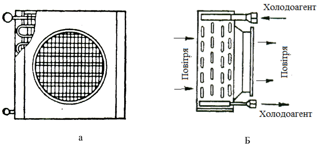
Рис.5.9. Повітряний фреоновий конденсатор (а). Повітряний конденсатор з зигзагоподібним розміщенням секцій (б).
