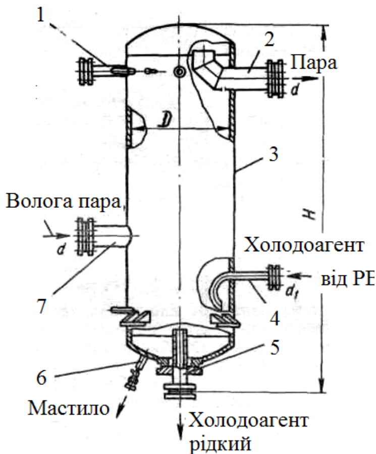
Рис.10.1. Віддільник рідини: 1 - патрубок приєднання до парової зрівняльної лінії; 2 - патрубок відведення пари до компресора; 3 - кожух; 4 - патрубок підведення холодоагенту від РЕ; 5 - патрубок зливання рідкого холодоагенту; 6 - вентиль відведення мастила; 7 - патрубок підведення вологої пари з випарника; H - висота ВР; d і d_1 - діаметри патрубків
