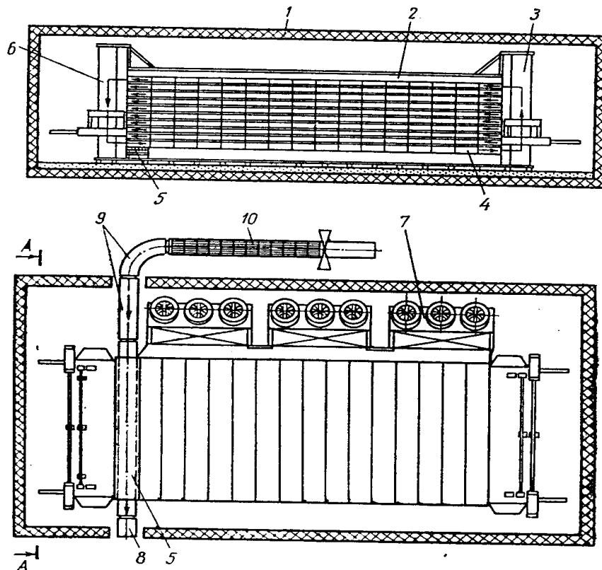
Рис.15.2. Апарат з циклічно рухомих конвеєром: 1–теплоізоляційна огорожа; 2 – стелаж; 3 – завантажувальний пристрій; 4 – каретки; 5 – рольганговий конвеєр; 6 – вивантажувальний пристрій; 7 – повітроохолоджувач; 8 – розвантажувальний конвеєр; 9 – завантажувальний конвеєр; 10 – накопичувальний конвеєр з рахунковим пристроєм
