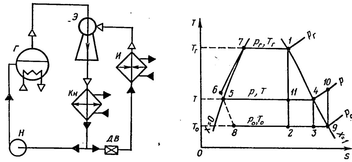
Рис.13.3. Функціональна схема водяної пароежекторної холодильної машини та її теоретичний цикл
