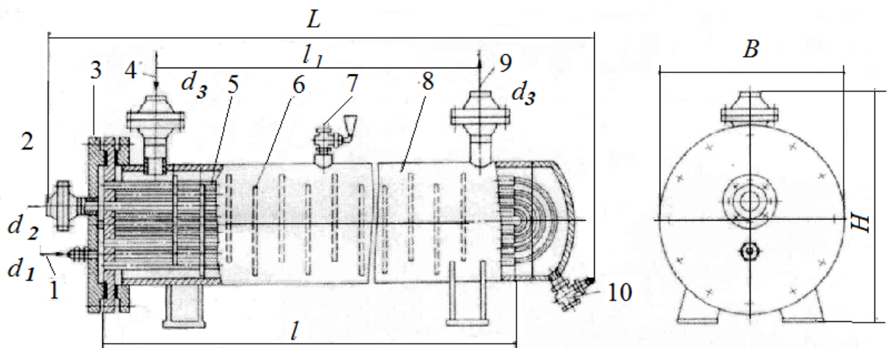
Рис. 6.5. Кожухотрубчастий випарник з внутрішнім кипінням холодоагенту в U-подібних трубах: 1,2 – підведення і відведення холодоагенту; 3 - кришка; 4, 9 – підведення і відведення розсолу; 5 - теплообмінні труби; 6 - поперечні перегородки для розсолу; 7 - кран для випуску повітря; 8 - обичайка; 10 - вентиль для зливу розсолу
