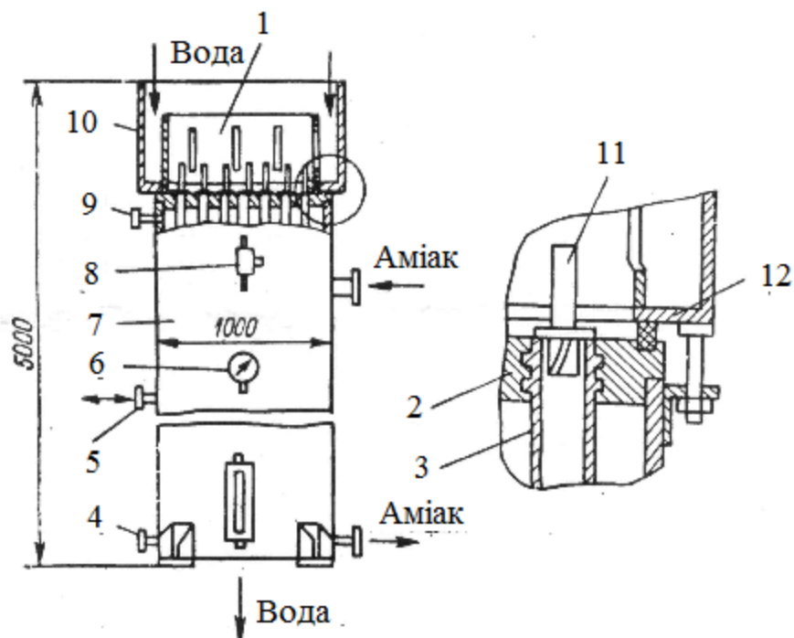
Рис. 5.4 - Вертикальний кожухотрубчастий конденсатор
