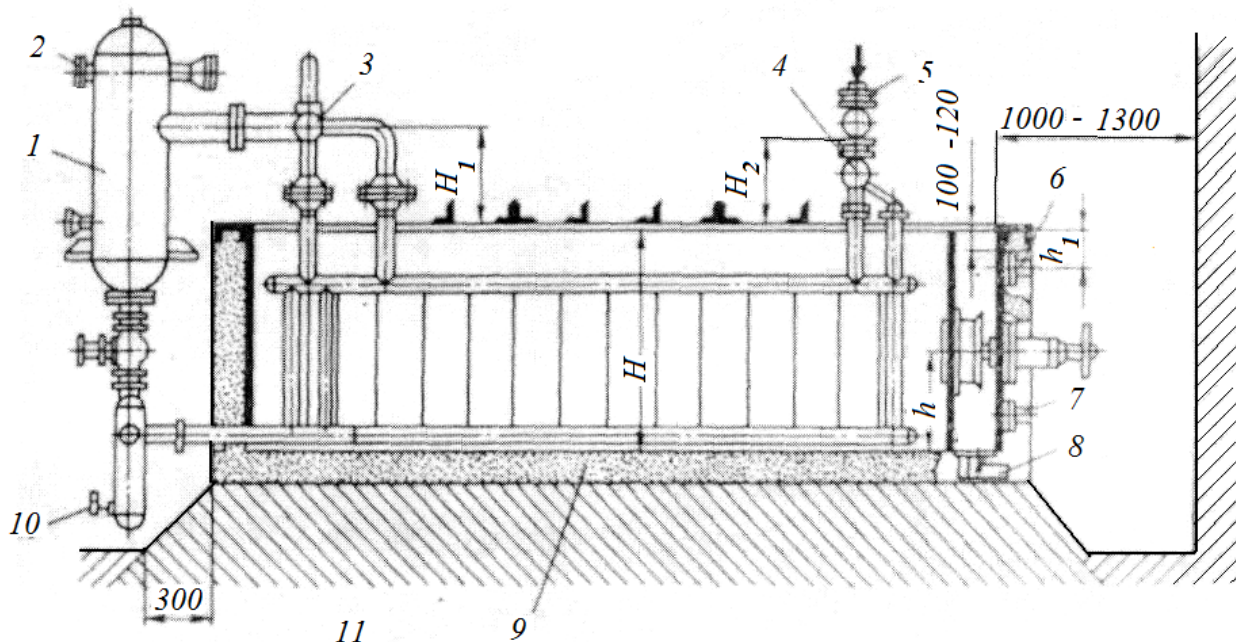
Рис.7. Панельний аміачний випарник ИП: 1 - віддільник рідини; 2 - патрубок для відведення парів аміаку; 3, 4 - збірний і розподільний колектори; 5 - патрубок для введення рідкого аміаку; 6 - перелив розсолу; 7 - патрубок для відведення розсолу; 8 – злив розсолу; 9 - ізоляція; 10 - вентиль для зливання мастила; 11 – запобіжний клапан
