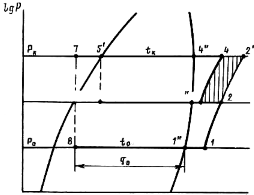
Рис.3.4. Зображення циклу парокомпресійної двоступеневої холодильної машини з повним проміжним охолодженням в діаграмі
