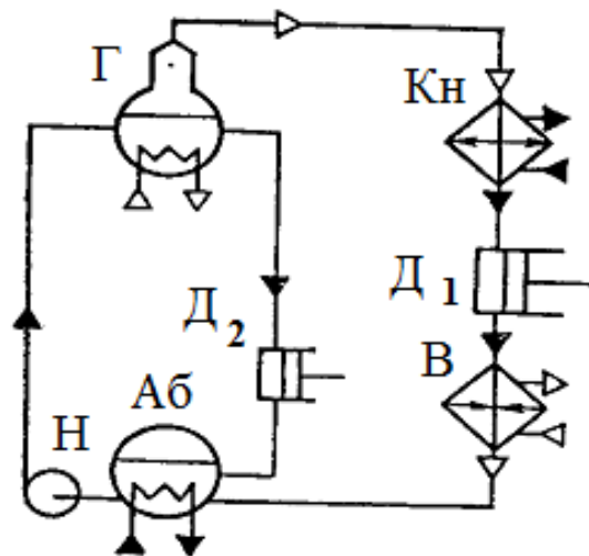
Рис.13.1. Функціональна схема найпростішої абсорбційної холодильної машини
