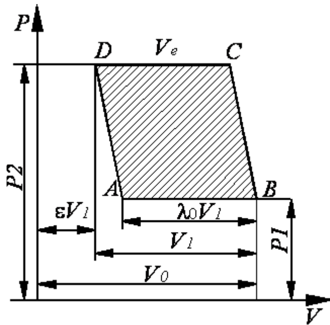
Рис. 4.3. Індикаторна діаграма
