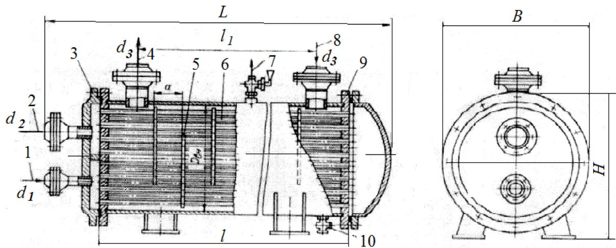
Рис.6.4. Кожухотрубчастий випарник з кипінням холодоагенту всередині прямих труб: 1,2- вхід і вихід холодоагенту; 3 - кришка; 4,8- вхід і вихід розсолу; 5 - поперечні перегородки для розсолу; 6 — теплообмінні труби; 7 — кран для спуску повітря; 9 - трубна дошка; 10 - вентиль для зливу розсолу
