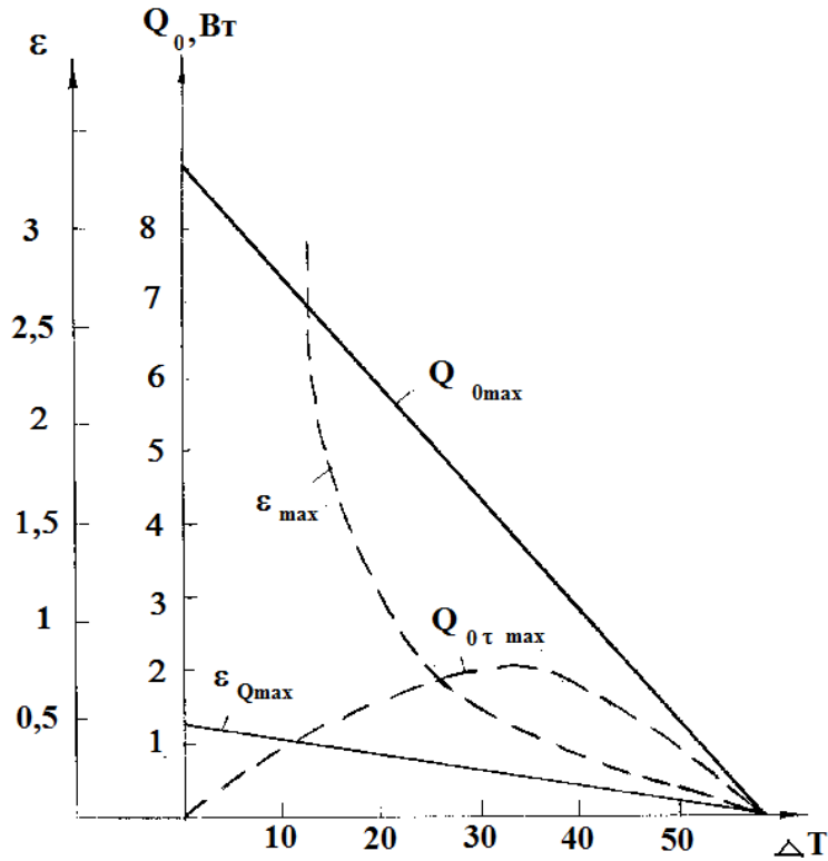
Рис 2.4. Якісний характер залежностей: \varepsilon_{\max} = f(\Delta T) ; Q_{0 \varepsilon_{\max}} = f(\Delta T) \varepsilon_{Q_{\max}} = f(\Delta T) ;
