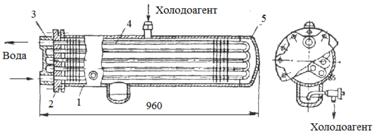
Рис. 5.3. Кожухозмієвидні конденсатори
