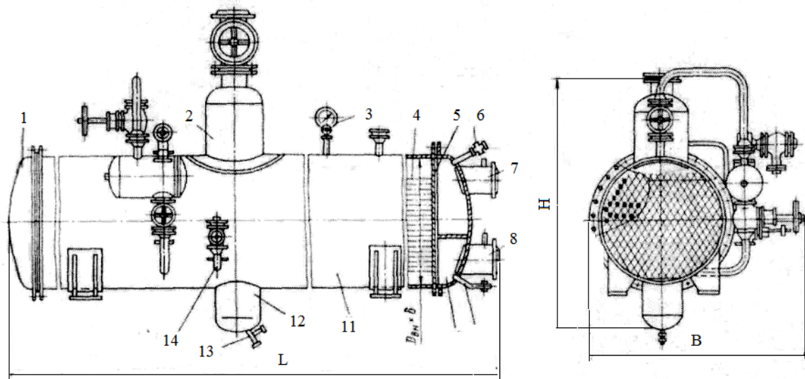
Рис.6.1. Амiачний кожухотрубчастий випаровувач заповненого типу: 1, 10 - кришки; 2 - сухопарник; 3 - манометр; 4 - труби; 5 - трубна решiтка; 6 - вентиль для випуску повітря; 7, 8 - штуцера для введення i вiдведення розсолу; 9 - злив розсолу; 11 - корпус; 12 - масловiдстiйник; 13 - кран для видалення мастила; 14 - патрубок для входу рiдкого амiаку
