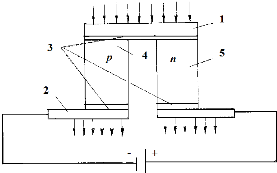
Рис 2.2. Схема напівпровідникового елемента: 1,2 – струмопровідні шини; 3-комутаційні переходи; 4-елемент р-типу; 5-елемент n-типу.
