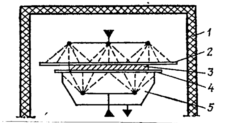
Рис. 15.10. Схема заморожування продукту за умови контакту з двома стальними стрічками: 1 – теплоізоляційна огорожа; 2 – стрічка верхнього конвеєра; 3 – продукт; 4 – стрічка нижнього конвеєра; 5 – ємність з холодоносієм
