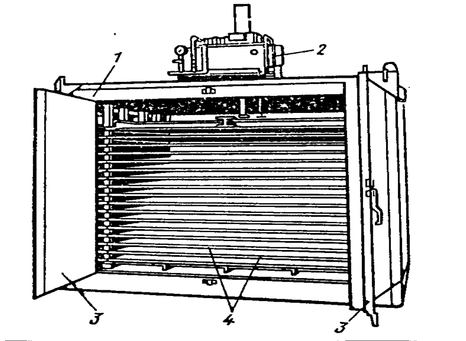
Рис. 15.7. Плитковий апарат: 1 – теплоізоляційна огорожа; 2 – гідравлічний привід; 3 – ствірки; 4 – морозильні плити
