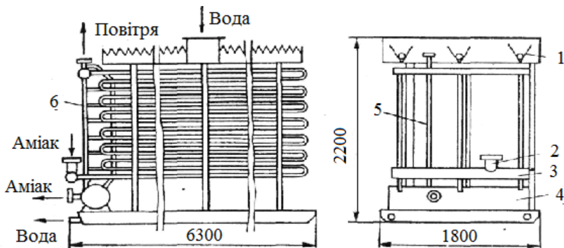
Рис. 5.6. — Зрошувальний конденсатор.
