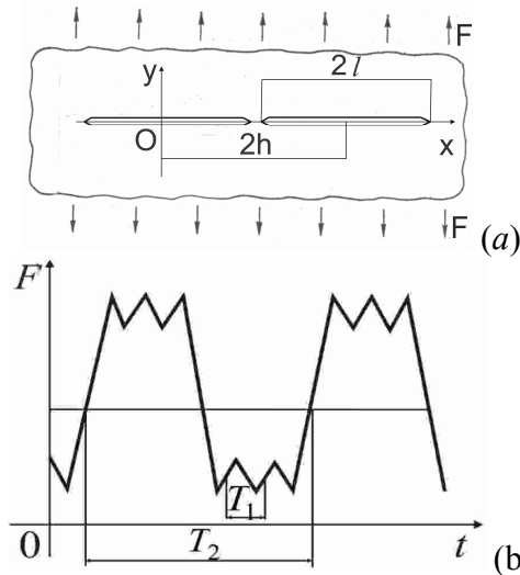
Рисунок 3. Схеми навантаження пластини з періодичною системою тріщин (а) і зміни блочного навантаження (b)
