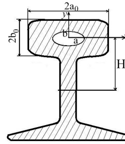
Рисунок 7. Поперечний переріз рейки з тріщиною
