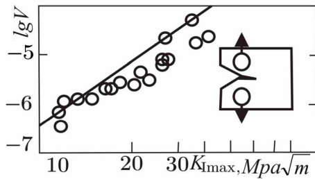
Рисунок 5. Графічне порівняння теоретичних (суцільна лінія) і експериментальних (кружечки) залежностей V \sim K_{Imax} для двочастотного навантаження
