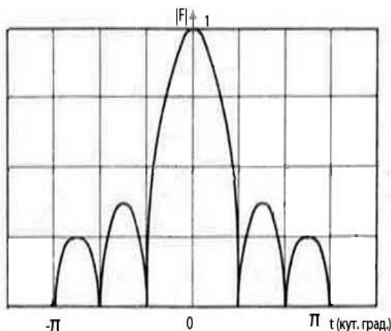
Рис. 1. Класична діаграма випромінювання досліджуваної в декартових координатах.
