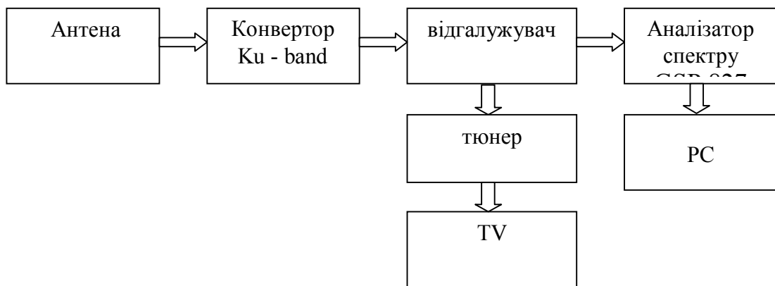
Рис. 4. Структурна схема вимірювання та аналізу ДВ.
