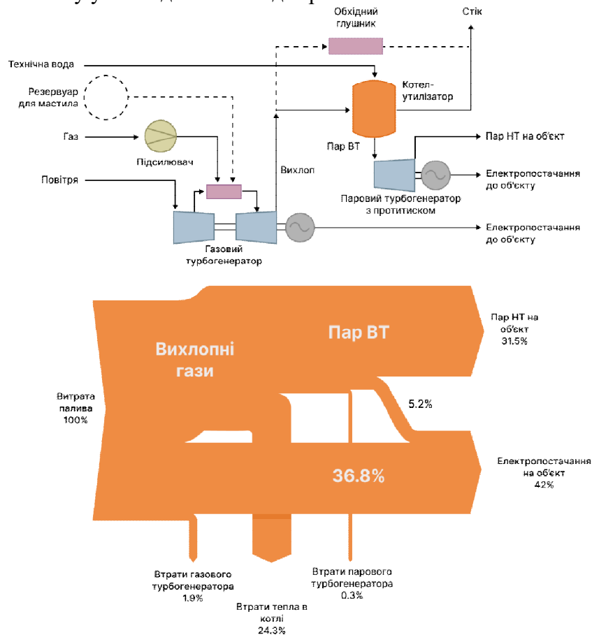
Схема енергетичних потоків для газотурбінної ТЕС з комбінованим циклом
