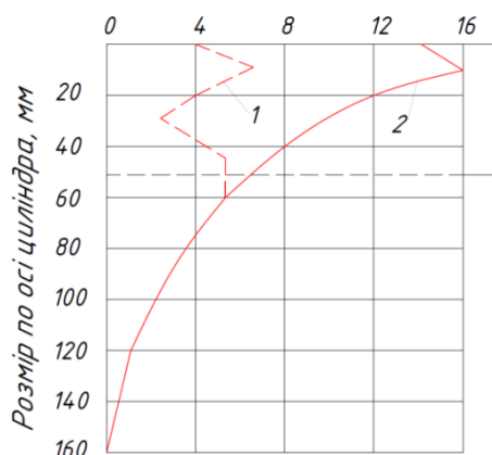
Рисунок 2 – Розподіл величини зносу по поверхні тертя гільзи циліндр автомобіля (величина пробігу 1000 км): 1 – поршень із вставкою, 2 – поршень без вставки
