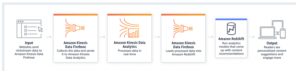
Рисунок 1 - Приклад використання сервісів Kinesis
