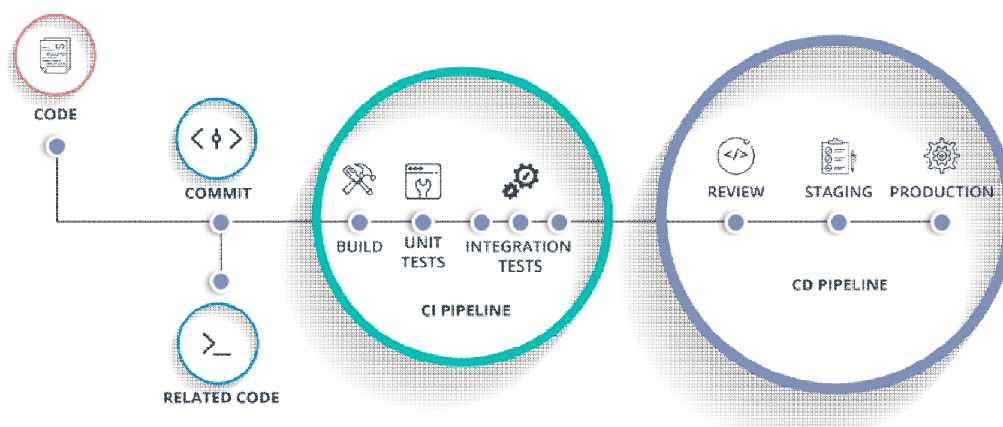
Рисунок 1. Конвеєри CI/CD
