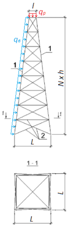
Рисунок 12.1 – Схема вежі
