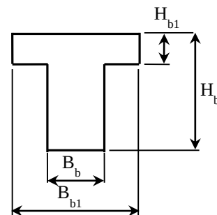
Переріз ригеля
