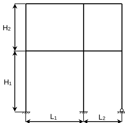
Рисунок 2.1 – Схема рами
