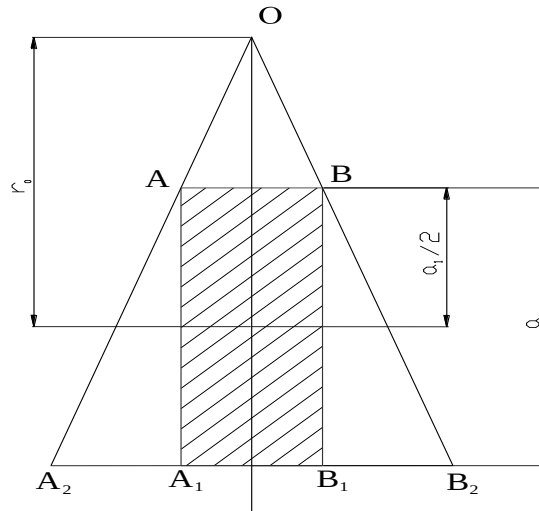
Рис. 1 Схема поперечного січення елемента деформованої стружки а відносна поперечна деформація
