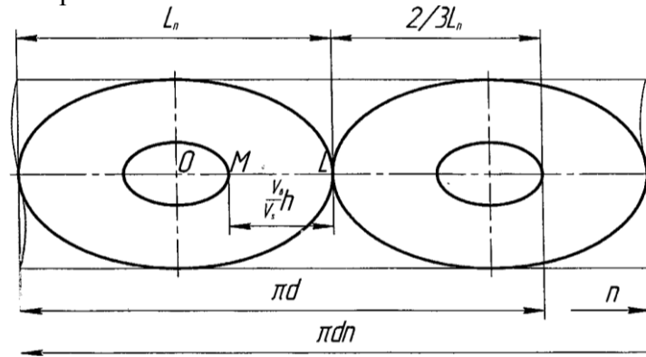
Рисунок 2 – Розташування п'ятен контакту шліфувального круга на шийки валу.
