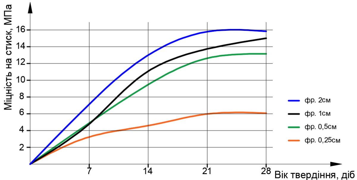
Рис.1 – Міцність бетонів з різними величинами крупного наповнювача у віці 7, 14, 21 і 28 діб
