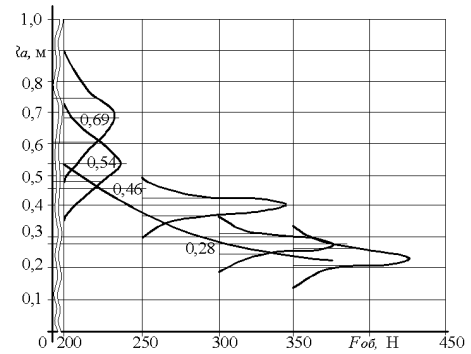
Рис. 2 Теоретичні криві Гауса розподілу параметра шорсткості R_a при різних значеннях зусилля обкочування F_{об}
