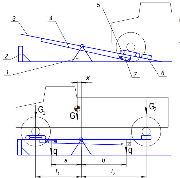
Рисунок 1 – Кінематична схема підіймача
