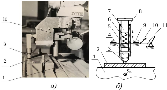
Рис. 1. Загальний вигляд – а) і кінематична схема – б) пристрою для вібраційного обкочування плоских поверхонь змонтованого на пінолі широкоуніверсального верстата мод. 6A75B
