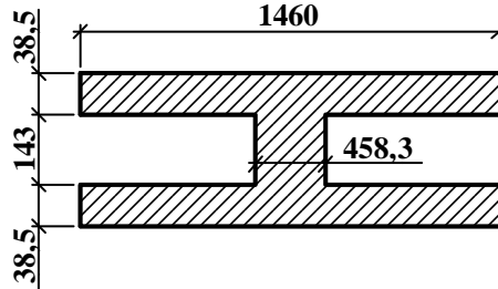
Рис. 2.5. Поперечний переріз багатопустотних плит.
