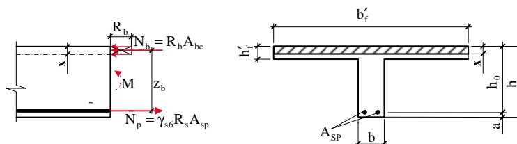
Рис. 2.2. Схема зусиль при розрахунку міцності за нормальним перерізом.
