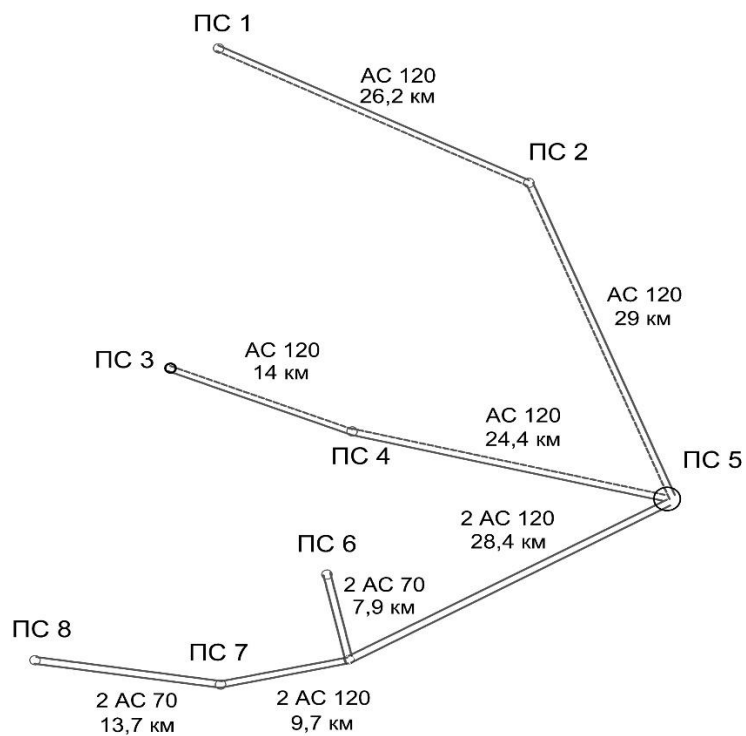
Рисунок 3.2 - Електрична схема з'єднань II-го варіанту
