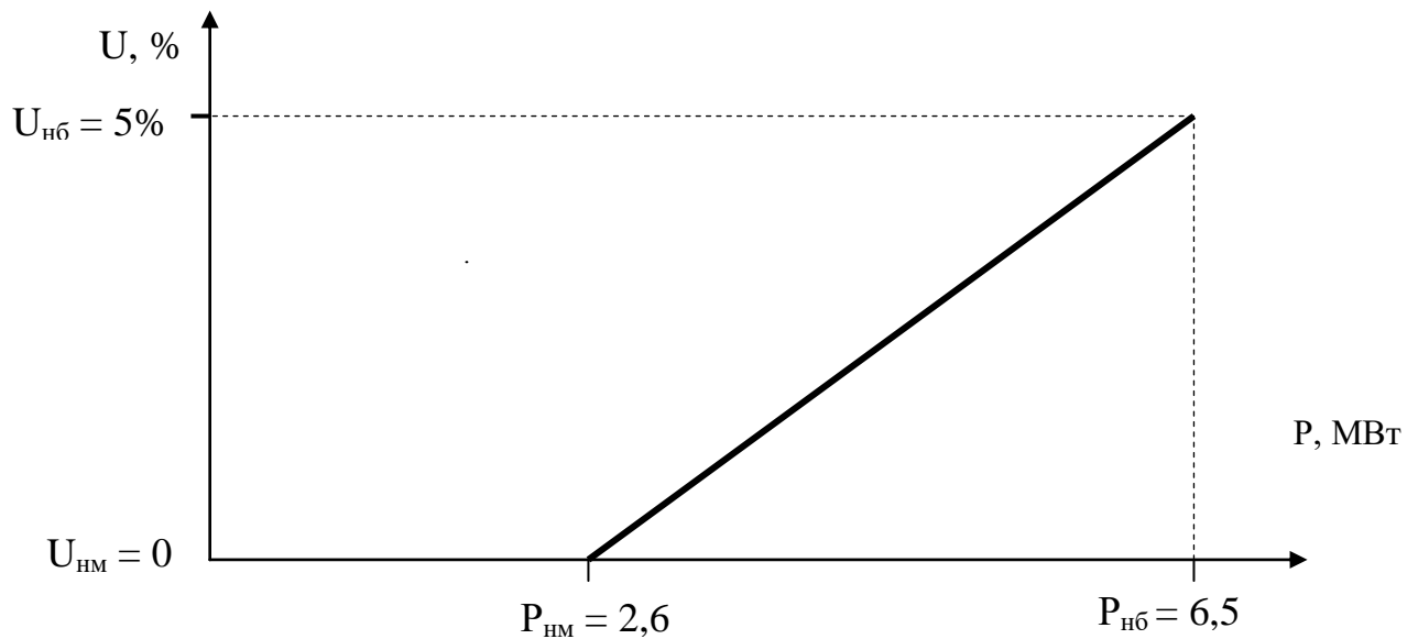
Рис. 5.1 - Закон регулювання напруги
