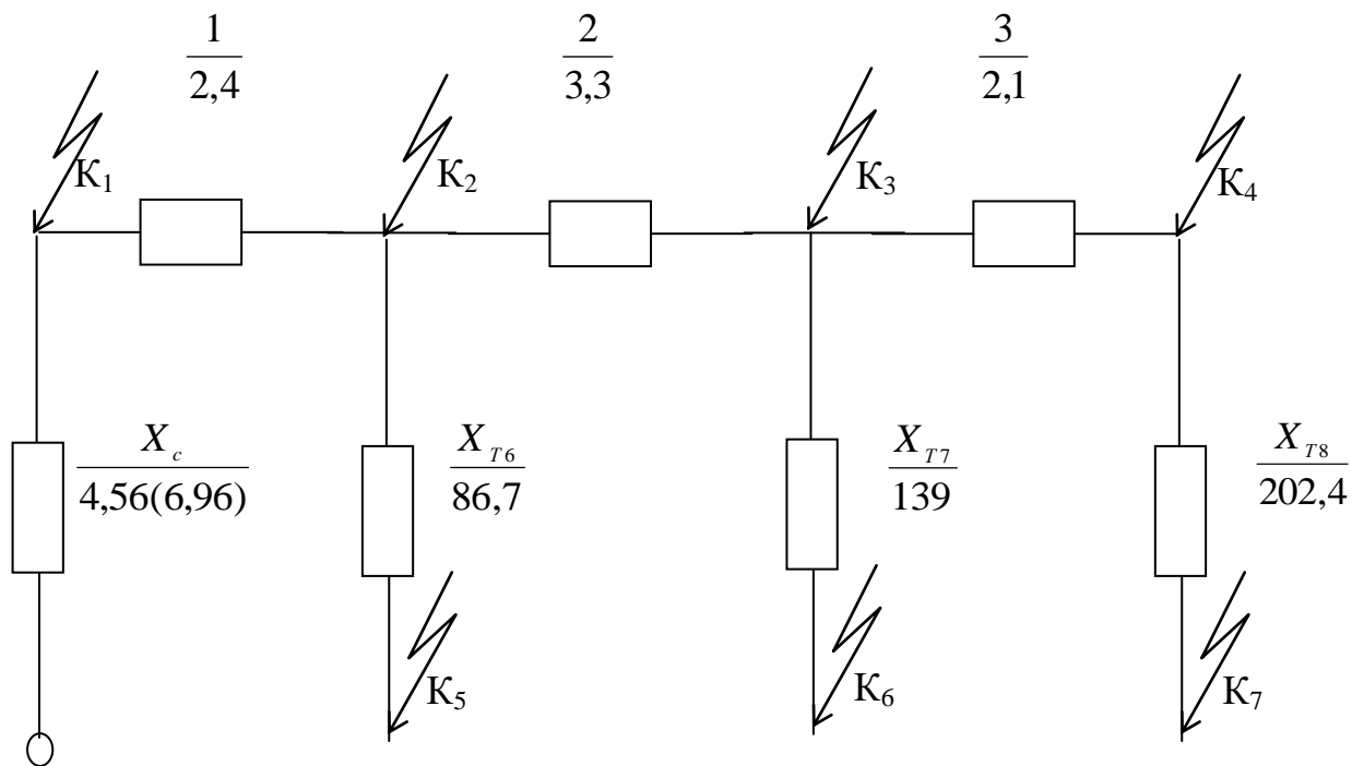
Рисунок 4.3 - Схема для розрахунків струмів КЗ - розрахункова
