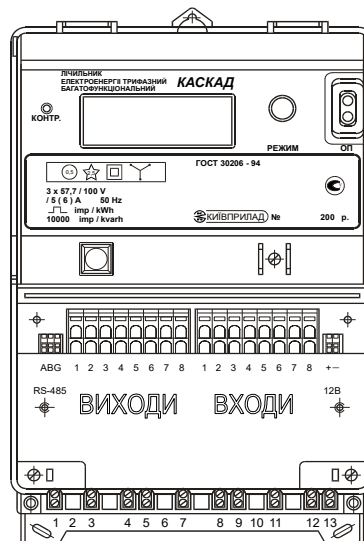
Рисунок 3.5 – Зовнішній вигляд лічильника «Каскад»
