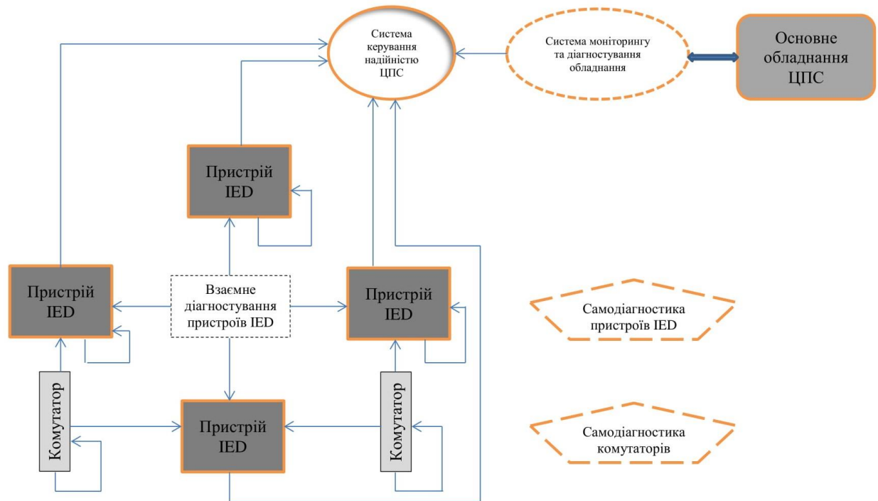
Рис. 2.1 – Схема інформаційних потоків на трансформаторній підстанції з цифровим електроустаткуванням
