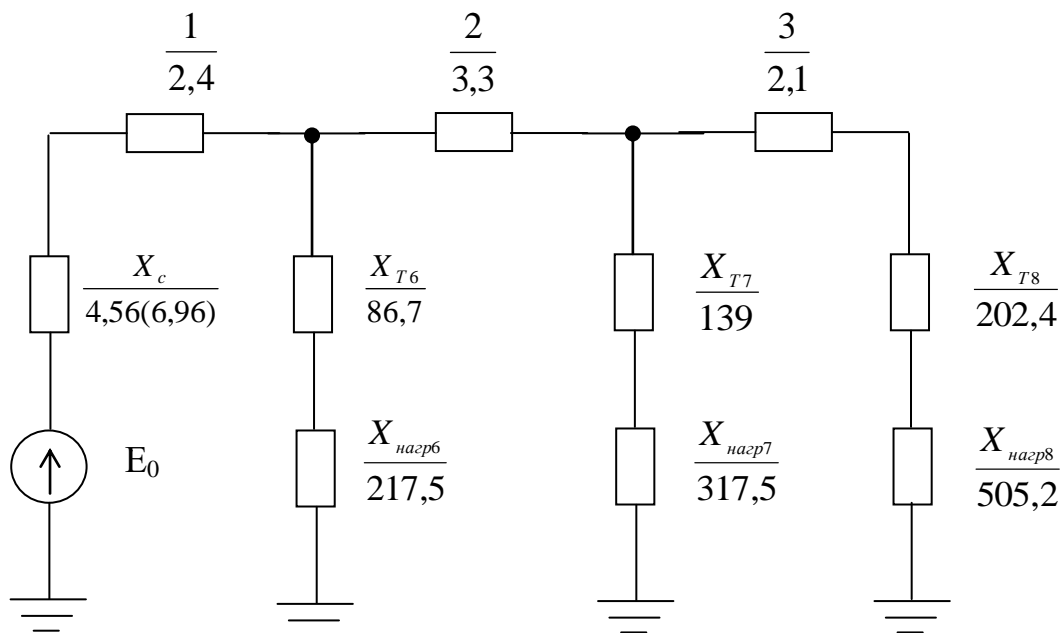
Рисунок 4.5 - Схема заміщення для визначення I_{сзн}
