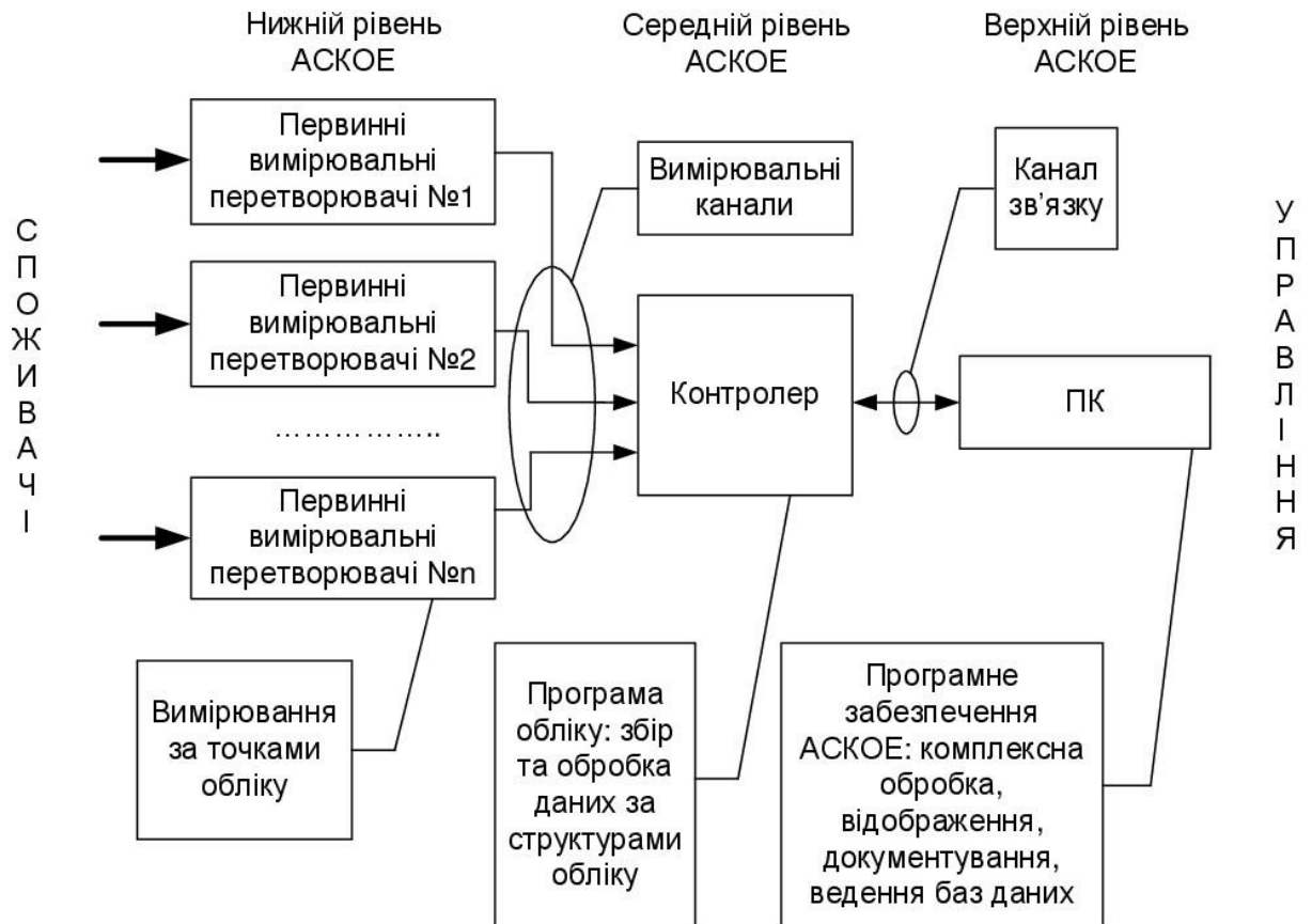
Рисунок 1.4 - Узагальнена схема трирівневої АСКОЕ
