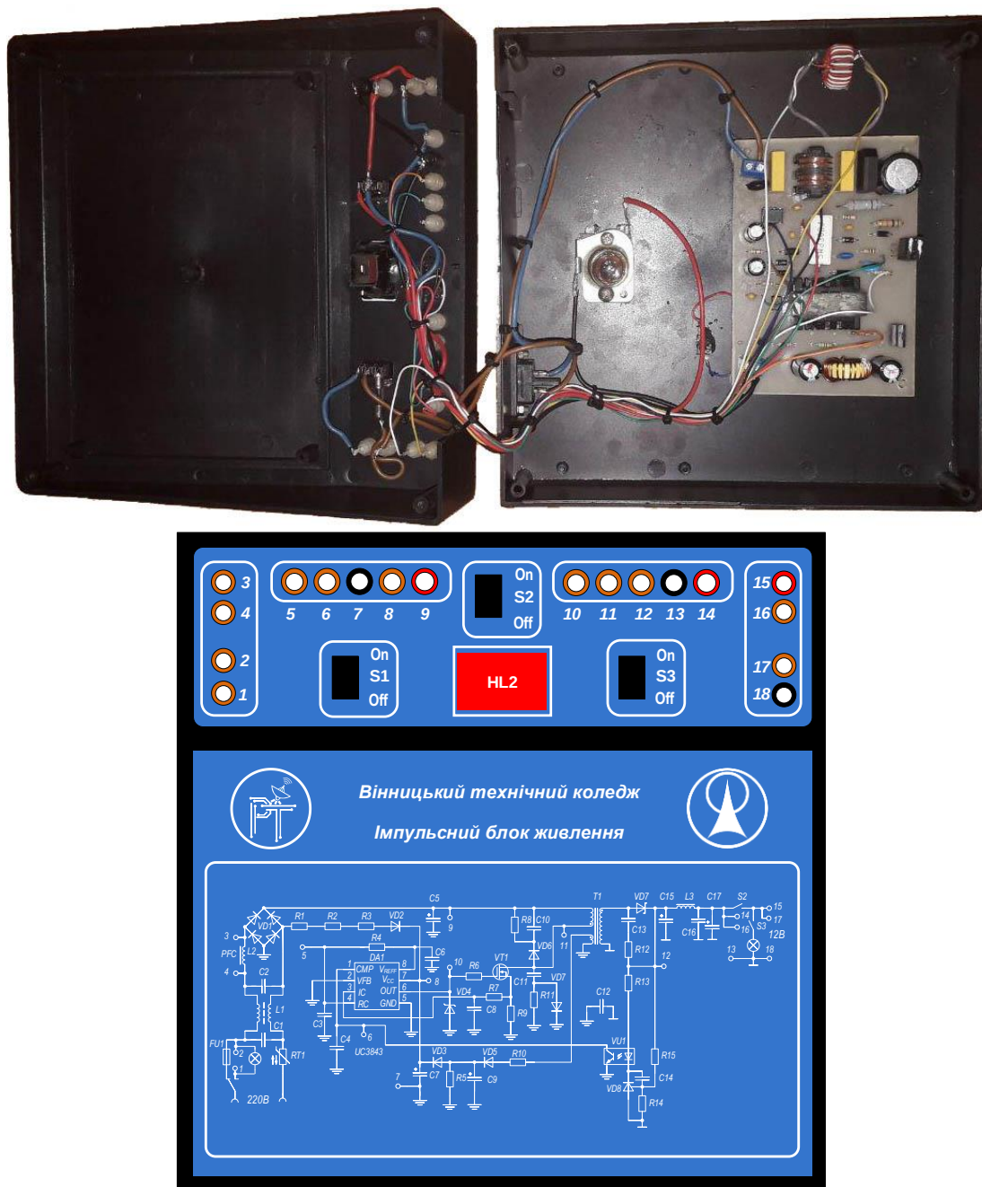
Рис. 2. Конструкція лабораторного блоку живлення
