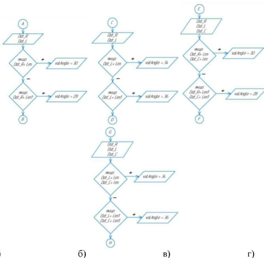
Рис. 2. Блок-схеми алгоритмів опрацювання показів датчиків і встановлення позиції кута повороту коліс: а) орієнтація по правому датчю відстані; б) орієнтація по лівому датчю відстані; в) орієнтація по правому та центральному датчю відстані; г) орієнтація по лівому та центральному датчю відстані.
