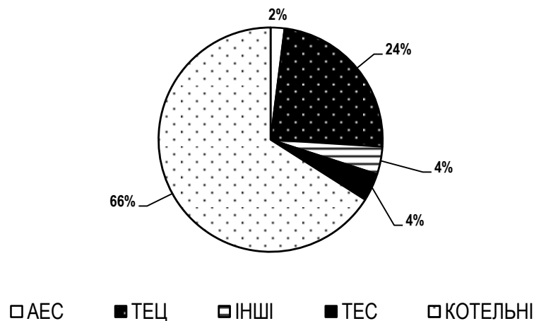
Рис.1. Установлена теплова потужність в Україні у 2017 р., % [2]
