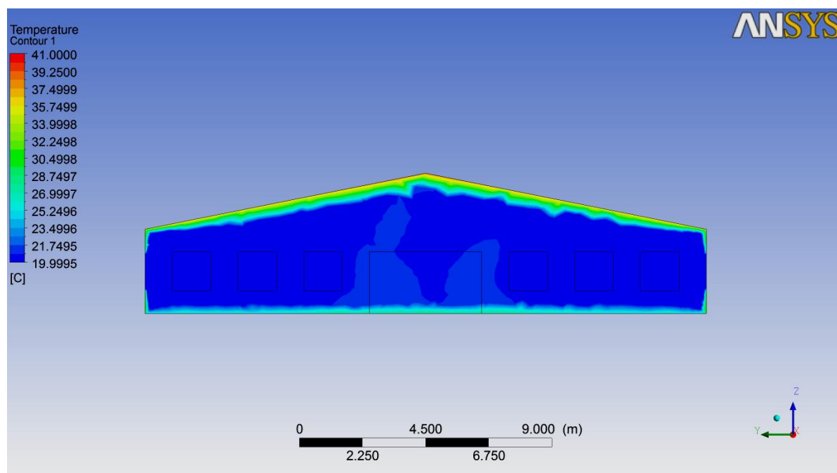
Рис. Г.8. Температурне поле в приміщенні пташника в поперечному перерізі будівлі по осі Oy на відстані 2 м від входу, ^{\circ}\text{C}
