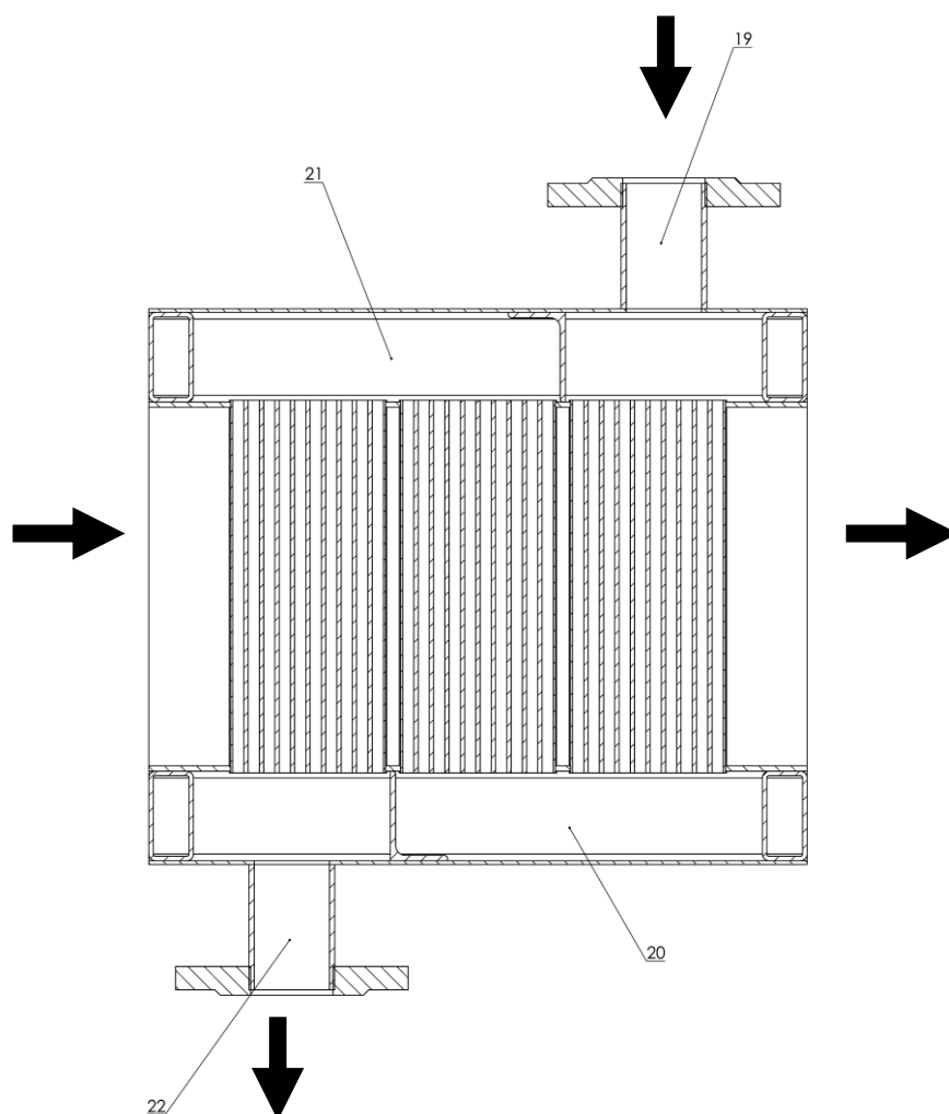
Рис. 4.4. Схематичне розташування датчиків температури в поперечному розрізі теплообмінного апарату
