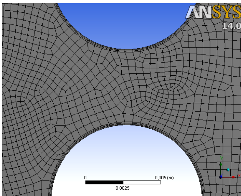
Рис. В.3. Чотирикутна сітка з методом межового шару ЗТ в кількості 3 шари з початковою товщиною 3 \cdot 10^{-5} м
