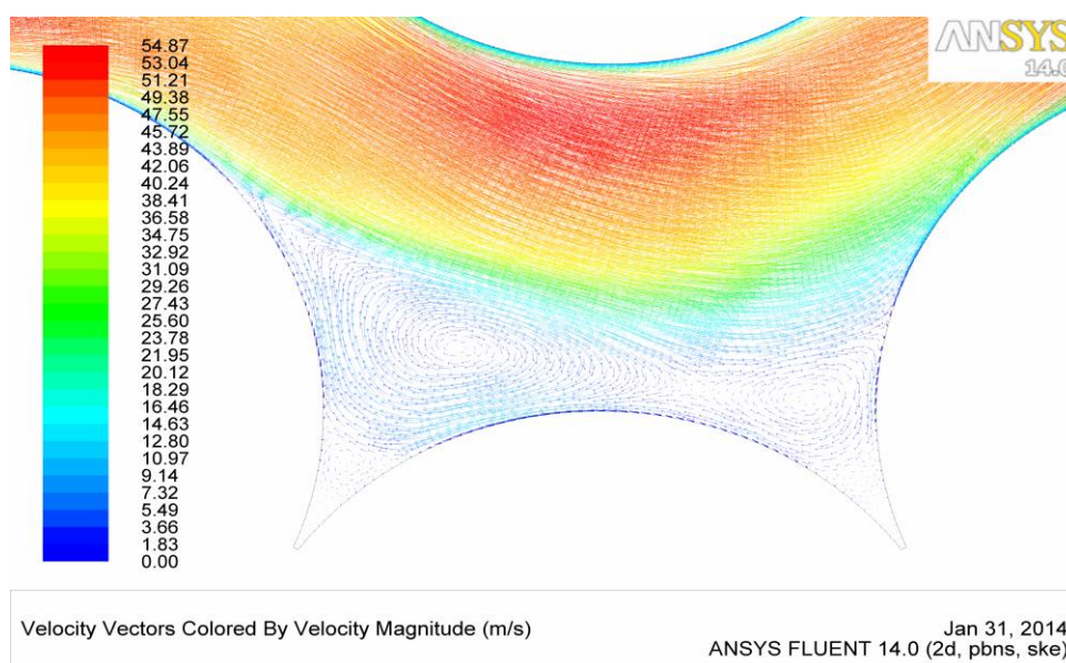
Рис. 3.12. Вектор швидкості в каналі, м/с
