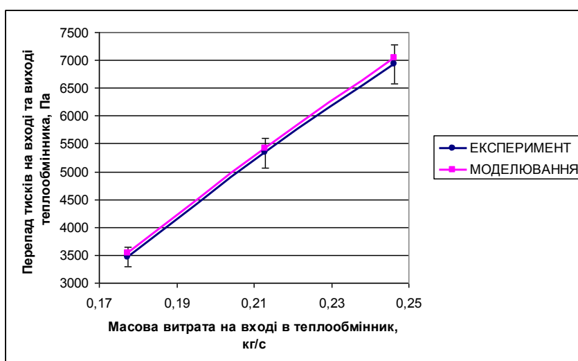
Рис. 4.11. Залежність падіння тиску від масової витрати на вході в теплообмінник
