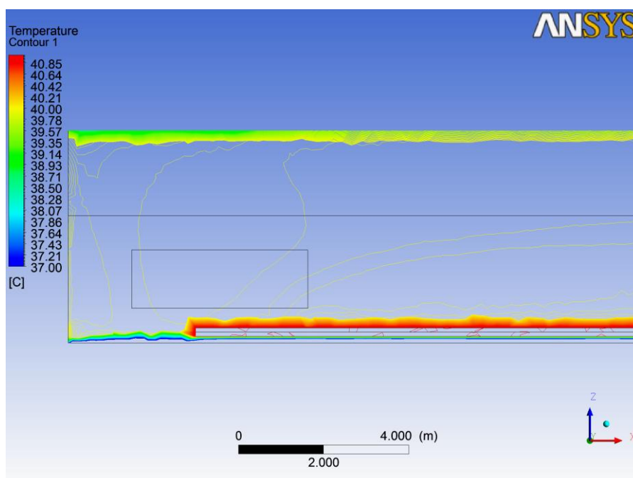
Рис. Г.2. Контурне поле температур в поздовжньому перерізі будівлі на відстані 6 м від стінки біля входу в інтервалі від 37 до 41, °C
