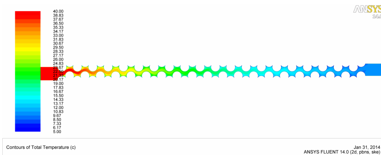
Рис. 3.13. Зміна температури в каналі, °C
