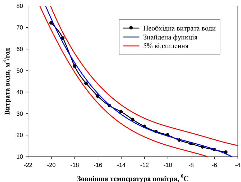
Рис. 2.28. Витрата води, яка необхідна для нагрівання припливного повітря в пташнику у зимовий період року в залежності від зовнішньої температури повітря
