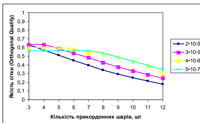
Рис. В.6. Графік залежності якості гібридної сітки від кількості межових шарів в межах товщини першого шару від 2 \cdot 10^{-5} м до 5 \cdot 10^{-5} м
