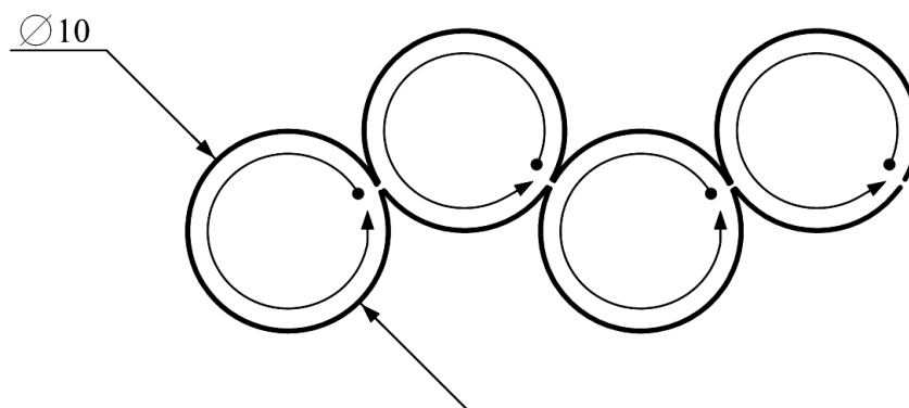
Рис. 3.25. Початкова і кінцева розрахункова точка по периметру труби пучка
