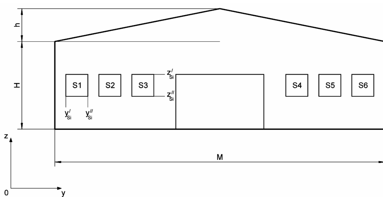
Рис. 2.8. Передня торцева стінка пташника
