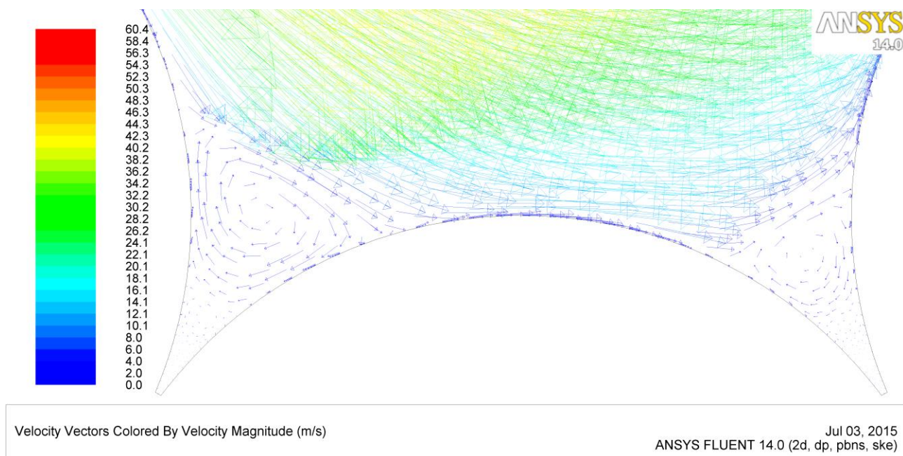
Рис. 3.22. Вектор швидкості в каналі, м/с
