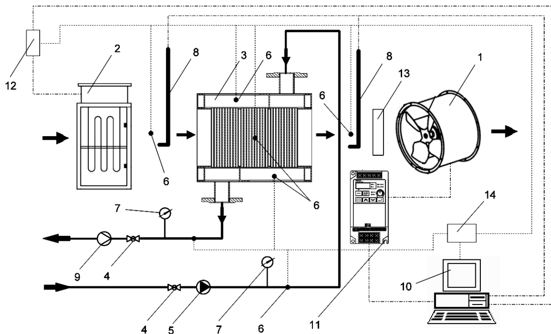
Рис. 4.2. Тепло-гідравлічна схема експериментальної установки модернізованого електротехнічного комплексу: 1 – вентилятор, 2 – ТЕНи, 3 – теплообмінник-рекуператор, 4 – вентиль, 5 – циркуляційний насос, 6 – накладні датчики температури, 7 – манометр, 8 – трубка Піто-Прандтля, 9 – витратомір, 10
