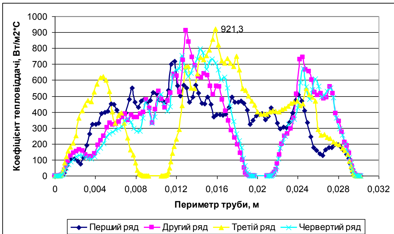
Рис. 3.26. Розподіл місцевої тепловіддачі по периметру труби запропонованого пучка при Re=18150
