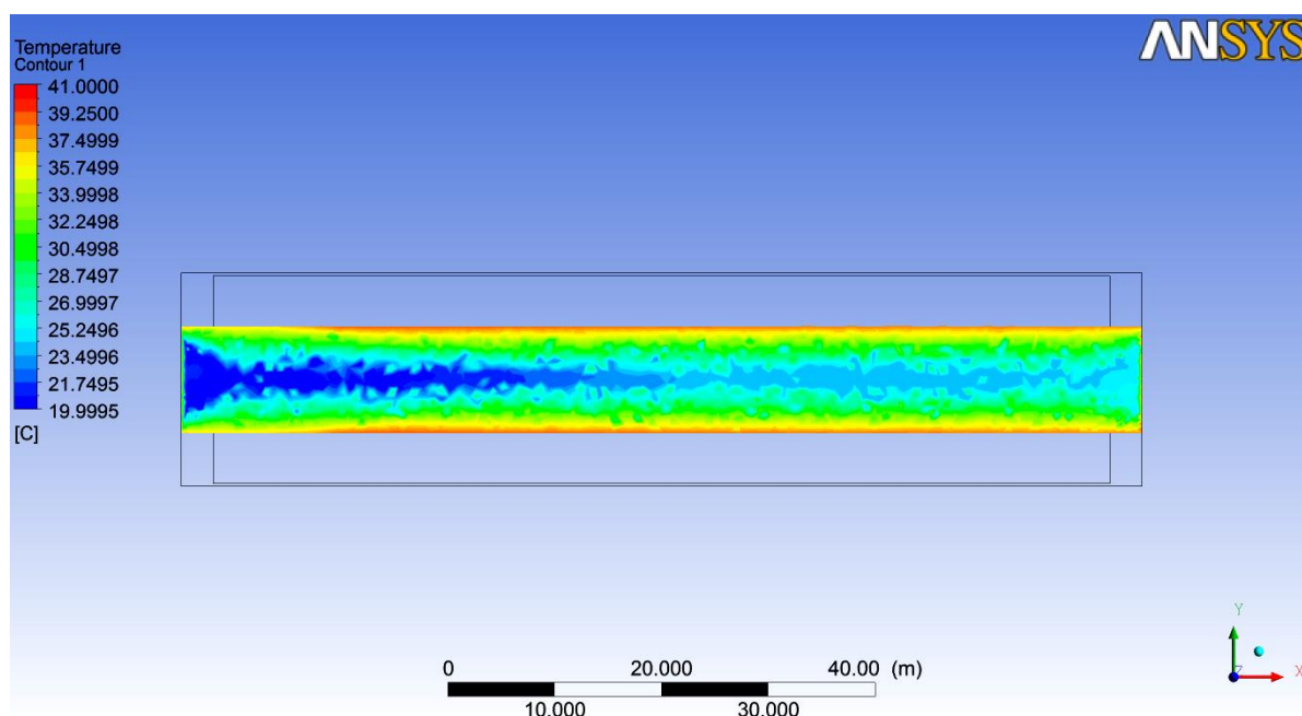
Рис. Г.11. Температурне поле в приміщенні пташника в поперечному перерізі будівлі по осі Oz на висоті 2,5 м від підлоги, ^{\circ}\text{C}
