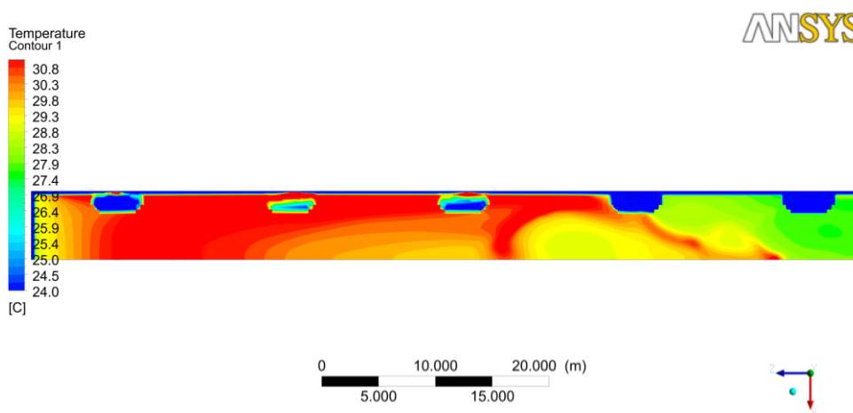
Рис. 2.25. Температурне поле в приміщення пташника в межах від 24 до 31 °С
