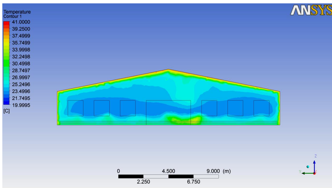
Рис. Г.10. Температурне поле в приміщенні пташника в поперечному перерізі будівлі по осі Oy на відстані 88 м від входу, ^{\circ}\text{C}
