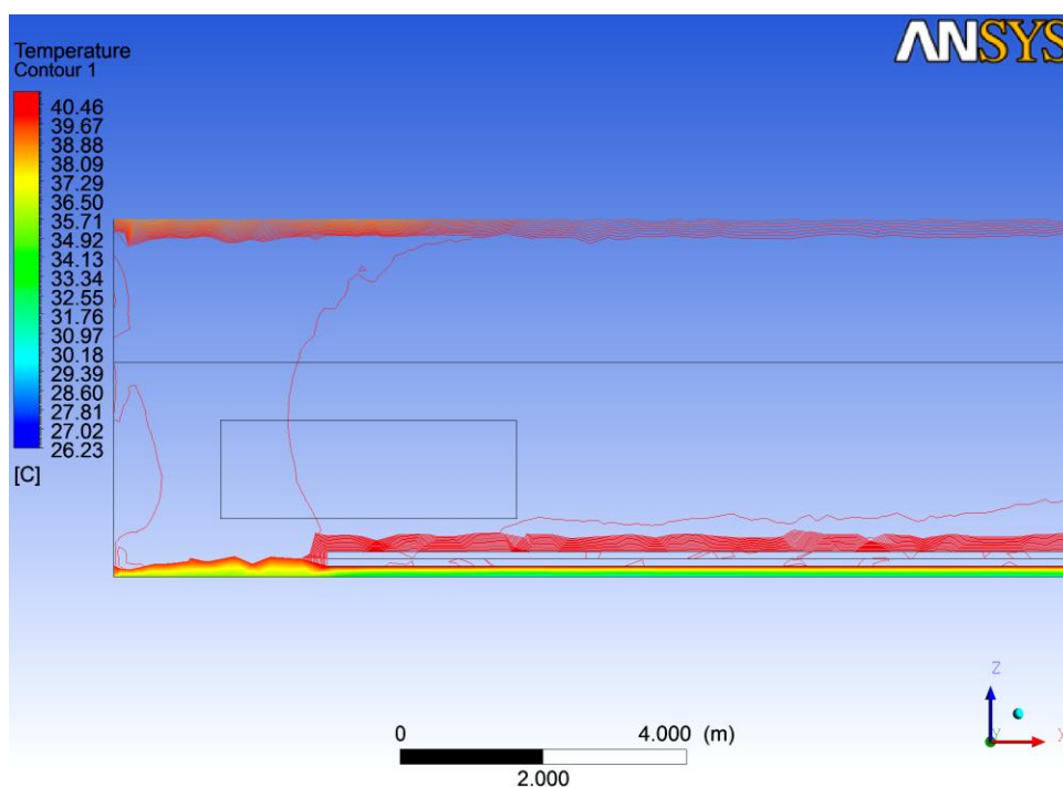
Рис. Г.1. Контурне поле температур в поздовжньому перерізі будівлі на відстані 6 м від стінки біля входу в інтервалі від 26 до 41, °C
