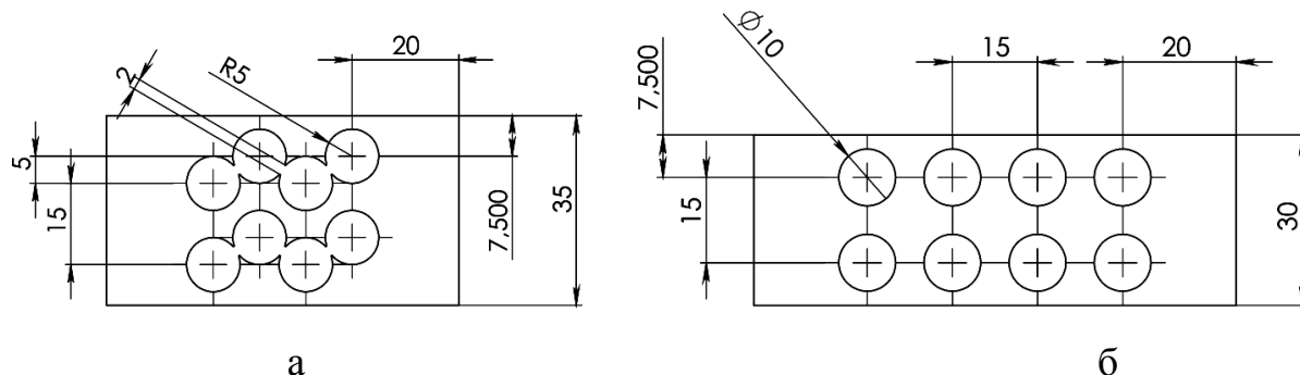
Рис. В.1. – Розташування труб в пучку (вигляд зверху): а – із зміщенням труб на 5 мм; б – традиційне коридорне розташування.
