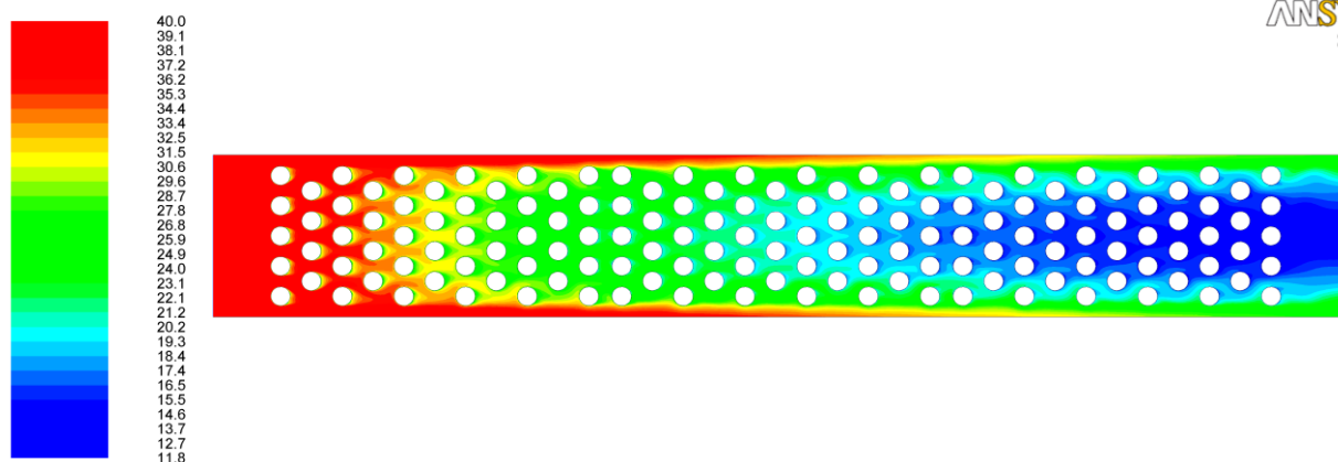
Рис. 3.6. Зміна температури в каналі шахового пучка, °C
