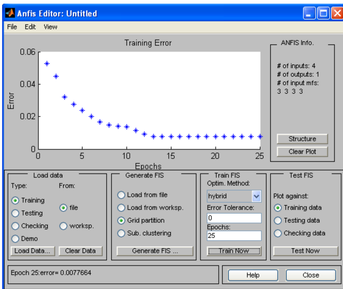
Рис. 4.18. Результати навчання мережі
