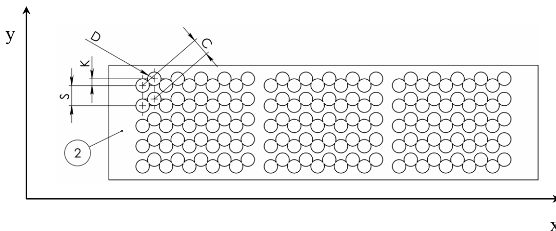
Рис. 3.2. Трубна дошка з компактним розташуванням трубок (вигляд зверху)
