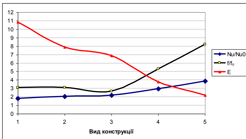
Рис. 3.17. Теплогідравлічна ефективність, відносні величини чисел Нуссельта та коефіцієнтів тертя для різних типів конструкцій пучка труб
