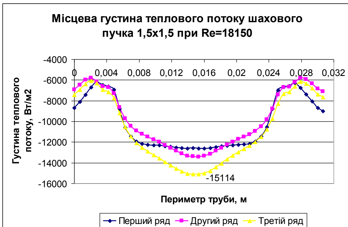
Рис. 3.9. Місцева густина теплового потоку шахового пучка 1,5x1,5 при Re=18150
