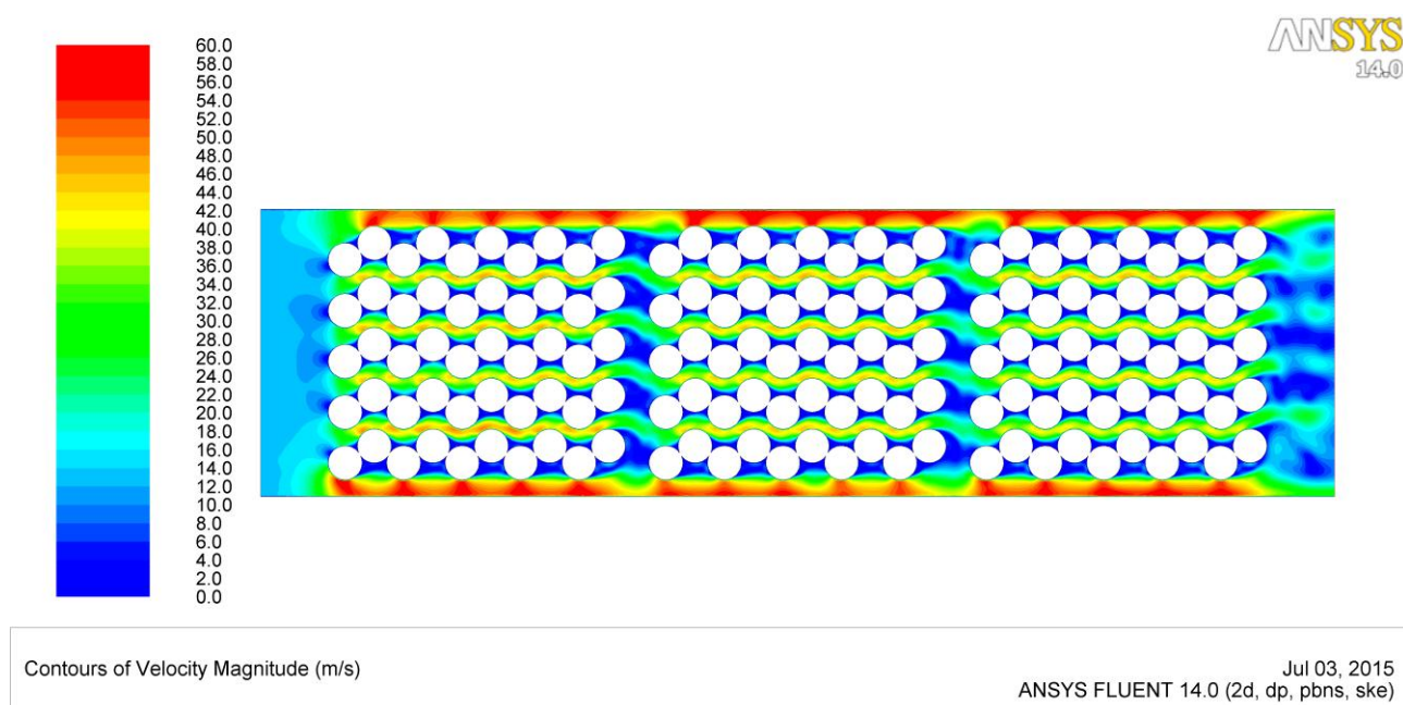
Рис. 3.20. Швидкість повітря в каналі, м/с
