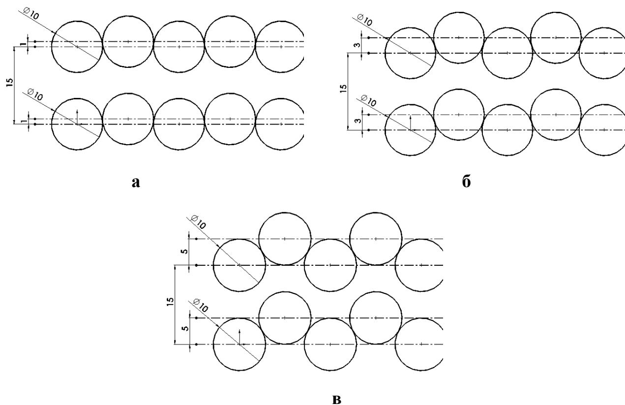
Рис. 3.10. Розташування компактного пучка труб (вигляд зверху): а – зміщення труб на 1 мм, б – зміщення на 3 мм, в – зміщення на 5 мм.
