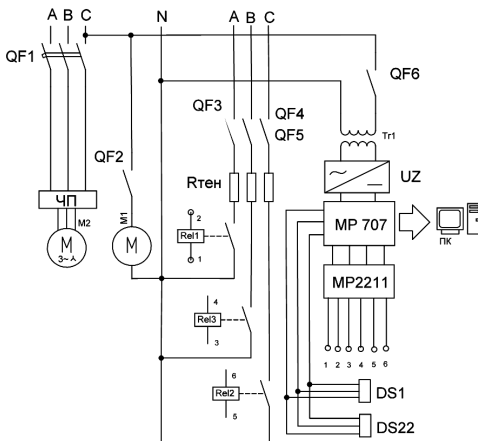
Рис 4.5. Принципова електрична схема експериментальної установки
