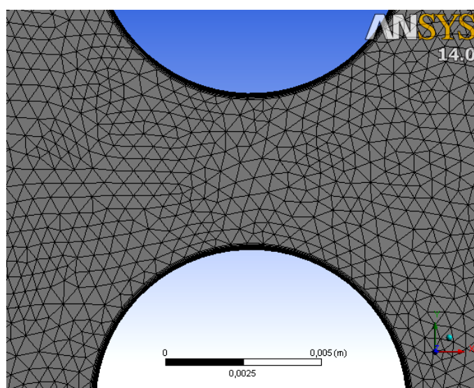
Рис. В.2. Гібридна сітка з методом межового шару 3Т в кількості 12 шарів з початковою товщиною 2 \cdot 10^{-4} м
