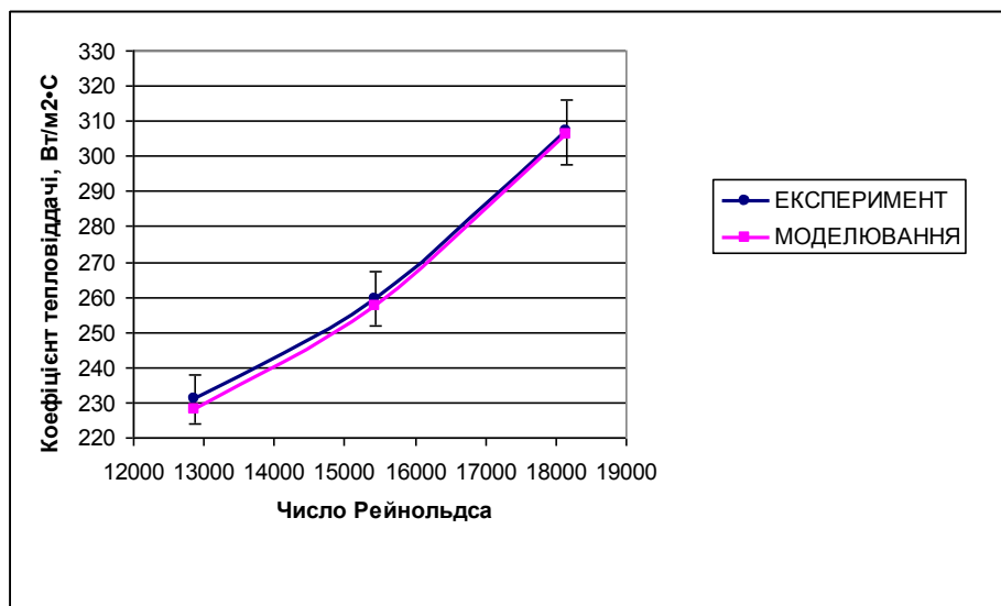
Рис. 4.9. Залежність коефіцієнта тепловіддачі на поверхні трубного пучка від числа Рейнольдса
