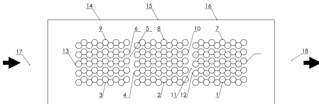
Рис. 4.3. Схематичне розташування датчиків температури в трубному пучку та на зовнішній стінці теплообмінного апарата
