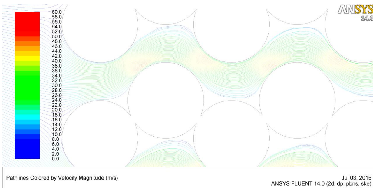
Рис. 3.21. Лінії току в каналі, м/с
