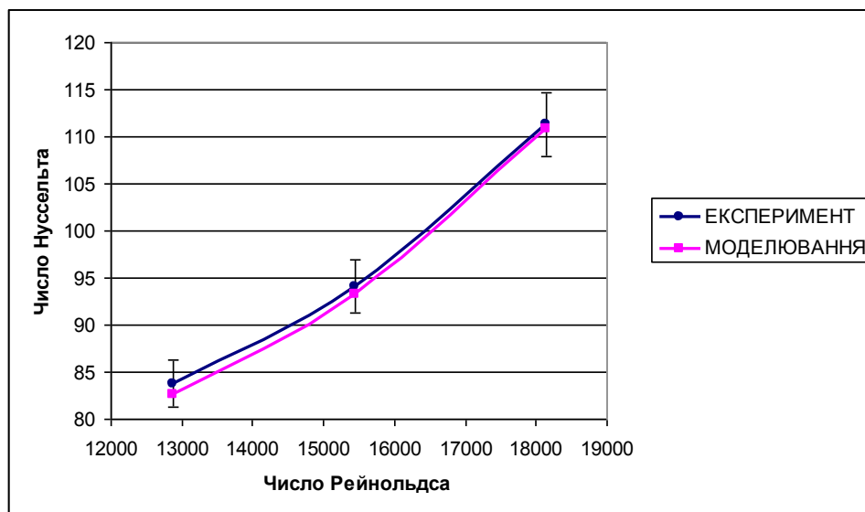
Рис. 4.8. Залежність числа Нуссельта на поверхні трубного пучка від числа Рейнольдса
