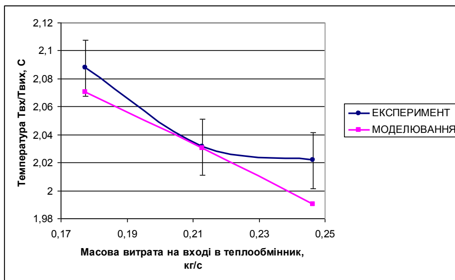
Рис.4.12. Залежність безрозмірної температури повітря на виході від масової витрати на вході в теплообмінник
