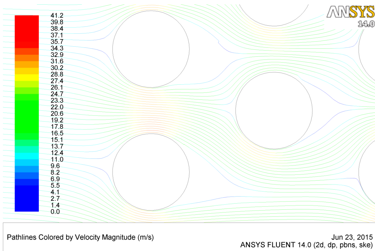
Рис. 3.4. Лінії току на вході в теплообмінник, м/с
