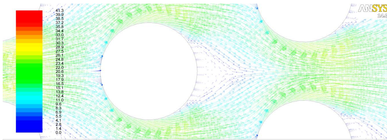
Рис. 3.5. Вектор швидкості в каналі шахового пучка, м/с
