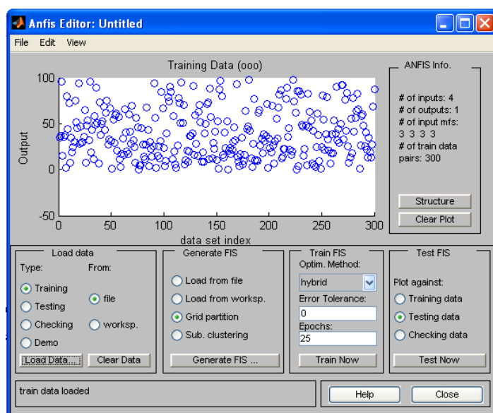
Рис. 4.15. Налаштування ANFIS редактора на навчальну вибірку експериментальних даних
