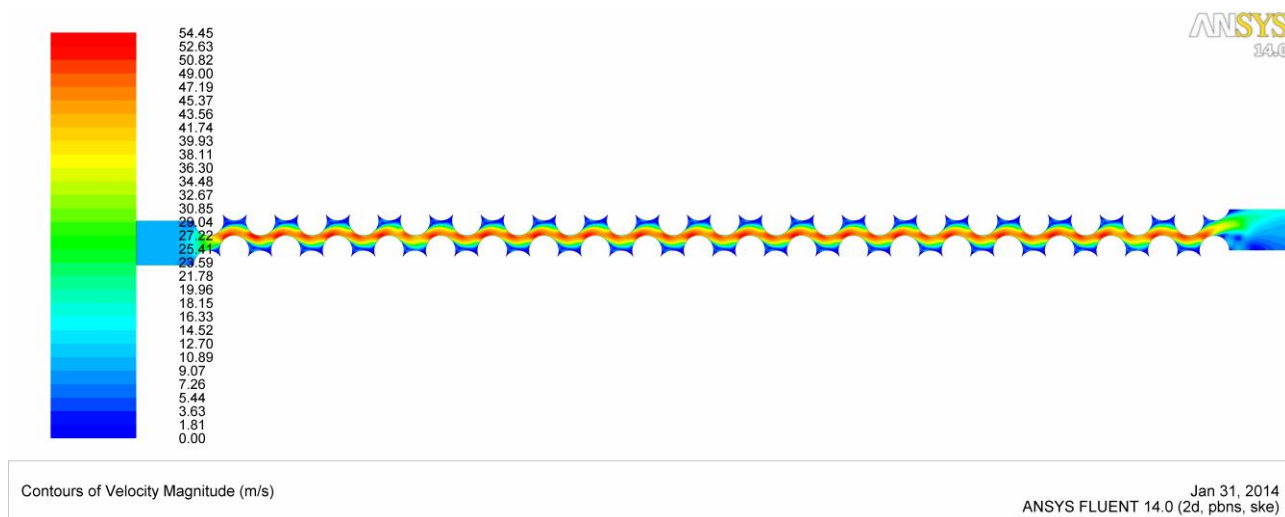
Рис. 3.11. Швидкість повітря в каналі, м/с
