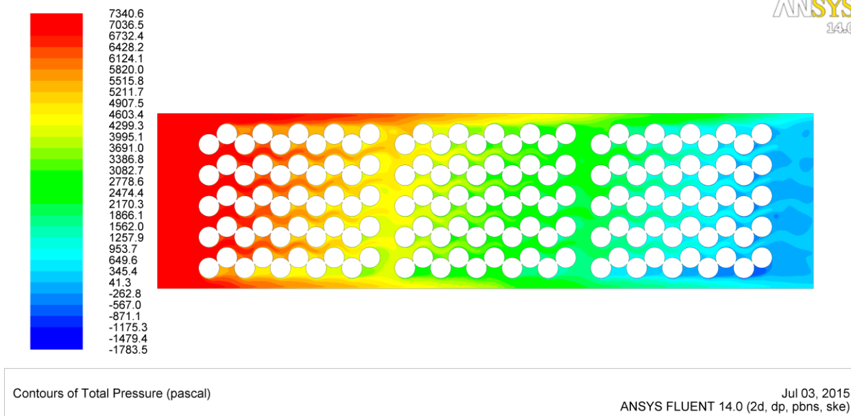
Рис. 3.24. Перепад тиску в каналі, Па
