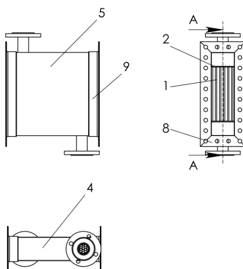
Рис. 4.6. Загальний вигляд кожухотрубного теплообмінника
