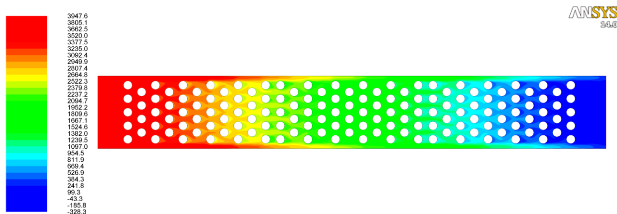
Рис. 3.7. Перепад тиску в каналі шахового пучка, Па
