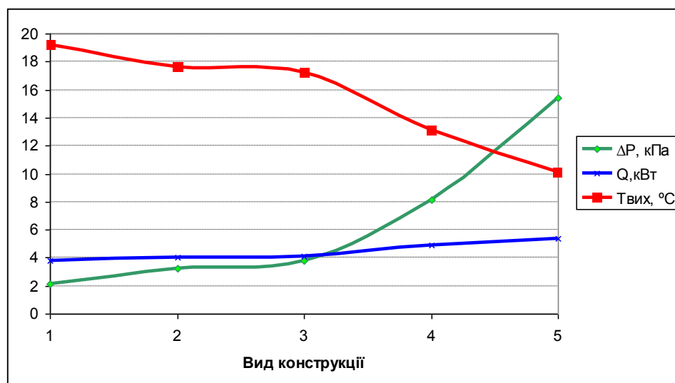
Рис. 3.18. Залежність падіння тиску \Delta P , загальної кількості відведеної теплоти Q та температури теплоносія на виході з теплообмінника t_{вих} від зміни геометрії пучка труб
