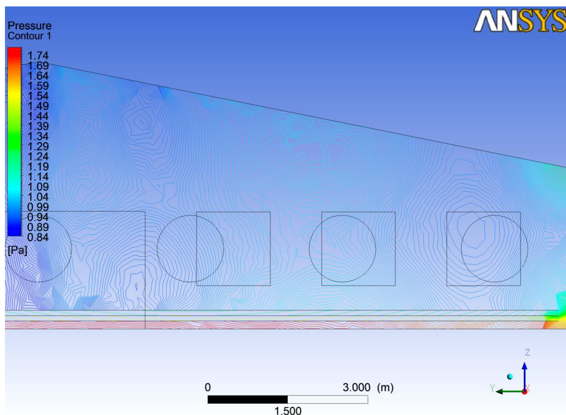
Рис. Г.7. Контурне поле тисків в поперечному перерізі будівлі по осі Oy на відстані 30 м від входу в інтервалі від 0 до 200,0 Па
