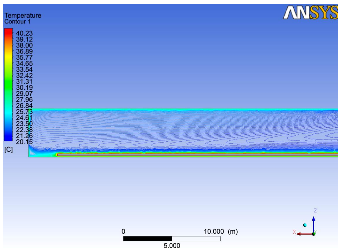
Рис. Г.12. Контурне поле температур в поздовжньому перерізі будівлі по середній лінії на відстані 6 м від стінки біля виходу в інтервалі від 20 до 41, ^{\circ}\text{C}
