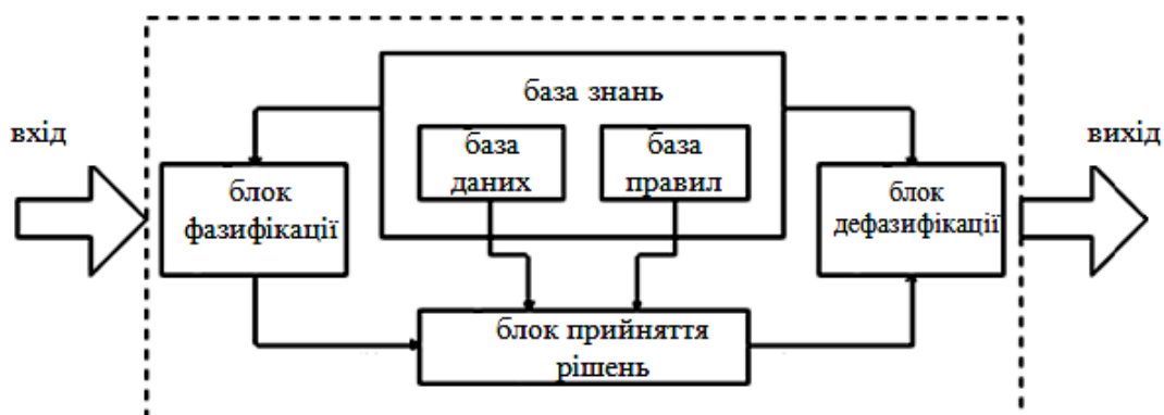
Рис. 4.13. Нейроінфонмаційна система
