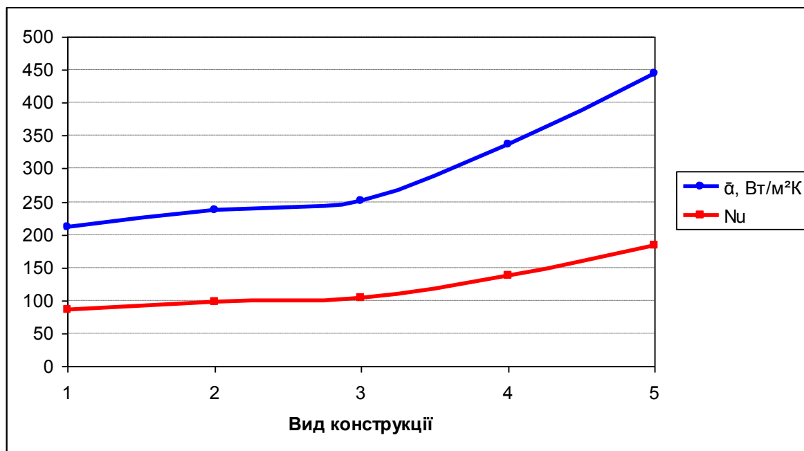
Рис. 3.16. Залежність числа Нуссельта та коефіцієнта тепловіддачі залежно від зміни конструкції пучка труб
