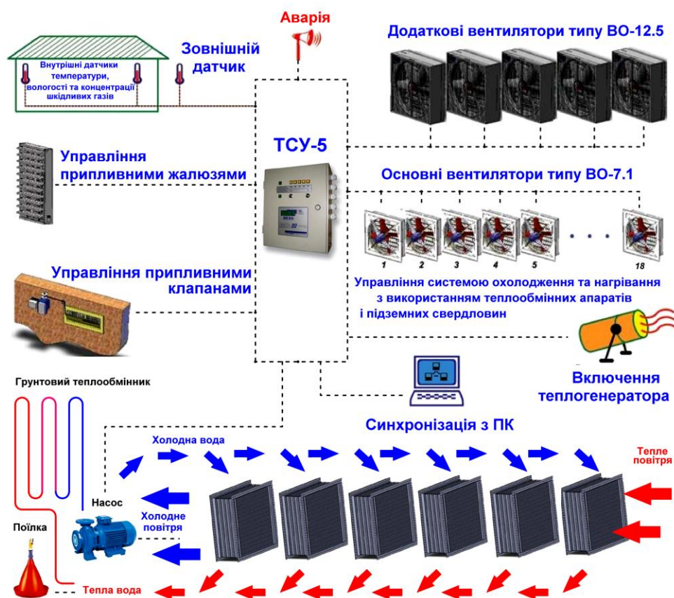
Рис. 2.3 Загальна схема нової системи підтримання оптимального мікроклімату в птахівничих приміщеннях з використанням води підземних свердловин та теплообмінників-рекуператорів
