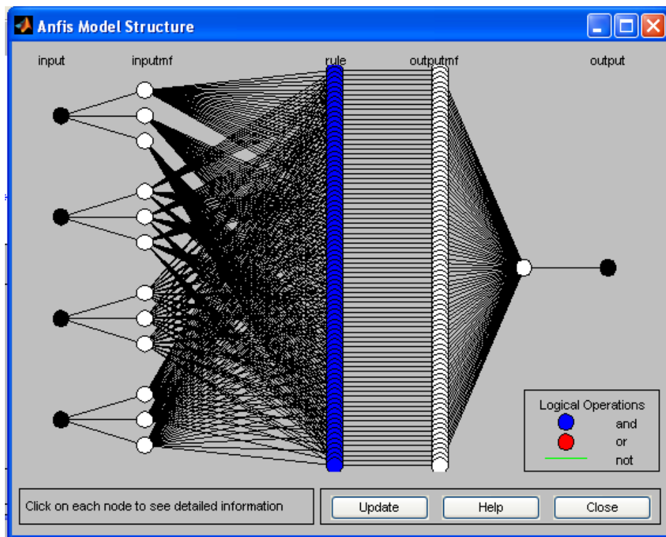
Рис. 4.17. Структура розробленої гібридної мережі
