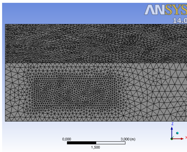
Рис. Б.2. Сітка пташника з бічної сторони
