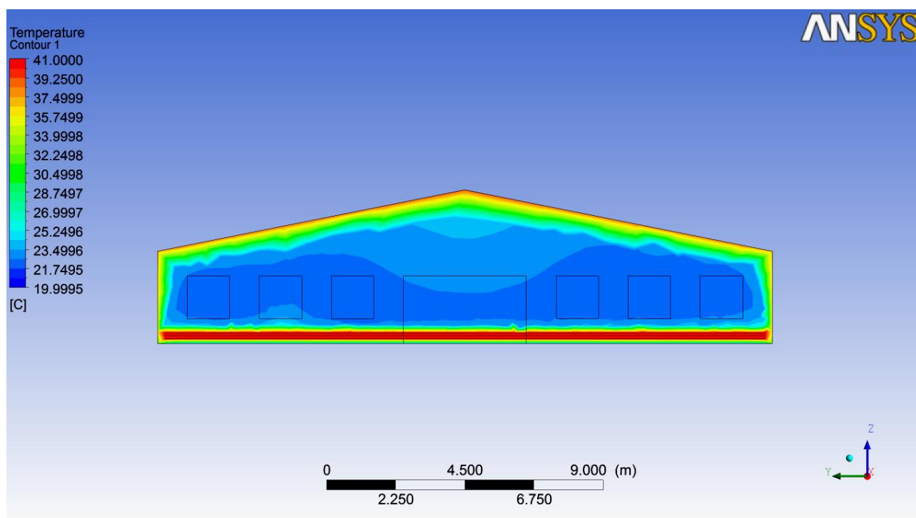
Рис. Г.9. Температурне поле в приміщенні пташника в поперечному перерізі будівлі по осі Oy на відстані 60 м від входу, ^{\circ}\text{C}
