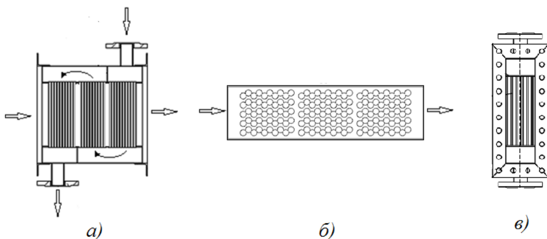
Рис. 3.1 Загальна схема кожухотрубного теплообмінника з компактним розміщенням трубного пучка: а – вигляд збоку; б – вигляд зверху; в – вигляд з торця.
