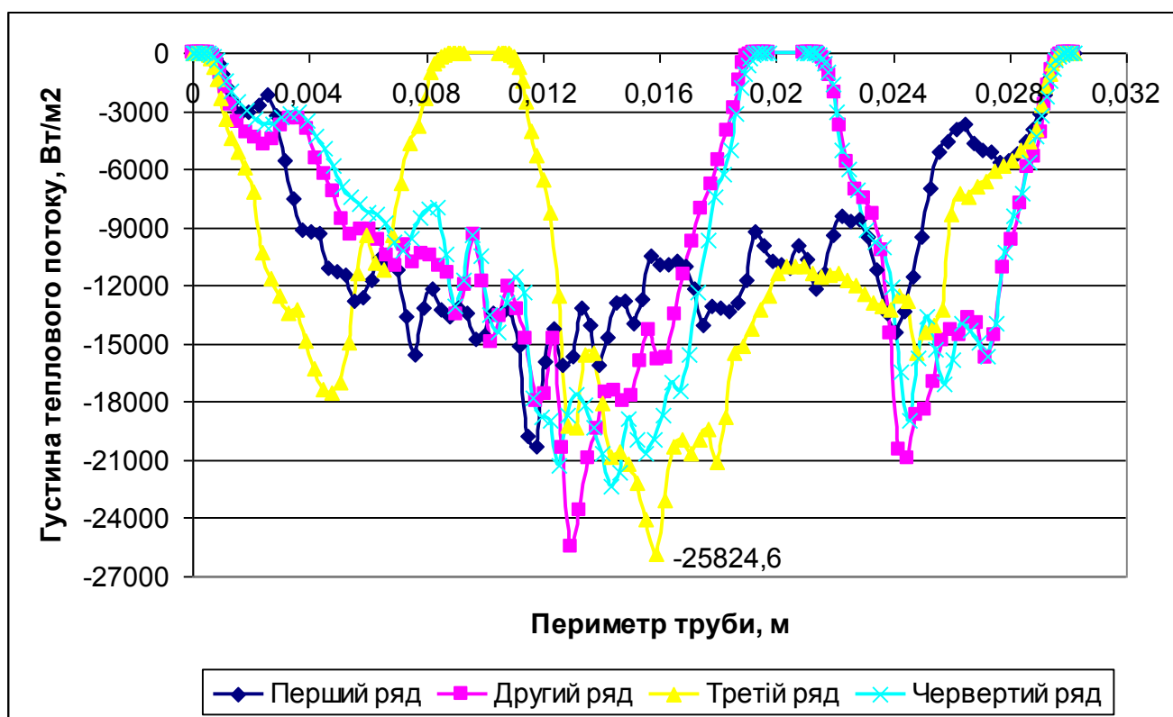
Рис. 3.27. Місцева густина теплового потоку запропонованого пучка при Re=18150
