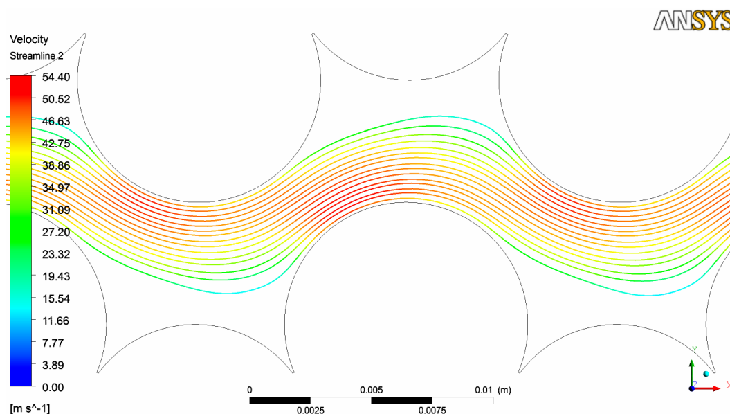
Рис. 3.15. Лінії току швидкості повітря, м/с
