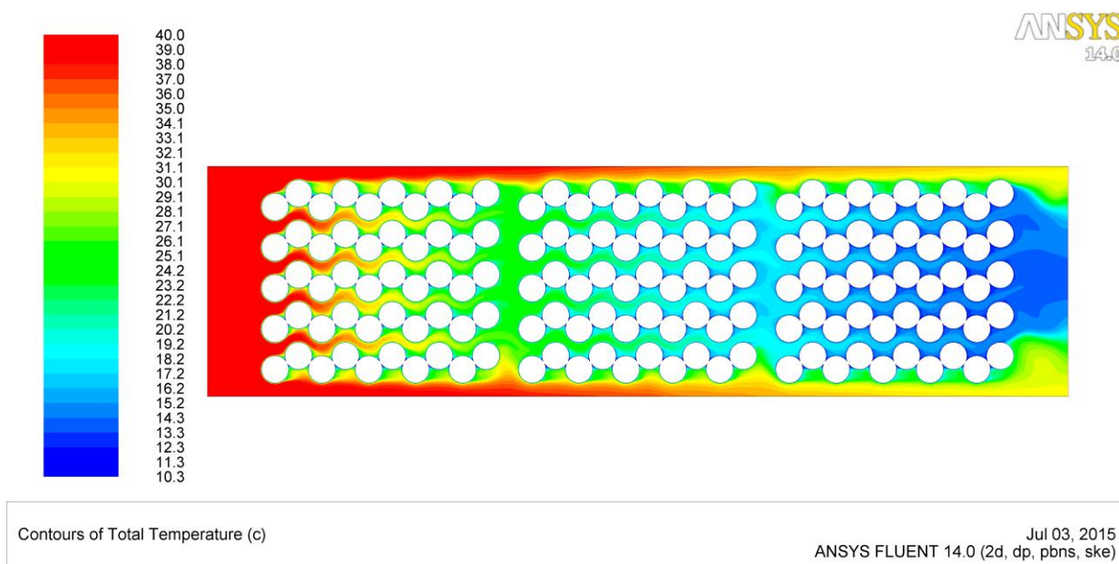
Рис. 3.23. Зміна температури в каналі, °C
