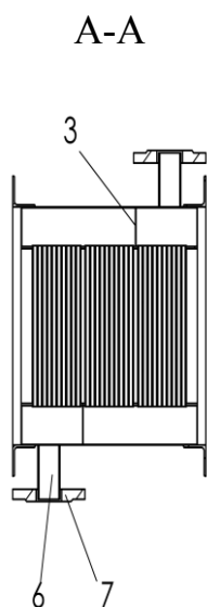
Рис. 4.7. Розріз кожухотрубного теплообмінника в перерізі А-А
