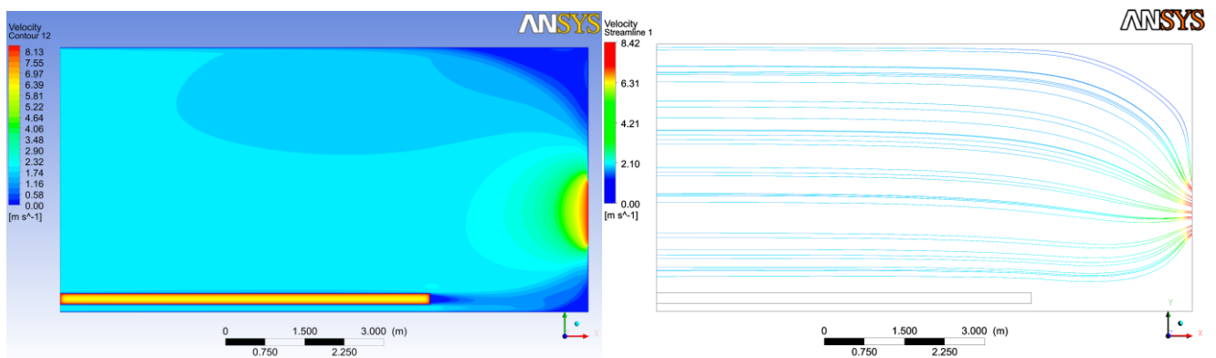
Рис. 2.23. Поле швидкості та лінії току повітря в поздовжньому перерізі будівлі по середній лінії на осі Ox
