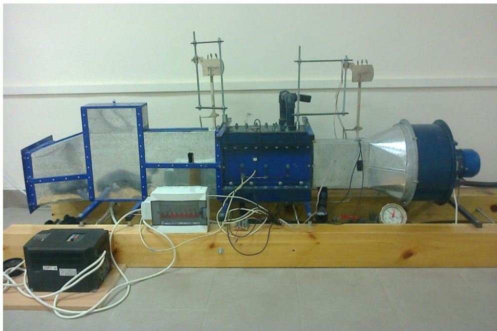
Рис. 4.1. Загальний вигляд модернізованого електротехнічного комплексу для підтримання нормованого мікроклімату пташника
