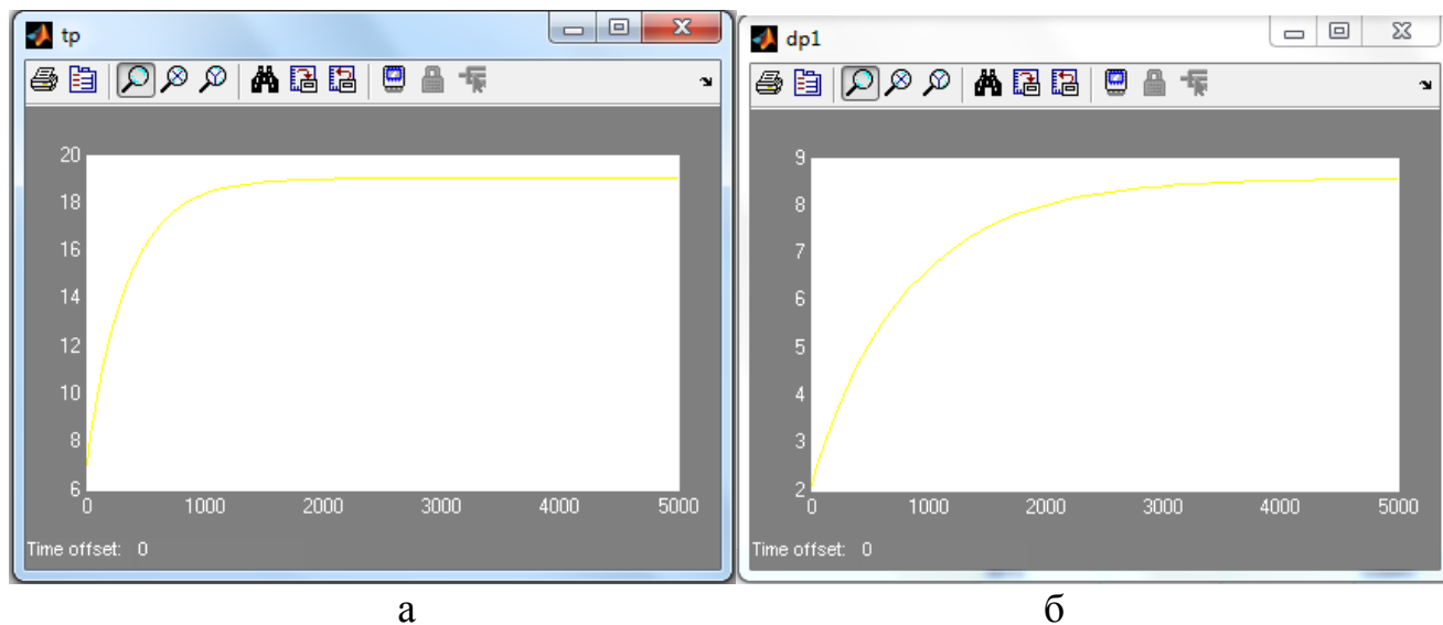
Рис. 2.34. Розгінна крива зміни температури (а) і вологовмісту (б) в приміщенні пташника в зимовий період року, яка отримана по даних моделі MATLAB Simulink
