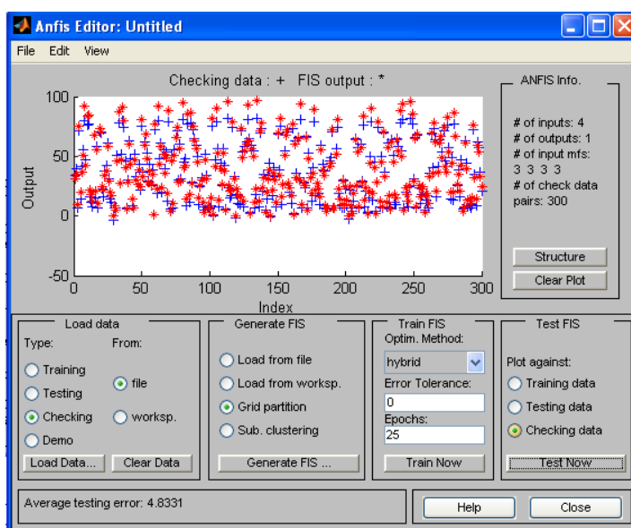
Рис. 4.20. Результати само налаштування ANFIS на перевіряльні дані
