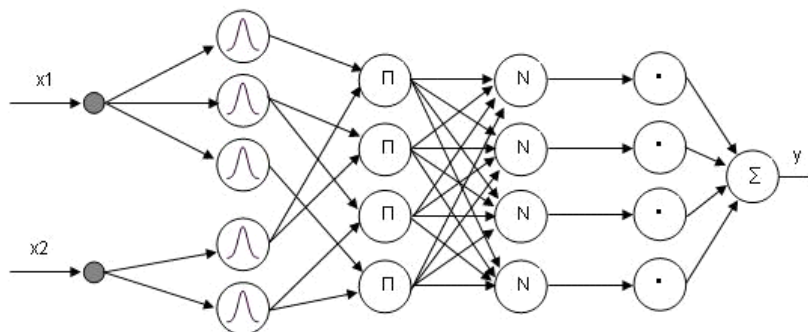
Рис. 4.14. ANFIS мережа
