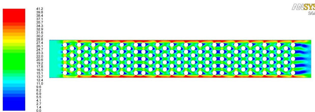
Рис. 3.3. Швидкість повітря в каналі шахового пучка, м/с
