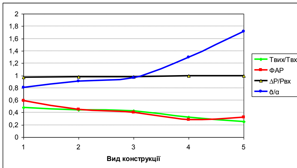
Рис. 3.19. Фактор аналогії Рейнольдса та безрозмірні значення вихідної температури, втрат тиску і коефіцієнта теплообміну на поверхні каналів різної геометрії з компактним розміщенням труб
