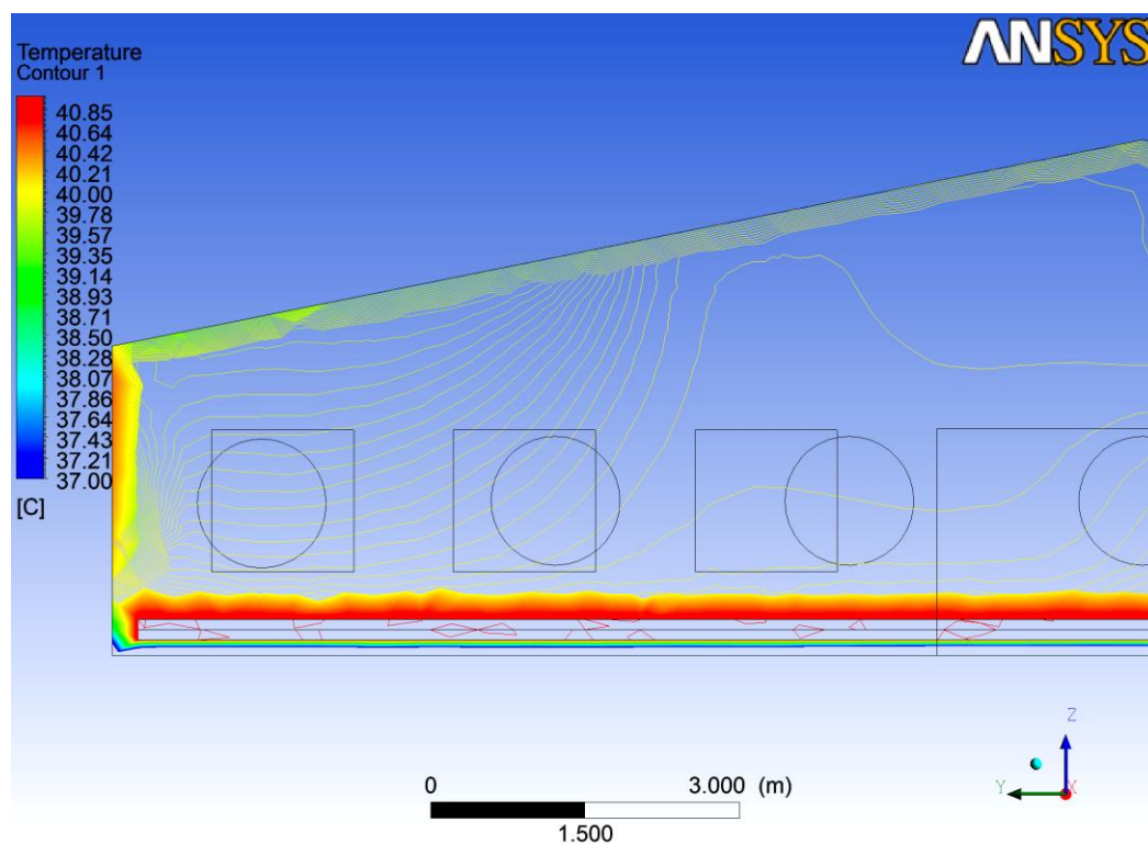
Рис. Г.4. Контурне поле температур в поперечному перерізі будівлі по осі Oy на відстані 30 м від входу в інтервалі від 37 до 41, °C
