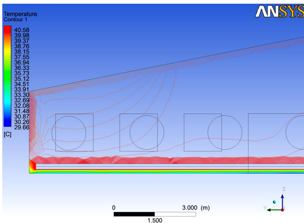
Рис. Г.3. Контурне поле температур в поперечному перерізі будівлі по осі Oy на відстані 30 м від входу в інтервалі від 30 до 41, °C
