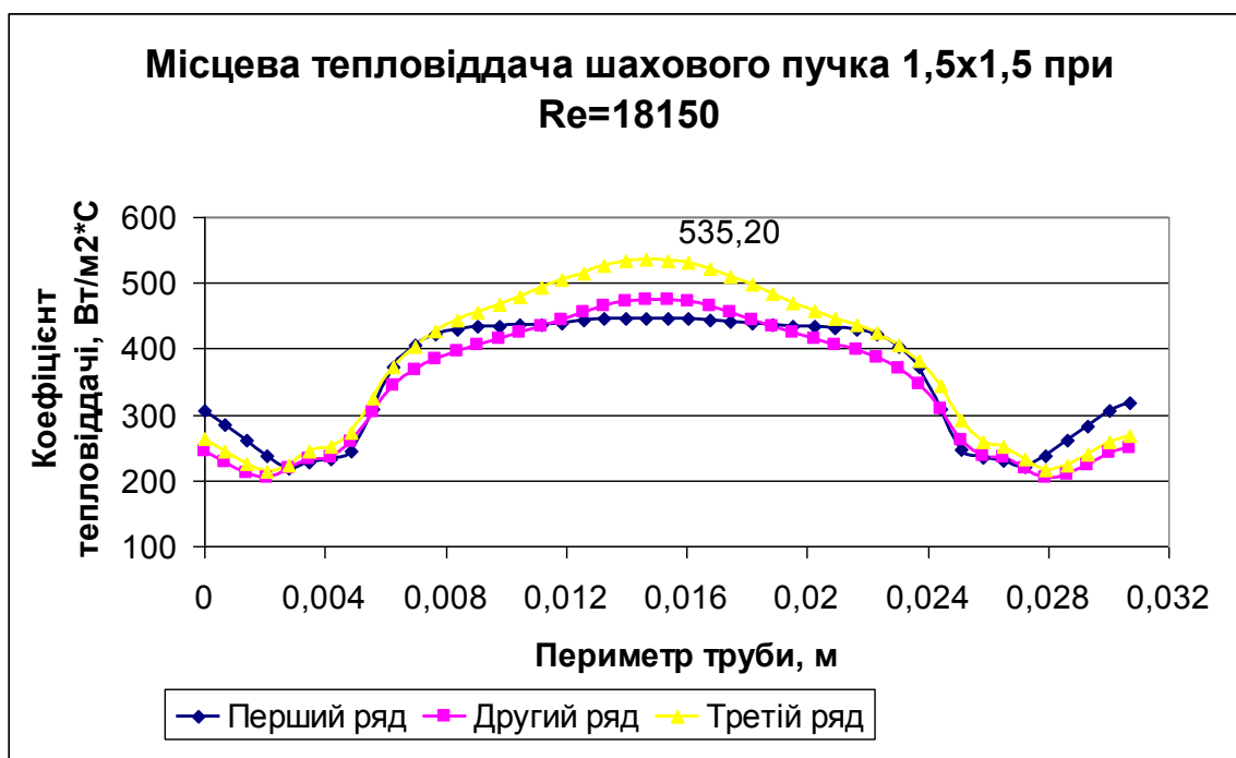
Рис. 3.8. Місцева тепловіддача шахового пучка 1,5x1,5 при Re=18150
