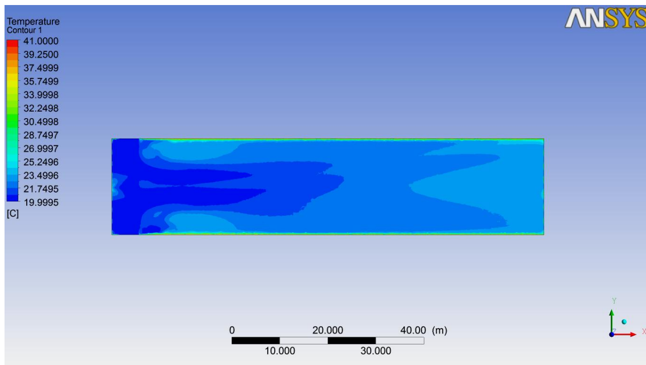
Рис. 2.18. Температурне поле в приміщенні пташника в поперечному перерізі будівлі по осі Oz на висоті 1,5\text{ м} від підлоги, ^{\circ}\text{C}
