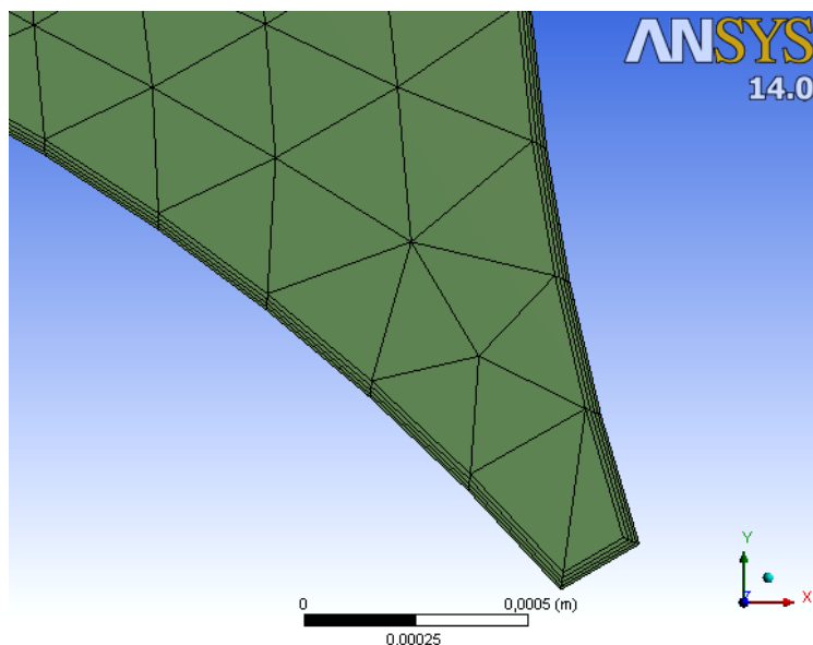
Рис. В.5. Гібридна сітка з методом межового шару 3Т при наявності 4 шарів з початковою товщиною шару 3 \cdot 10^{-5}
