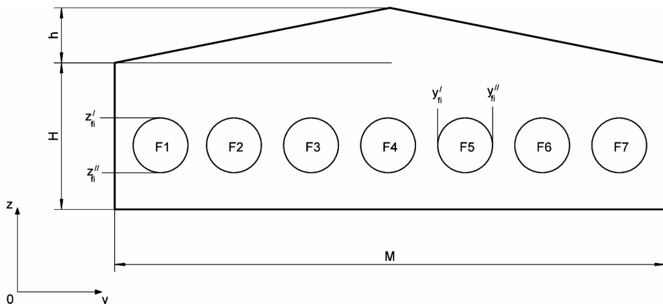
Рис. 2.10. Задня торцева стінка пташника
