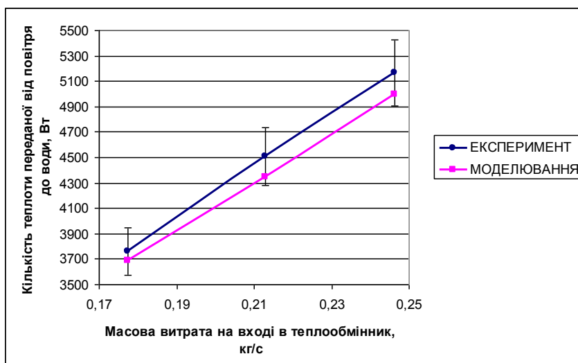
Рис. 4.10. Залежність кількості переданої теплоти від масової витрати на вході в теплообмінник
