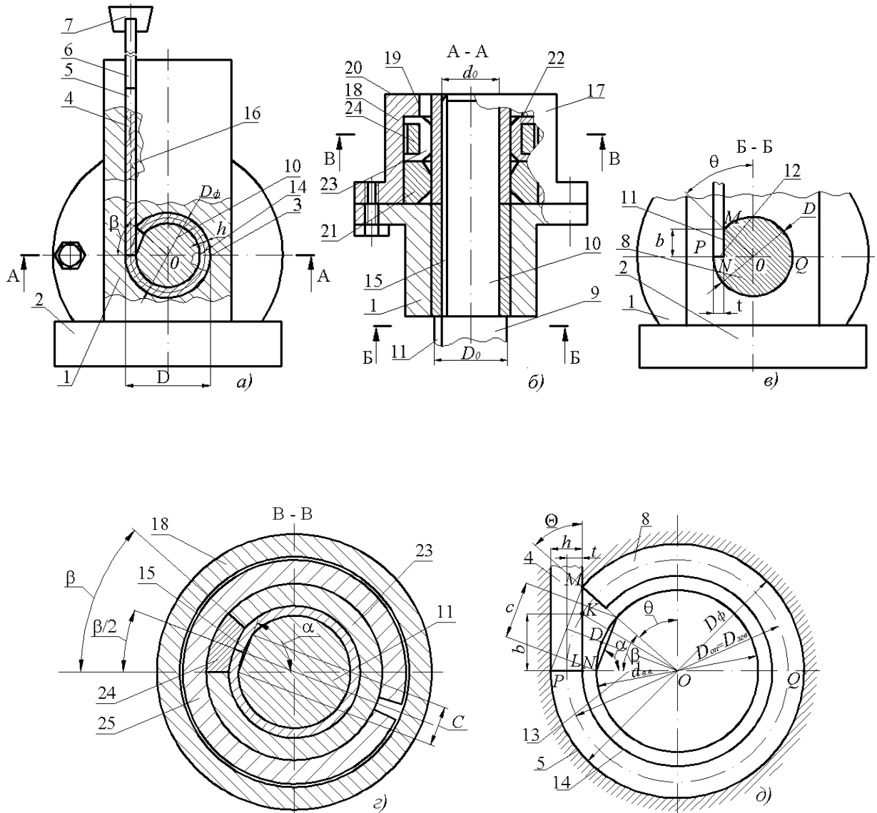
Рисунок 3.19 Пристрій для формування і калібрування згортних втулок: a – головний вигляд; б – переріз А-А; в – переріз Б-Б; г – переріз В-В; д – розрахункова схема
