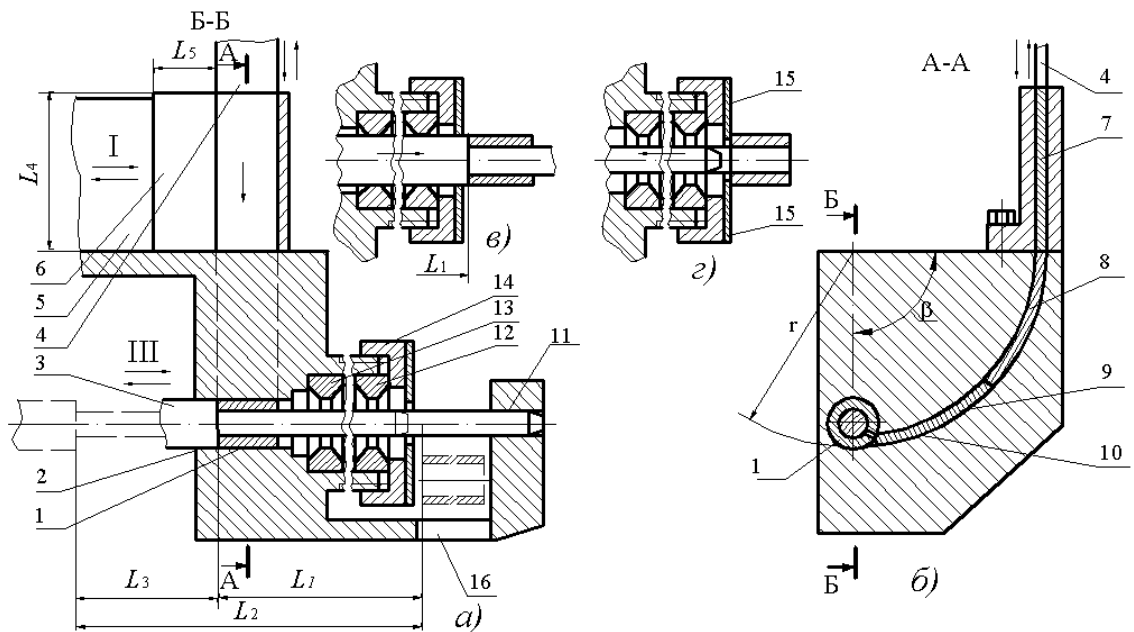
Рисунок 2.9 Пристрій для формування згортної втулки із карточки за запропонованою технологією: a – головний вигляд; б – переріз А-А; в – г – фрагментарні зображення оправки відповідно у правому і лівому крайніх положеннях
