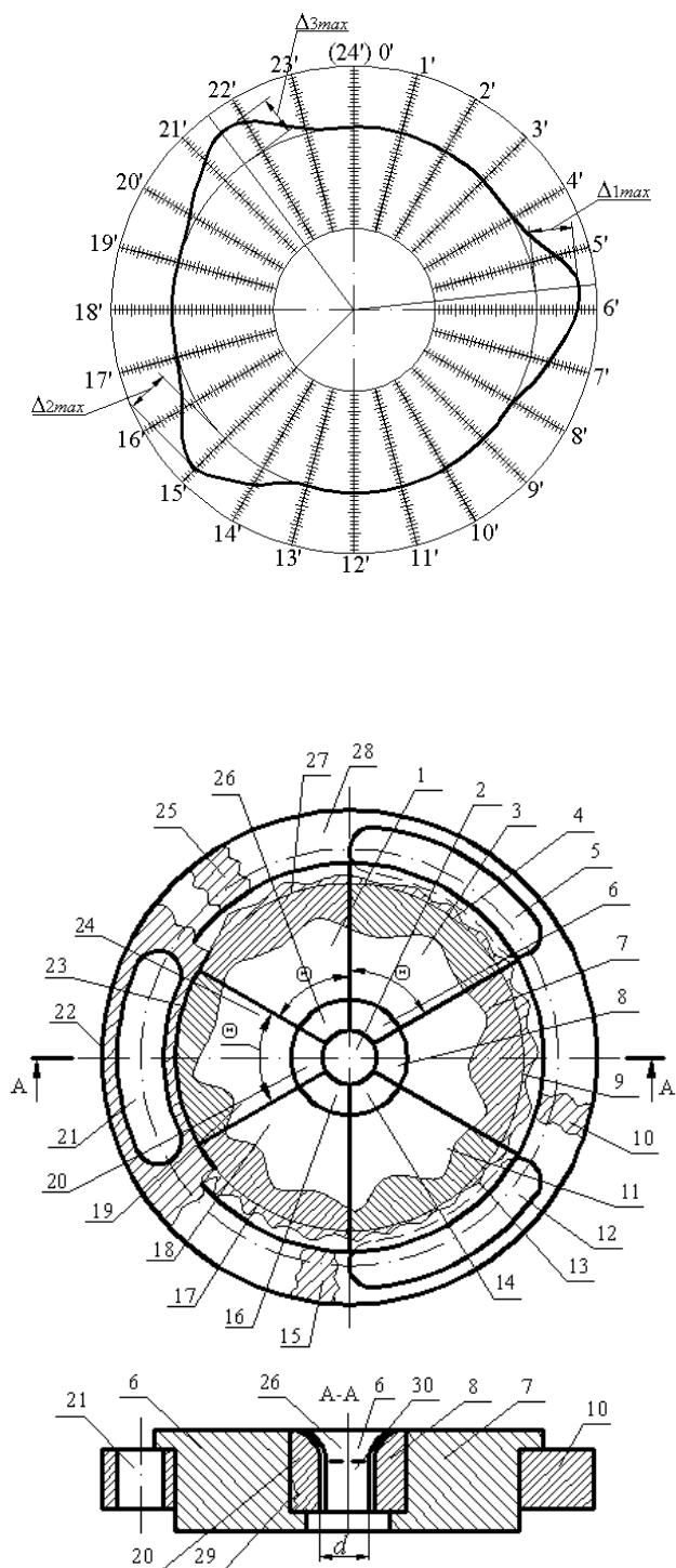
Рисунок 3.26 Запропонована нова розрізна пружня 2n-секторна фільєра – а), круглограма відхилень згортних втулок – б)
