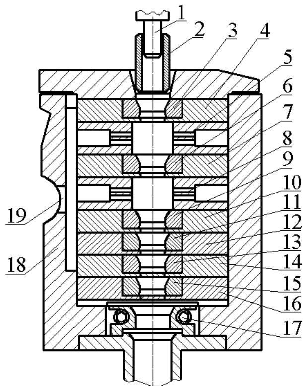
Рисунок 1.9 Пристрій для калібрування згортних втулок заводу «Краснодарсільмаш»
