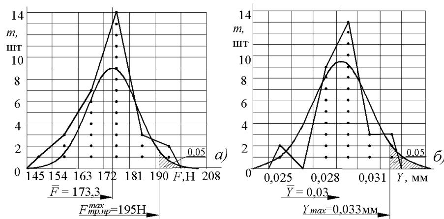
Рисунок 2.19 Полігони і теоретичні криві розсіювання: а) – приведеної сили тертя F_{mp,np} ; б) – приведеної величини відпружинення Y
