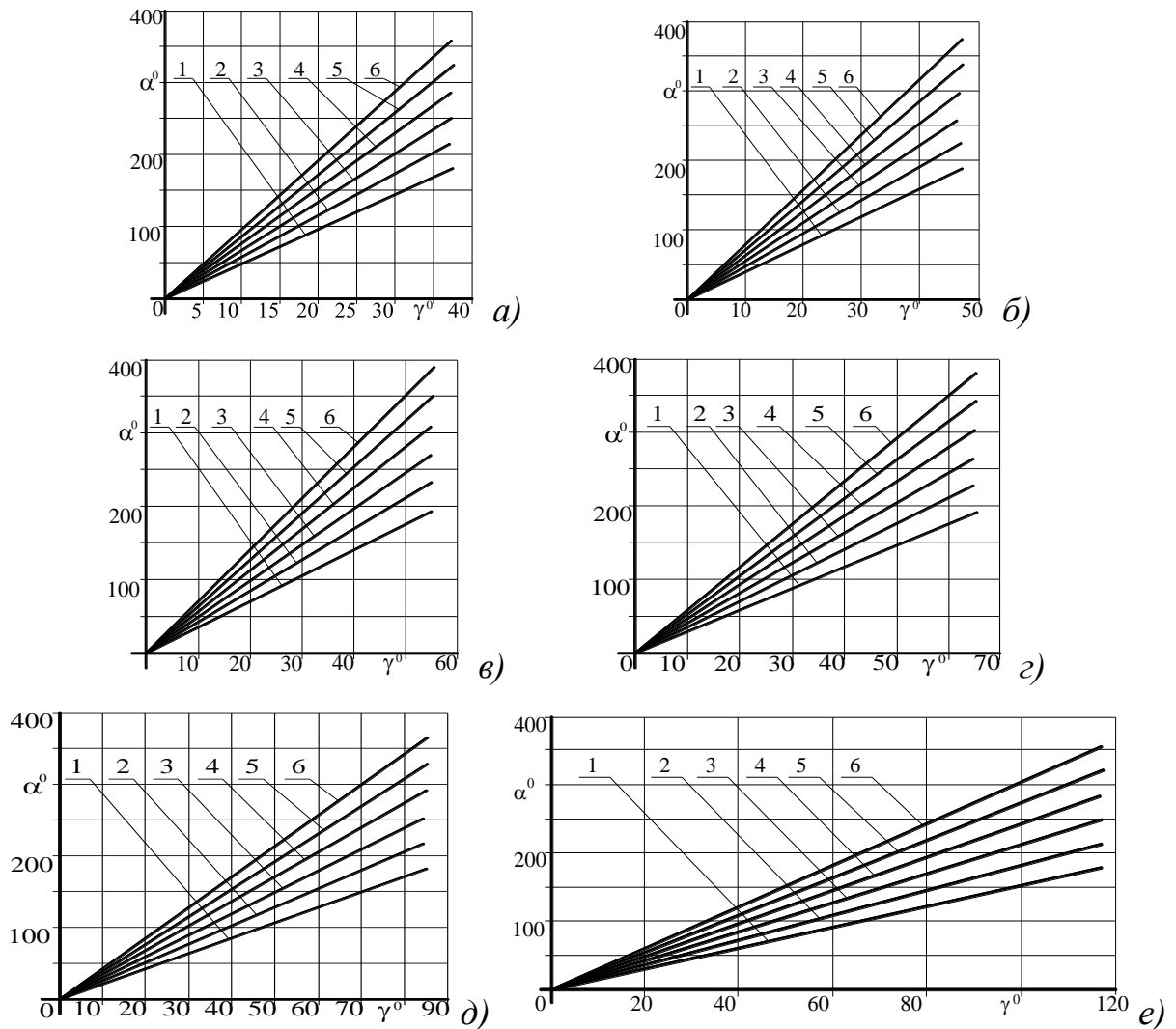
Рисунок 4.6 Графіки залежності кута \alpha повороту згортної карточки у ФМ від кута \gamma повороту кругової шкали для:
