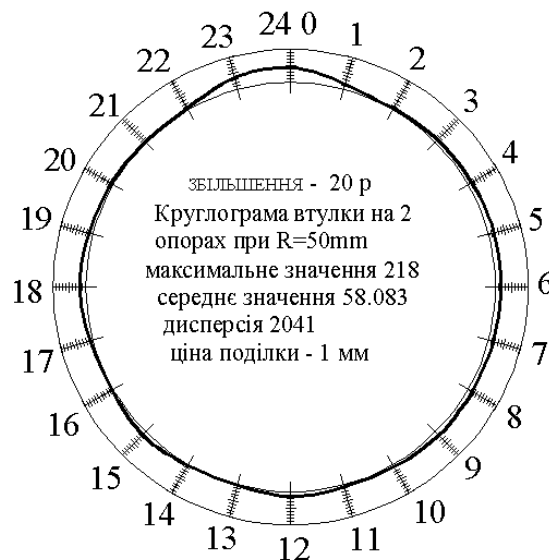
Рисунок 4.10 Усереднена круглограма згортної втулки сформованої при радіусі транспортного каналу R=50 мм і способі базування ФМ – оправка на 2-х опорах
