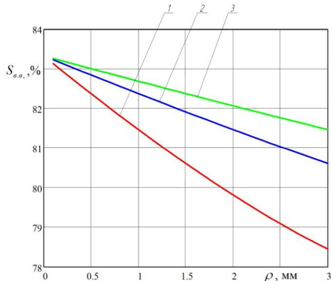
Рисунок 2.23 Графік залежності відносної площі віброобкочування регулярного мікрорельєфу S_{в.в.} у % від ширини канавки \rho в мм при відповідних значеннях ширини стрічки: 1 – H=10 мм, 2 – H=20 мм, 3 – H=30 мм.
