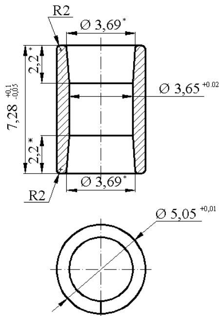
Рисунок 1.3 Корсетна згортна втулка для дворядного приводного втулкового ланцюга з кроком 9,525 мм приводу механізму газорозподілу і помпи системи мащення двигуна внутрішнього згоряння заводу DITTON (Латвія)
