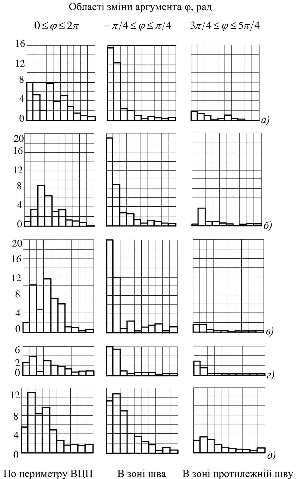
Рисунок 4.12 Експериментальні лінійчасті спектри амплітуд відхилень від круглості ВЦП втулок для приводних ланцюгів з кроками відповідно:
