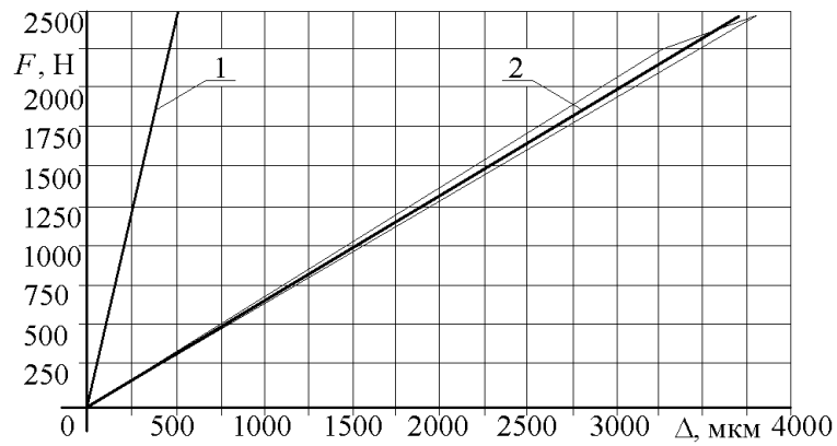
Рисунок 4.3 Тарувальні графіки: 1 і 2 – відповідно для динамометрів зразкового (ДОР-3) і досліджуваного (ДОР-0,5)
