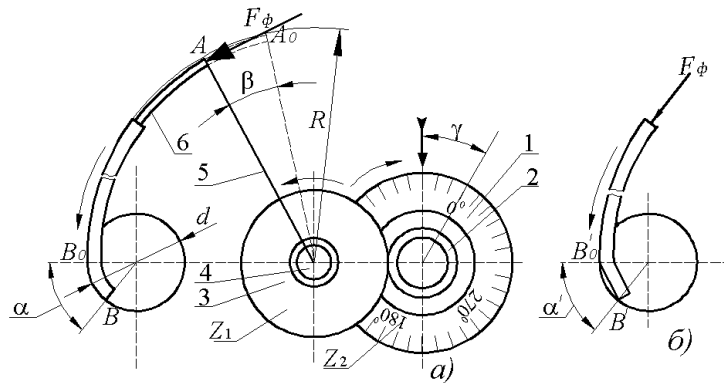
Рисунок 4.4 Варіанти технологічної операції формування згортної втулки з різними способами базування заготовки: a – без оправки; б – на консольно закріпленій оправці; в – на оправці, закріпленій на двох опорах
