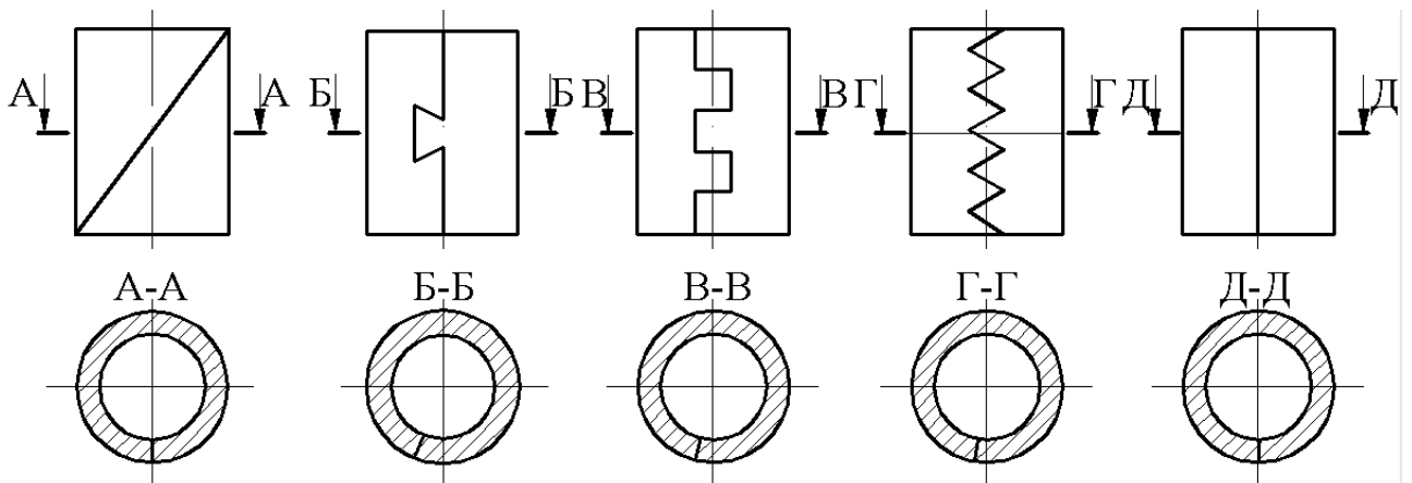
Рисунок 1.2 Деякі види стикових швів згортних втулок
