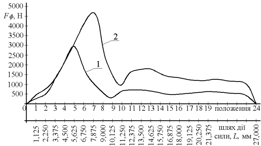
Рисунок 5.1 Графіки зміни сили формування втулки F_{\phi} в процесі її згортання:
