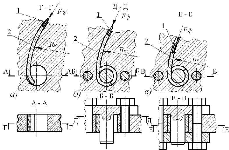
Рисунок 4.4 Варіанти технологічної операції формування згортної втулки з різними способами базування заготовки: a – без оправки; б – на консольно закріпленій оправці; в – на оправці, закріпленій на двох опорах
