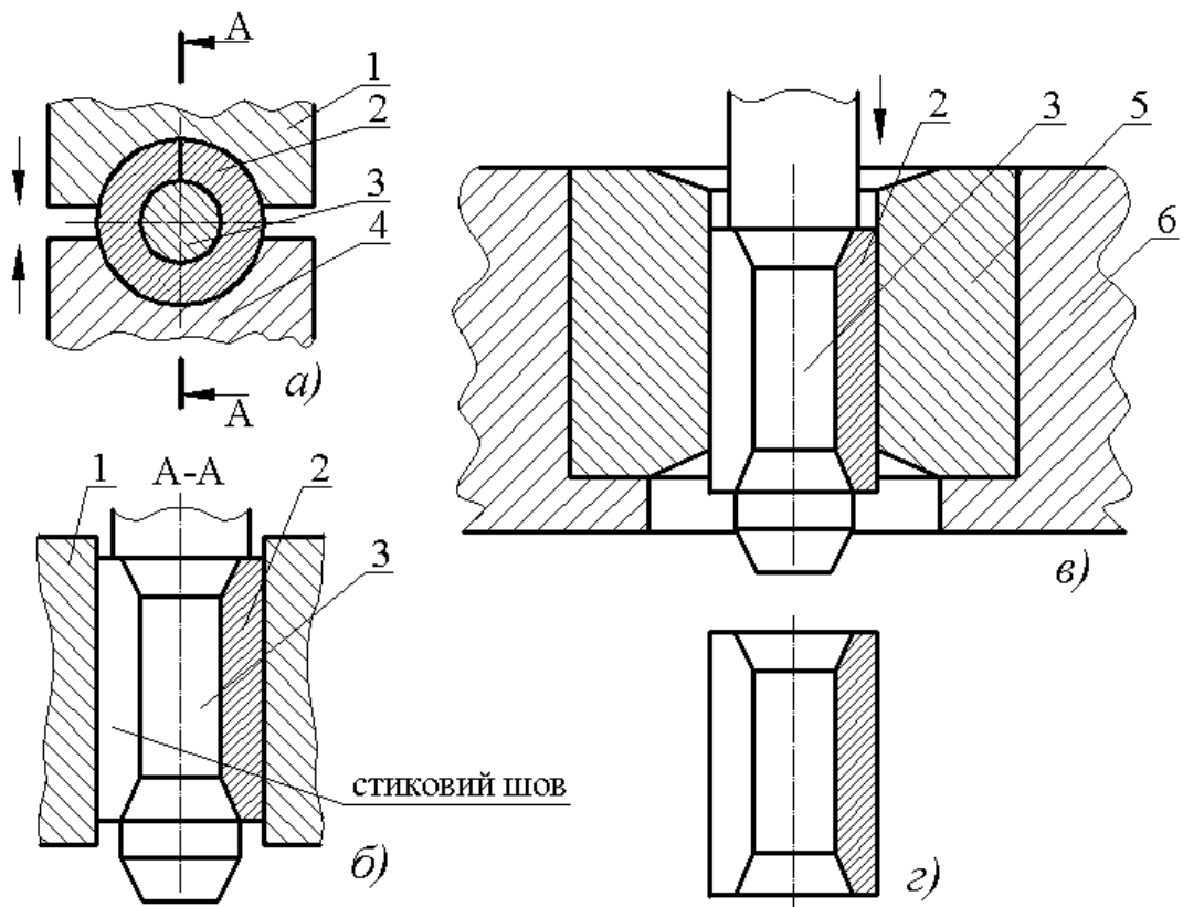
Рисунок 1.7 Схеми останніх переходів формування згортої втулки втулкового приводного дворядного ланцюга з кроком 9,525 мм.: a – положення на оправці 3 згортої втулки 2 у закритих верхній 1 і нижній 4 напівматрицях; б – переріз А-А рис.1.7, a ; в – схема процесу калібрування згортої втулки 2, розміщеної на оправці 3 у калібруючій фільтері 5, встановленій у отворі плити 6; г – сформована корсетна втулка
