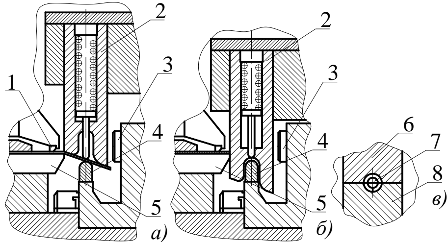
Рисунок 1.8 Послідовність формування згортних втулок за технологічним процесом на заводі «Краснодарсільмаш»
