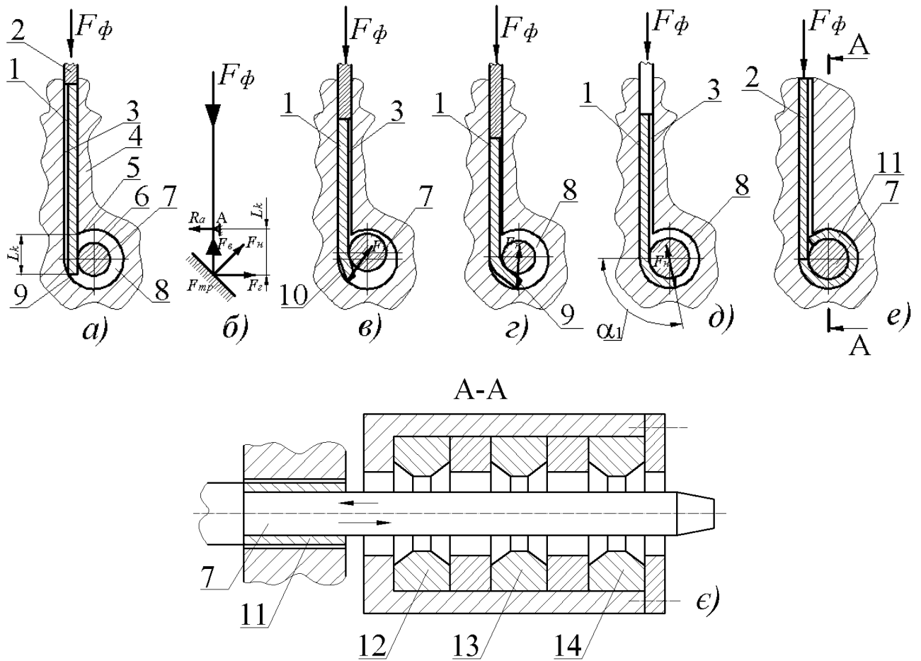
Рисунок 1.10 Схематичне зображення фрагментів технологічного процесу формування циліндричної поверхні згортної втулки, реалізованого на НЗНА
