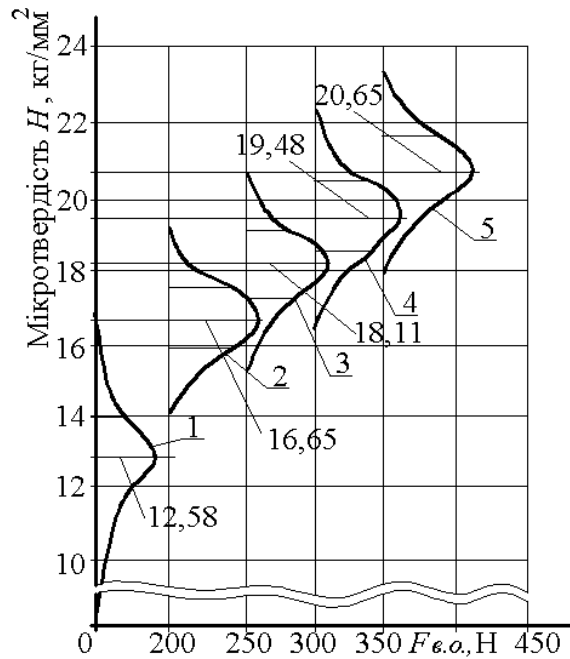
Рисунок 4.17 Теоретичні криві Гауса розподілу параметра мікротвердості при різних значеннях зусилля обкочування F_{во}
