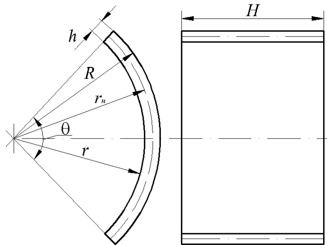
Рисунок 3.1 Схематичне зображення заготовки згортої втулки у вигляді частково-циліндричної оболонки: h – товщина стінки згортої втулки, R і r – відповідно радіуси зовнішньої та внутрішньої поверхонь заготовки, H – її висота
