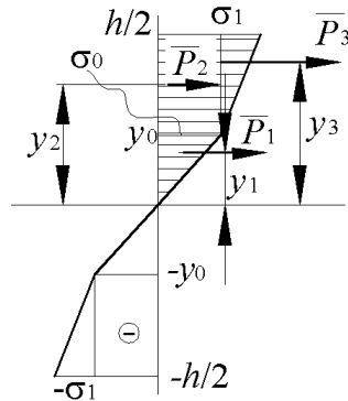
Рисунок 2.4 Діаграма розподілу напружень за товщиною h стінки згортної втулки
