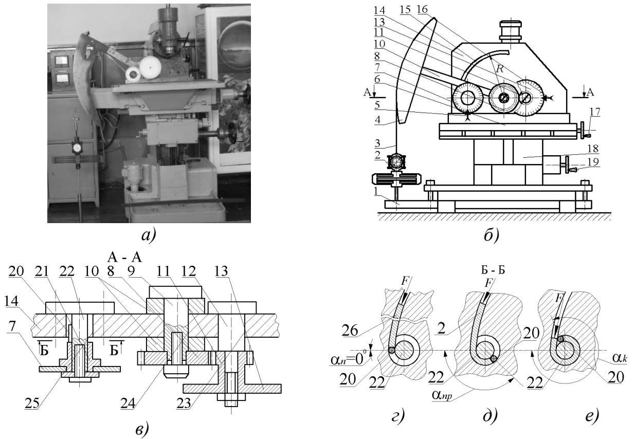
Рисунок 4.1 Експериментальна установка: а) – загальний вигляд; б) – конструктивна схема; в) – переріз по А-А; г) –, д) –, е) – переріз по Б-Б, положення картки у формуючій фільтрі, які визначаються відповідними кутами закручування: \alpha_n = 0^\circ ; 0^\circ \leq \alpha_{np} \leq 270^\circ і \alpha_k > 270^\circ
