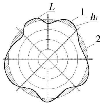
Рисунок 1.15 Схематичне зображення круглограми для визначення середнього арифметичного відхилення від круглості EFK_d : 1 – реальний профіль; 2 – середнє коло
