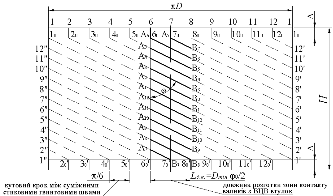
Рисунок 3.8 Схематичне зображення слідів розгортки рівномірно розміщених по колу стикових швів 12-ти згортних втулок
