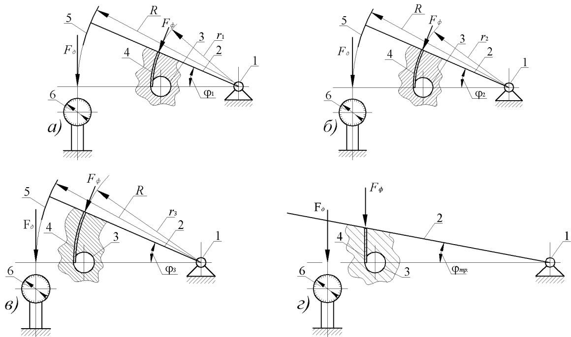
Рисунок 4.8 Розрахункові схеми для визначення зусилля формування F_\phi згортних втулок при R=500 мм., та різних радіусах транспортного каналу: а) – r_1=50 мм., б) – r_2=75 мм., в) – r_3=100 мм., г) – прямолінійний транспортний канал. 1 – шарнір, 2 – важіль, 3 – формуюча матриця, 4 – транспортний канал, 5 – обичайка з R=const , 6 – динамометр
