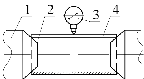
Рисунок 1.20 Схема вимірювання відхилень від круглості зовнішньої циліндричної поверхні згортних втулок в центрах: 1 і 5 – відповідно передній і задній центри; 2 – згортна втулка; 3 – індикатор; 4 – стиковий шов
