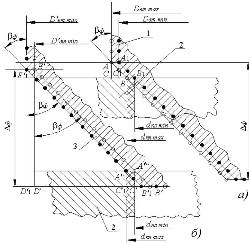
Рисунок 3.11 Розрахункова схема для визначення значень діаметрів зовнішньої циліндричної поверхні згортних втулок з розкритим стиковим швом: a і б – відповідно положення згортних втулок із закритим і відкритим стиковими швами перед їх запресуванням у отвори внутрішніх пластин; 1 і 2 – відповідно згортні втулки із закритим і розкритим стиковими швами; 3 – внутрішня пластина
