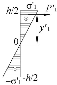
Рисунок 2.5 Епюра напружень в кожному перерізі балки
