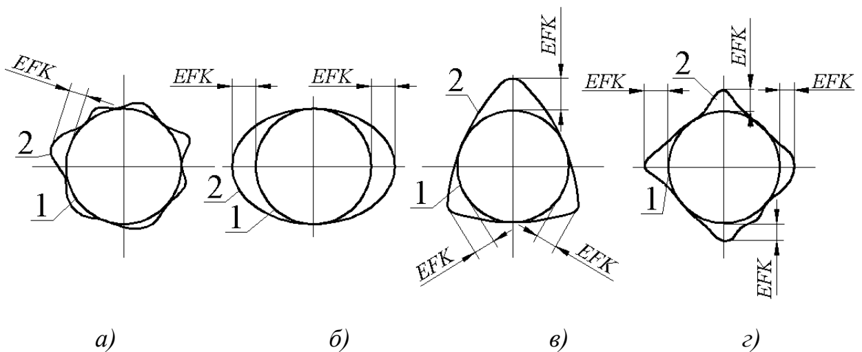
Рисунок 1.17 Схематичне зображення форми поперечних перерізів циліндричних поверхонь з однаковою величиною відхилень від круглості: 1 – круглограма; 2 – прилягаюче коло; a , б , в , г – різні форми відхилень від круглості
