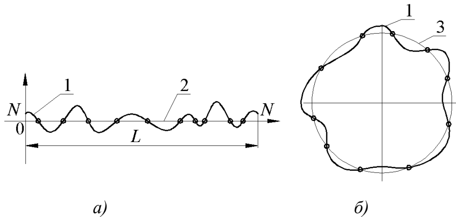
Рисунок 1.16 Схематичне зображення кількості точок перетину реального профілю із середнім профілем: a – для поздовжнього перерізу; б – для круглості: 1 – реальний профіль; 2 – середня пряма; 3 – серединне коло
