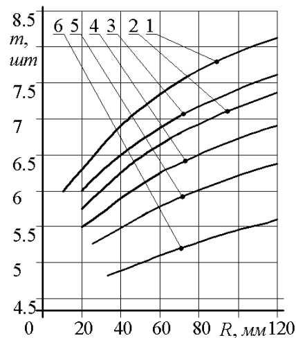
Рисунок 2.16 Графік залежності t = \psi(r) для втулок різних карточок;
