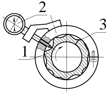
Рисунок 1.18 Схема вимірювання відхилень від круглості зовнішньої циліндричної поверхні згортних втулок з використанням спеціального кільця: 1 – досліджувана згортна втулка; 2 – індикатор; 3 - кільце
