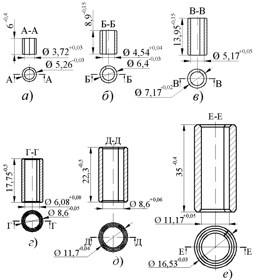
Рисунок 1.1 Згорні втулки для ПРВЛ різних виробників:
