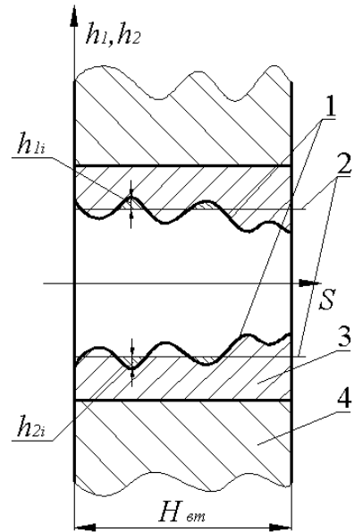
Рисунок 1.14 Схематичне зображення відхилення профілю поздовжнього перерізу: 1 – реальний профіль; 2 – середній профіль; 3 – втулка; 4 – корпус
