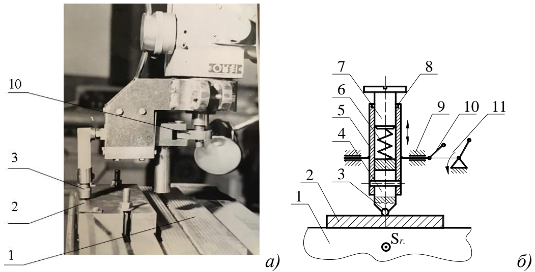
Рисунок 4.14 Загальний вигляд – а) і кінематична схема – б) пристрою для вібраційного обкочування плоских поверхонь змонтованого на пінолі широкоуніверсального верстата мод. 6А75В
