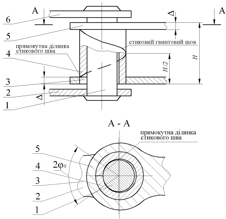
Рисунок 3.7 Фрагмент ПРВЛ із запропонованою втулкою: 1 – валик; 2, 6 – зовнішні пластини; 3, 5 – внутрішні пластини; 4 – згортна втулка
