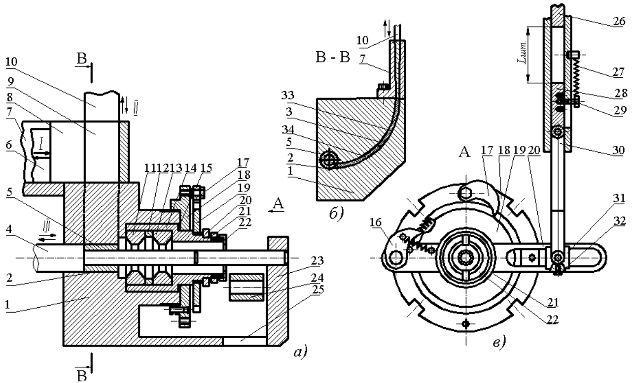
Рисунок 3.14 Пристрій для формування і калібрування згортих втулок з храповим механізмом повороту фільєр
