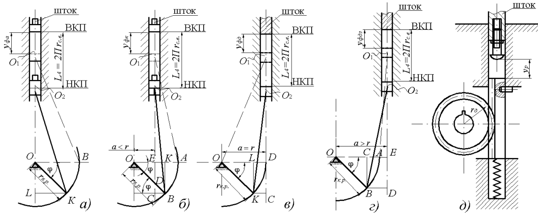
Рисунок 3.16 Розрахункові схеми для визначення налагоджуваного розміру у:
