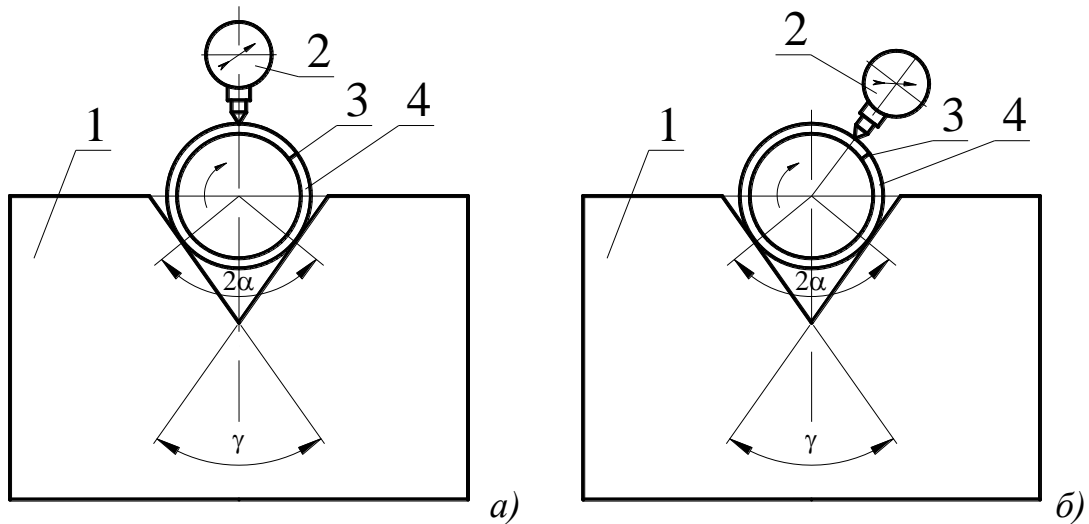
Рисунок 1.19 – Схеми вимірювання відхилення від круглості – огранювання в призмі: а – симетрична; б – несиметрична; 1 – призма; 2 – індикатор годинникового типу; 3 – згортний шов; 4 – досліджувана згортна втулка
